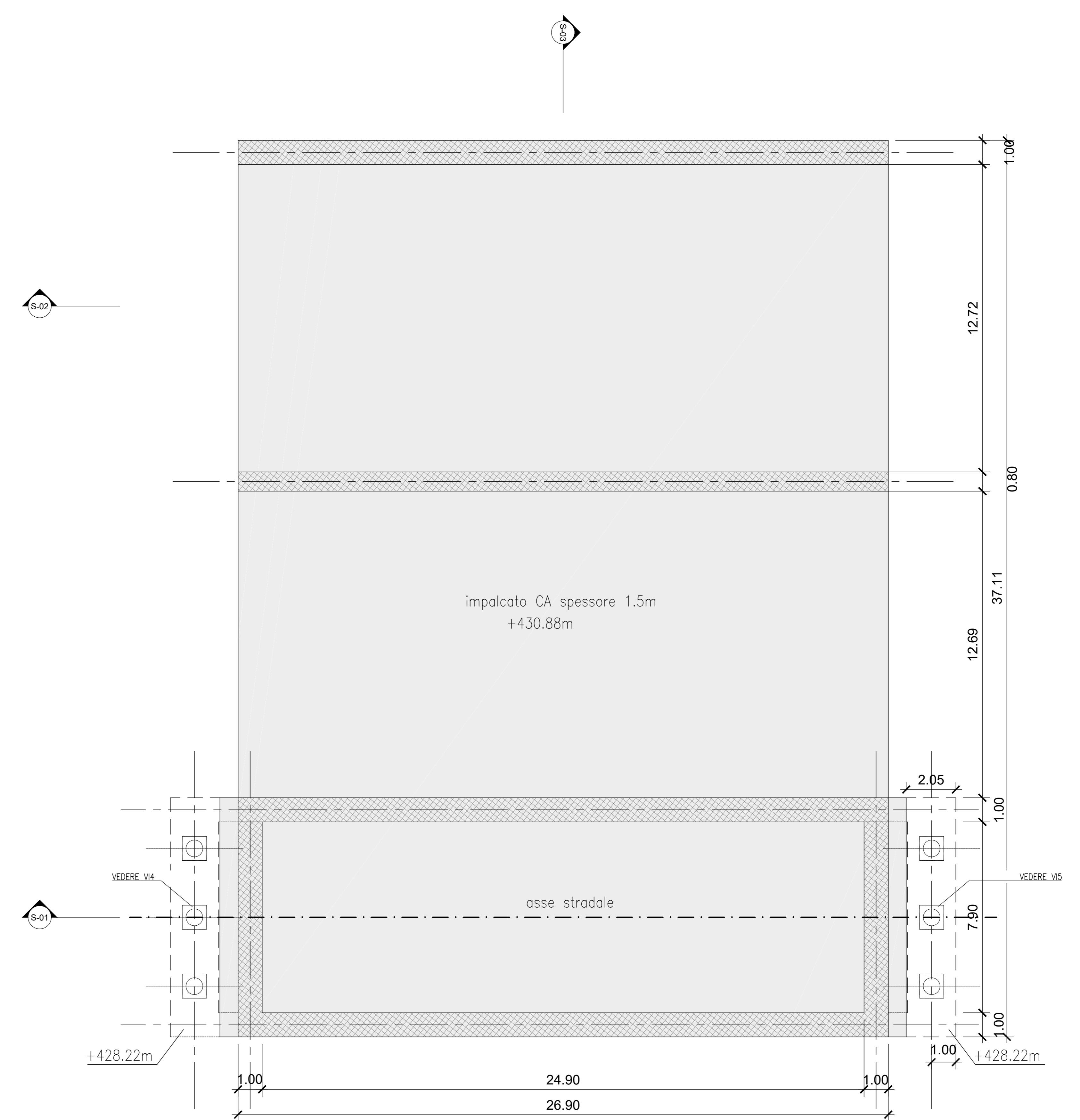
PIANTA IMPALCATO - Scala 1:100
