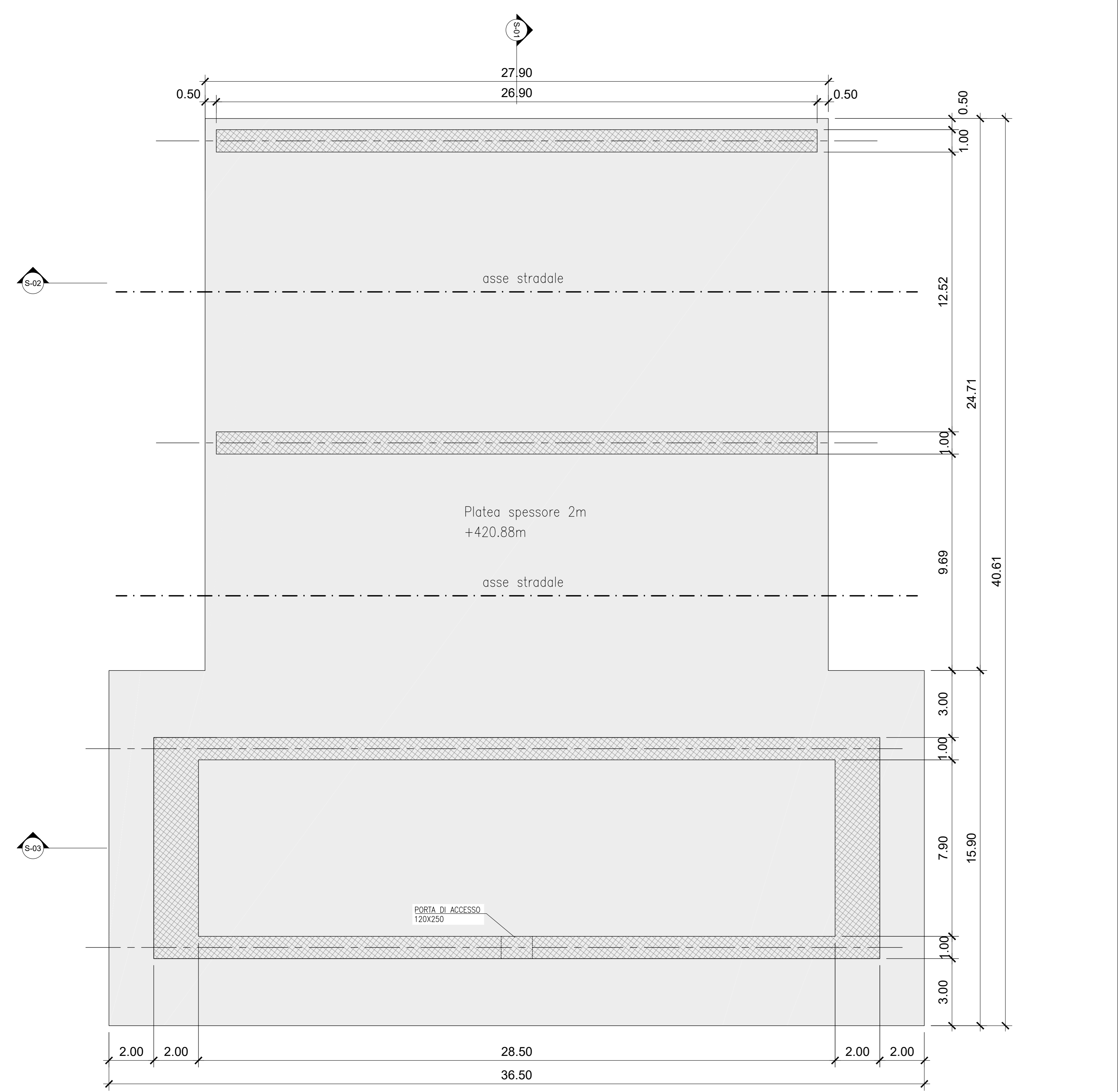
PIANTA FONDAZIONI - Scala 1:100
