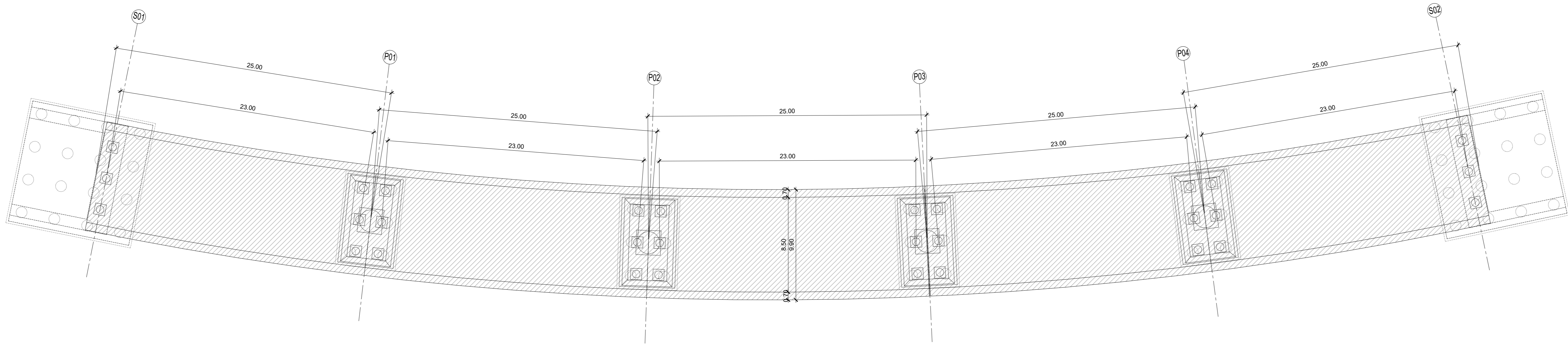
PIANTA IMPALCATO - Scala 1:200
