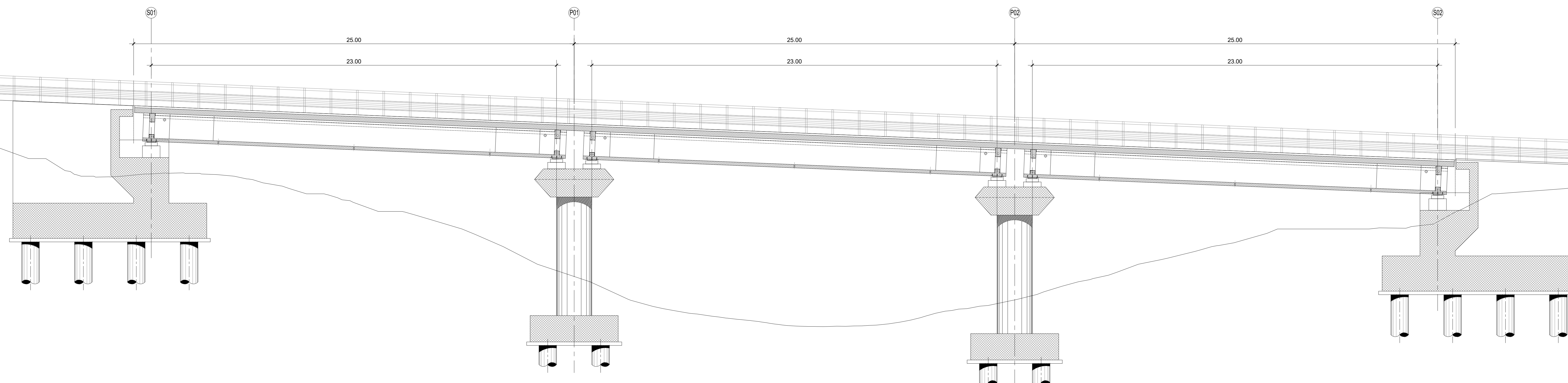
SEZIONE LONGITUDINALE - Scala 1:100
