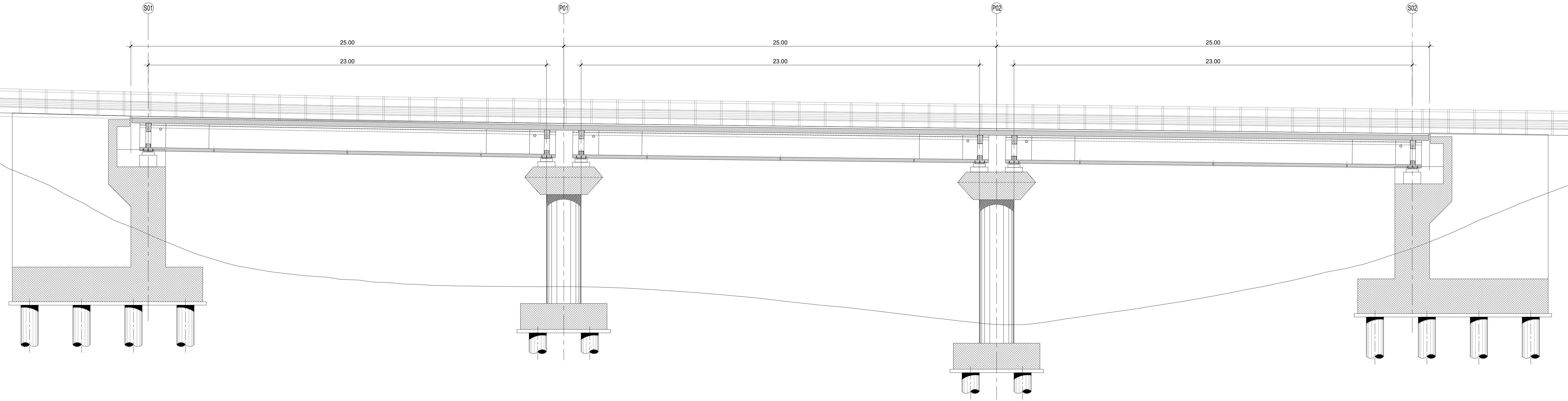
SEZIONE LONGITUDINALE - Scala 1:100
