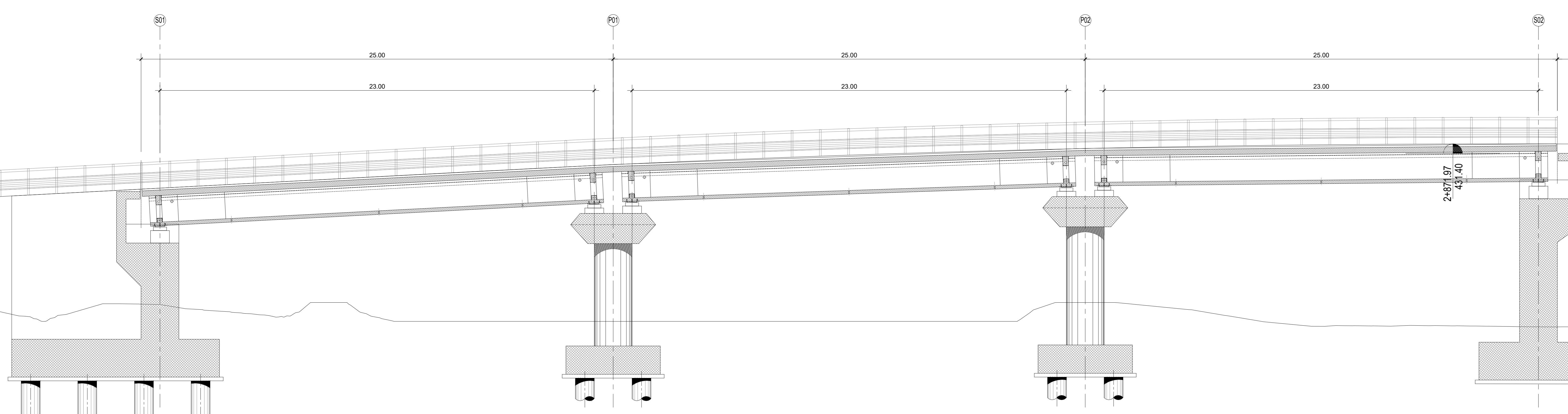
SEZIONE LONGITUDINALE - Scala 1:100
