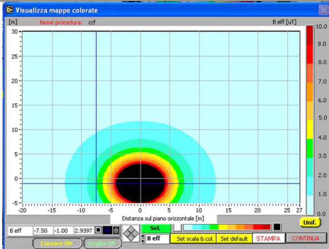
SINGOLA TERNA DI CAVI POSATI A TRIFOGLIO: DPA = 7.5 m
