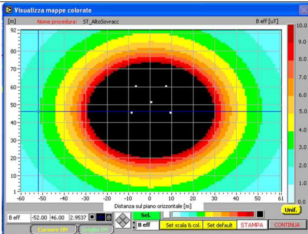
SOSTEGNO A TRALICCIO SINGOLA TERNA 380 kV ALTO SOVRACCARICO TIPO G1
