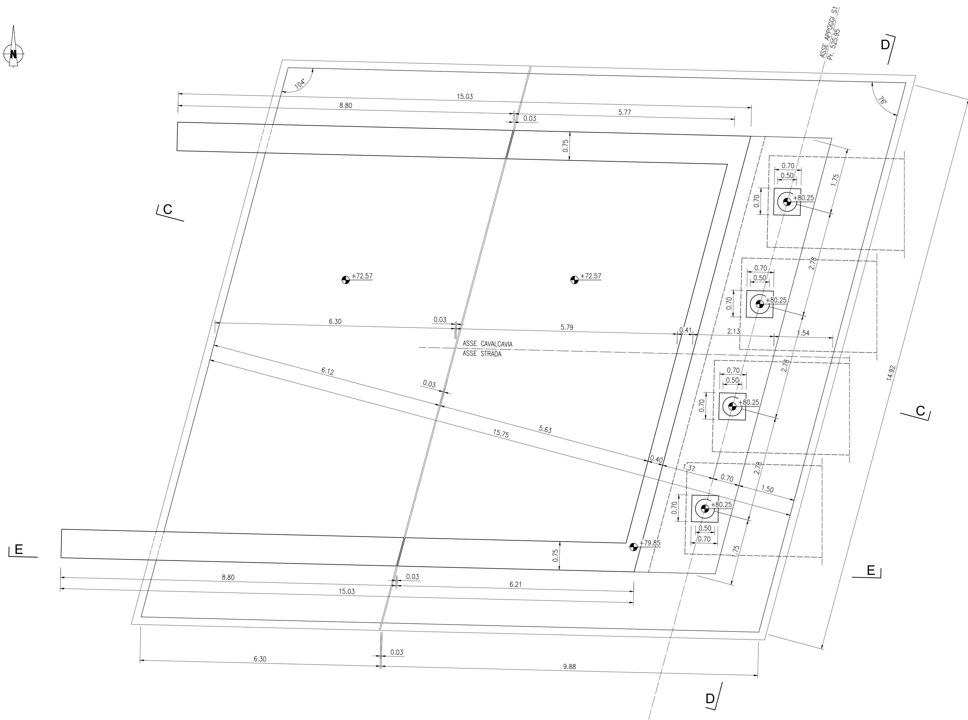
VISTA DALL'ALTO (1:50)
