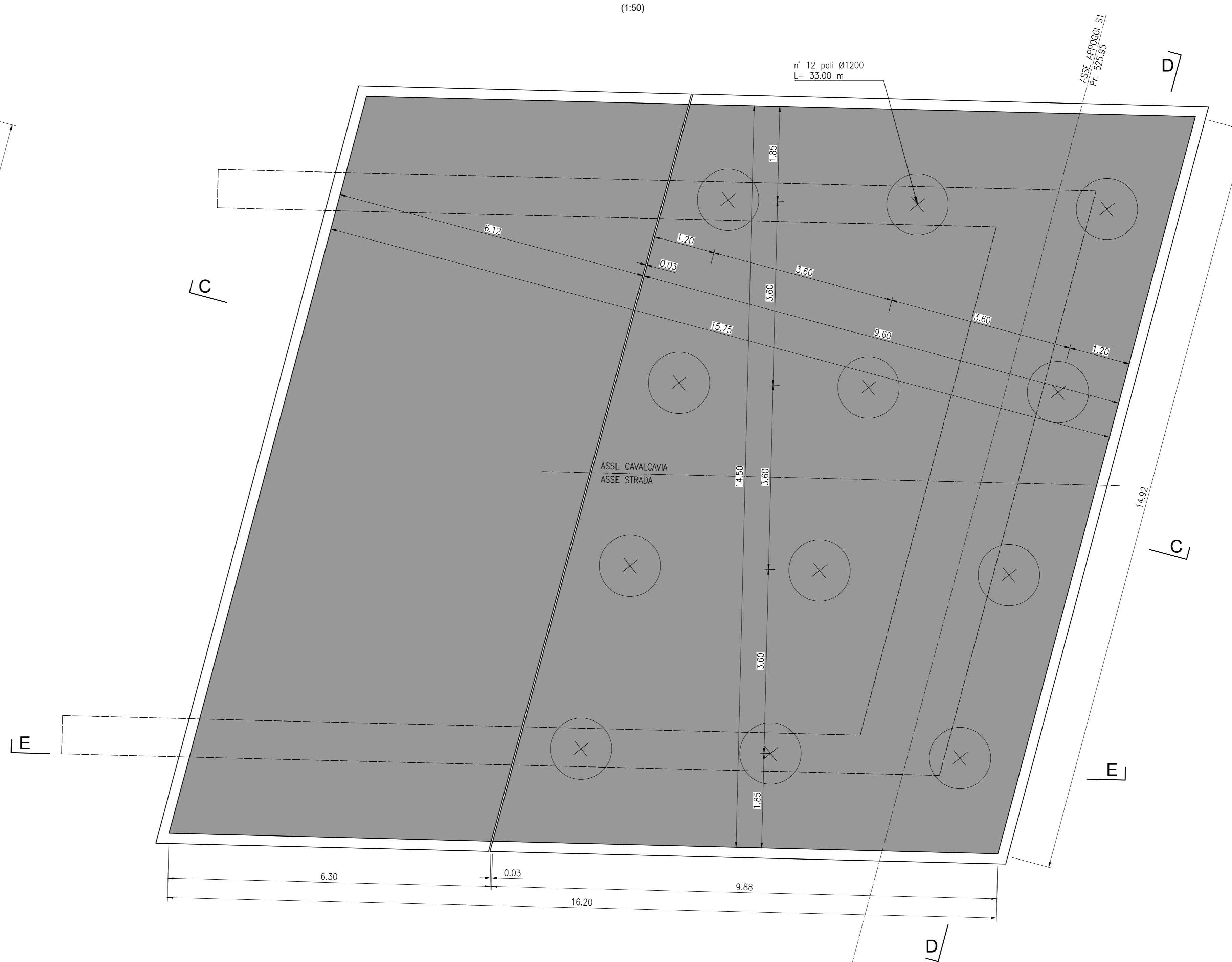
SEZIONE B-B (1:50)
