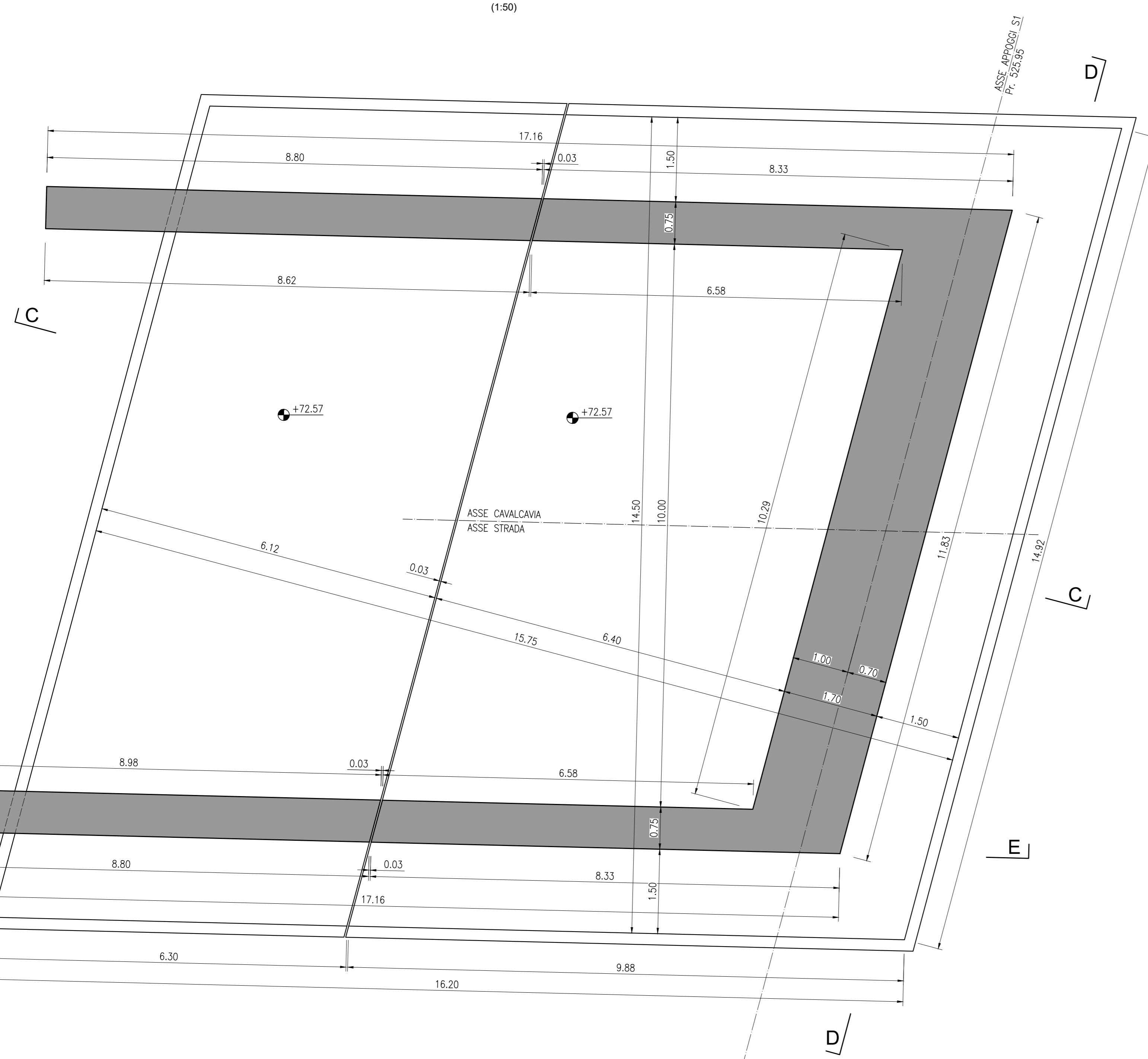
SEZIONE A-A (1:50)
