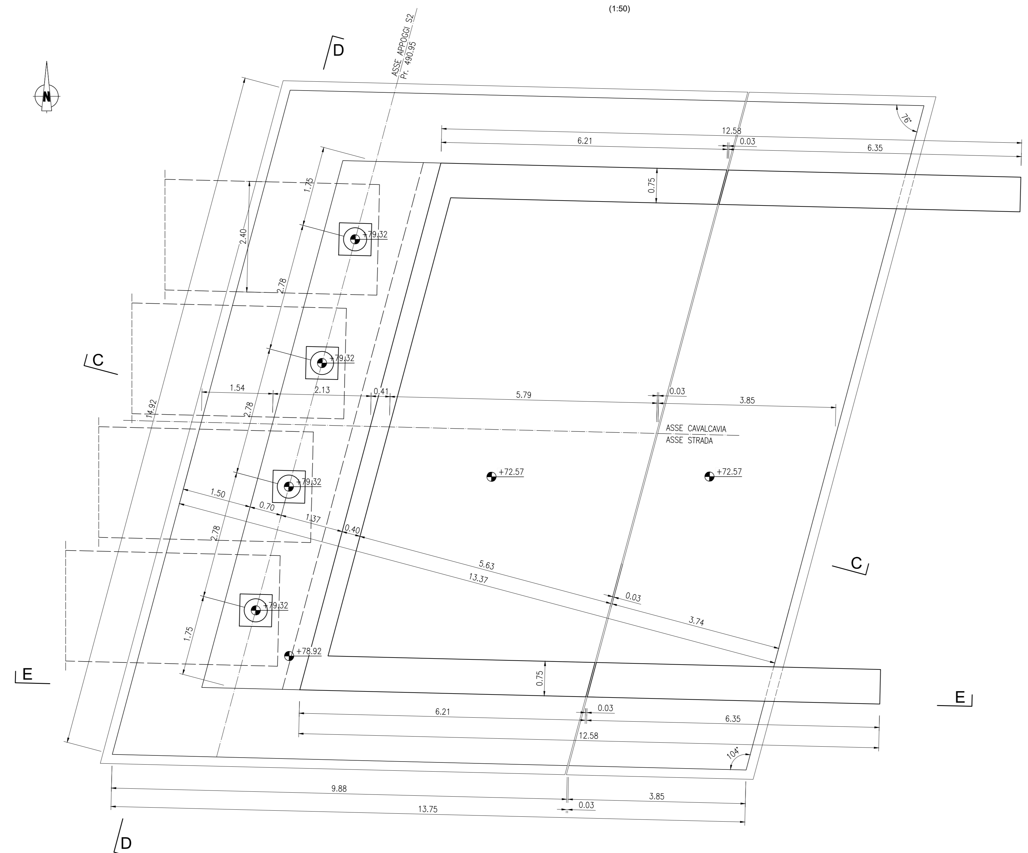
VISTA DALL'ALTO (1:50)
