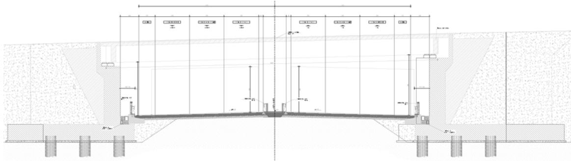
Figura 3: Sezione tipo in corrispondenza cavalcavia
