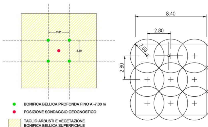
Figura 7 – Dettagli progettazione maglia
