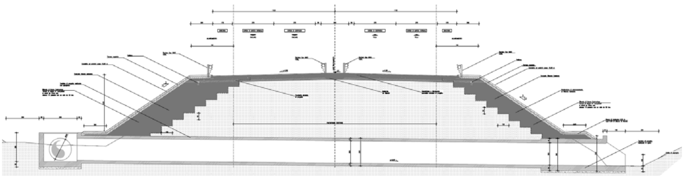
Figura 4: Sezione tipo in corrispondenza opera minore
