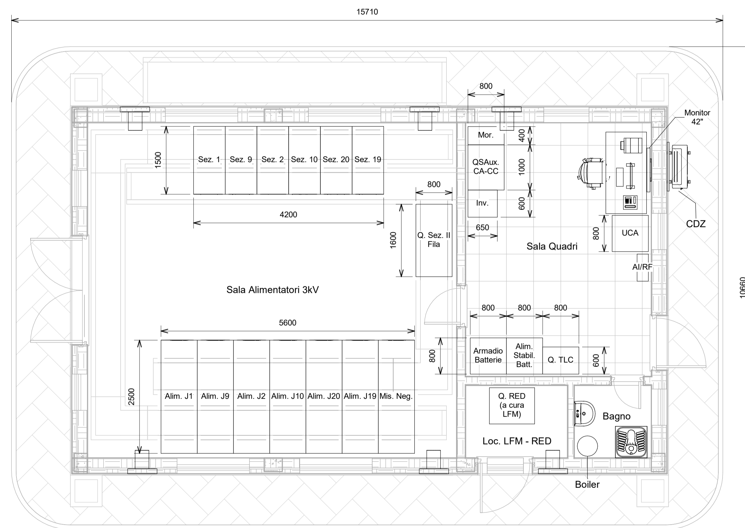
1 Disposizione apparecchiature (Layout) 1 : 50
