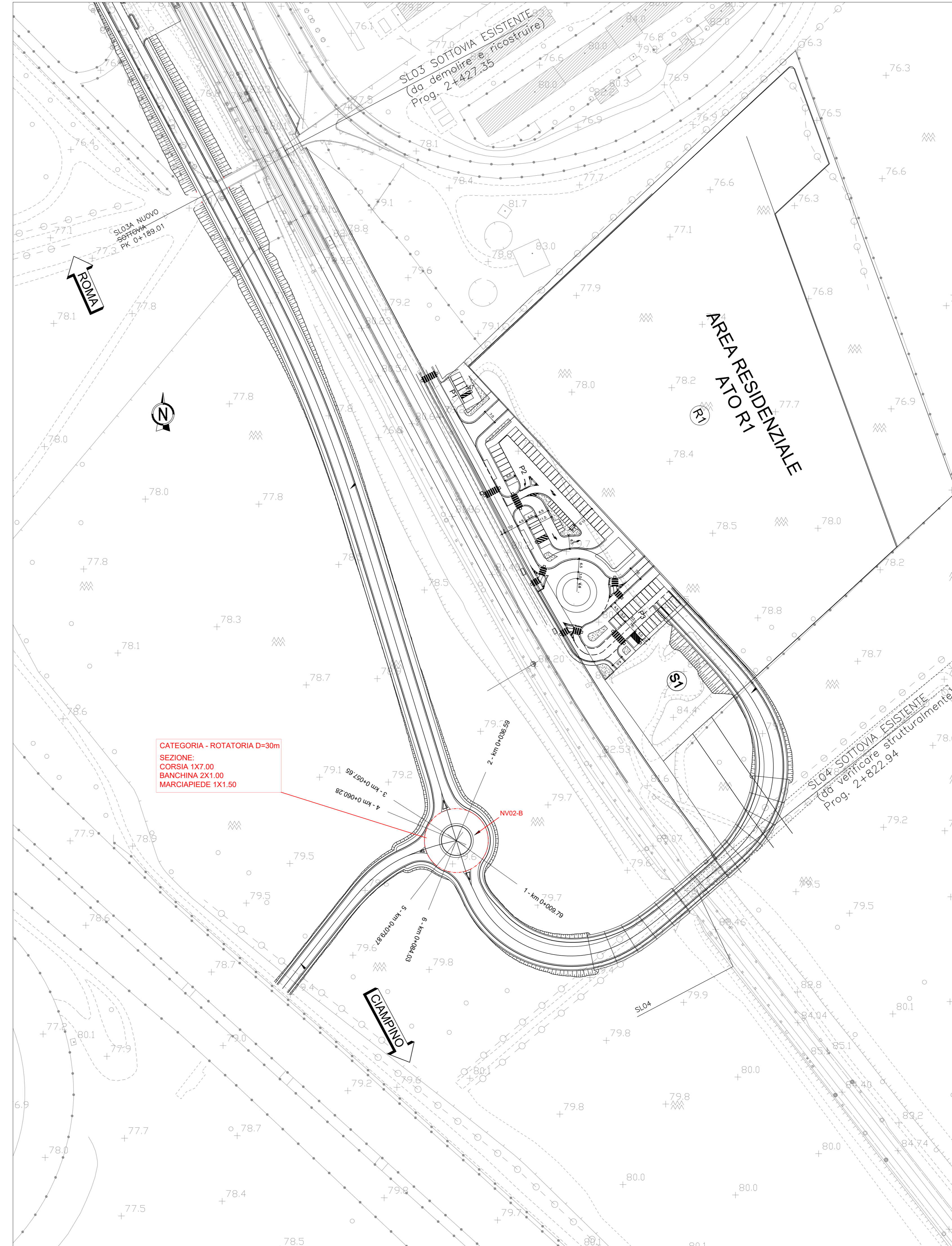
PLANIMETRIA DI PROGETTO VIABILITA' NV02B - Nuova Rotatoria scala 1:1000
