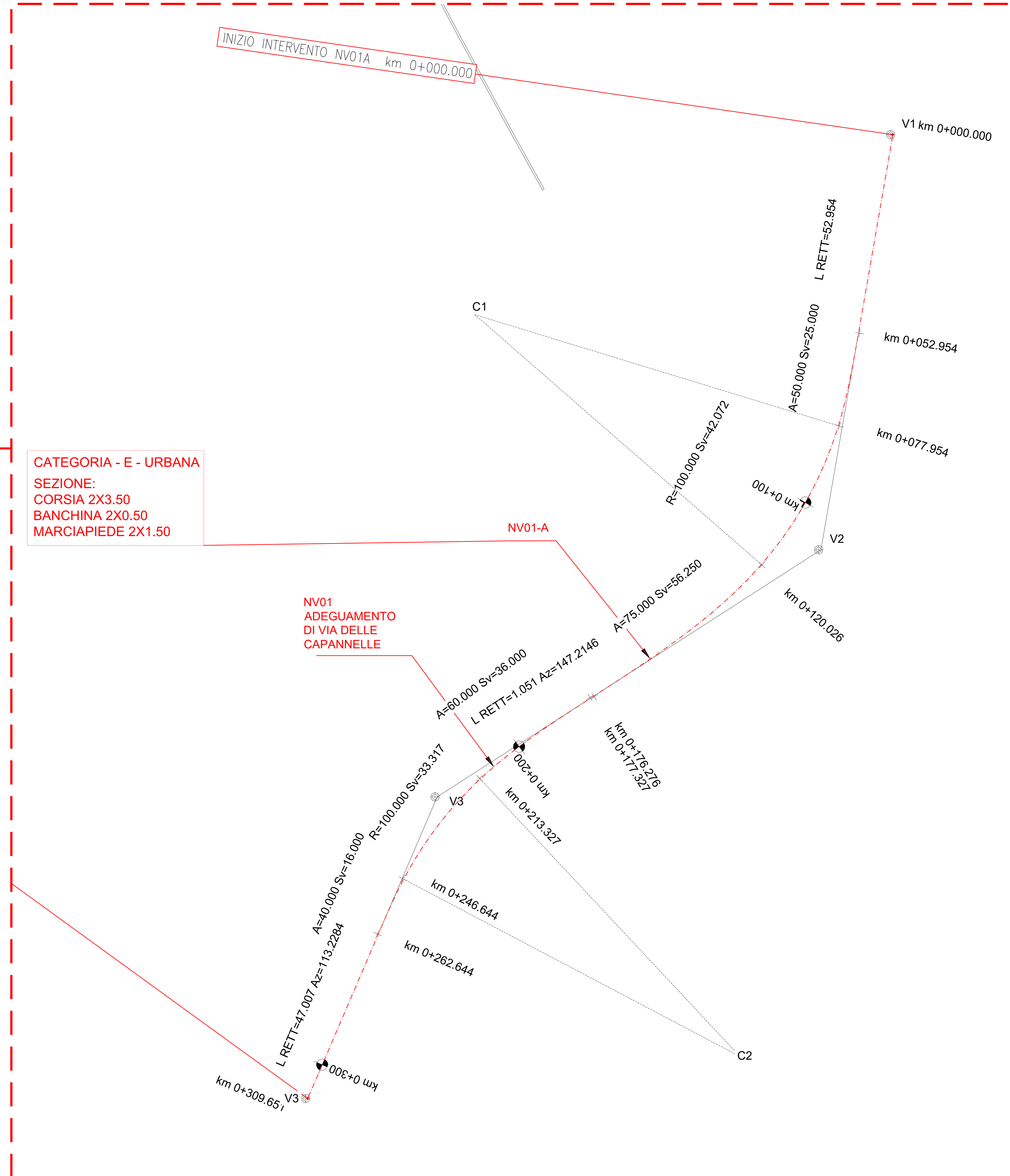
PLANIMETRIA CON DATI DI TRACCIAMENTO - VIABILITA' NV01A - VIA DELLE CAPANNELLE scala 1:500
