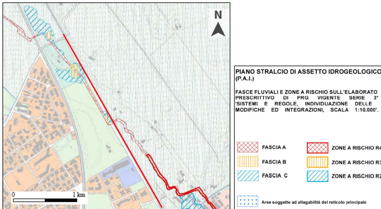
Figura 5-6 – Stralcio non in scala del foglio 18 della Carta dei Sistemi e delle Regole in scala 1:10.000 del PRG del Comune di Roma (Succhiarelli et al., 2008).
