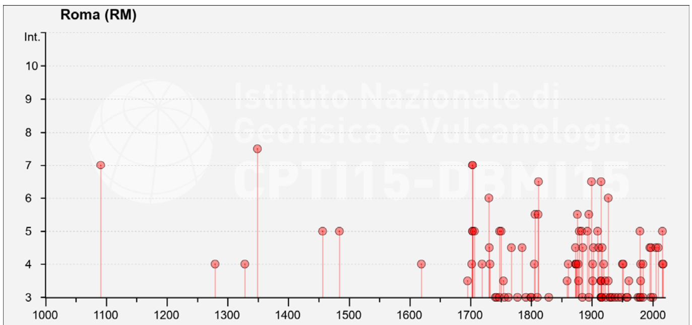
Figura 8-6 – Storia sismica del comune di Roma (dal catalogo DBMI 2015, Locati et al., 2016).
