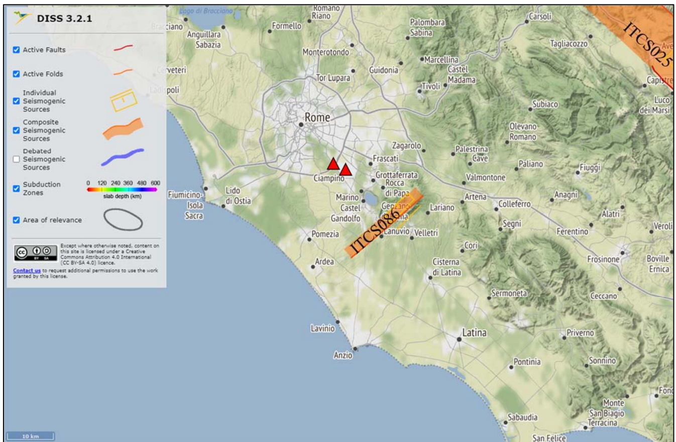
Figura 8-4 - Sorgenti sismogenetiche individuali e composite dal “Database of Individual Seismogenic Sources” (DISS 3.2) rilevanti per l’area in oggetto (gli stremi con triangoli rossi).
