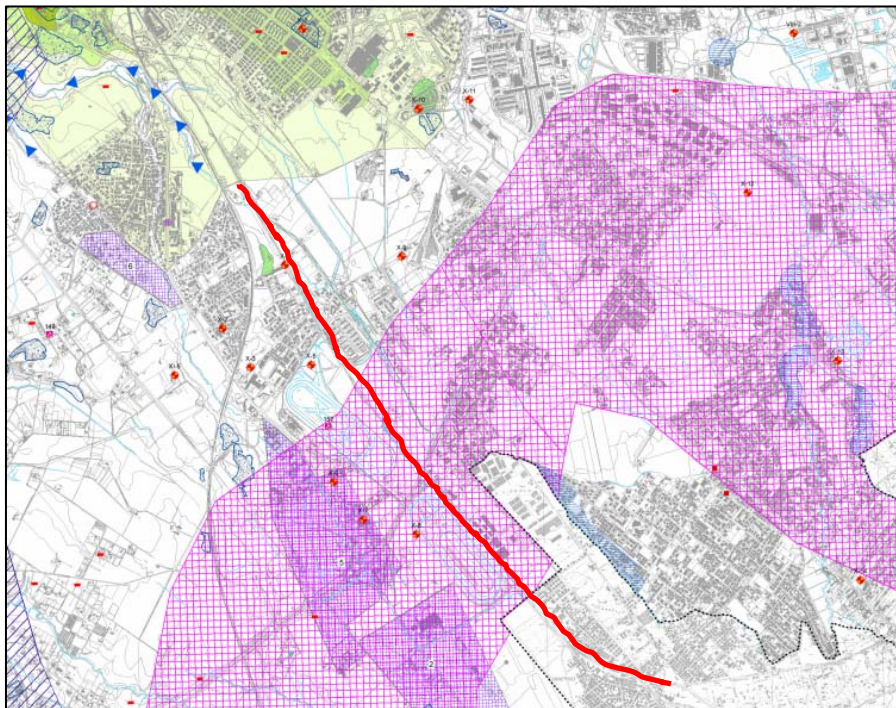
Figura 5-1 – Stralcio non in scala della carta della pericolosità e della vulnerabilità geologica del PRG del Comune di Roma (Succhiarelli et al., 2008)
