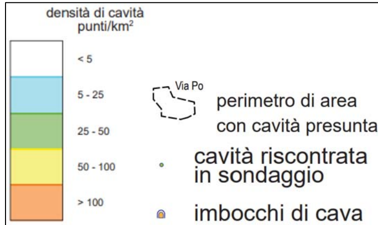
Figura 5-4 Legenda della carta delle cavità sotterranee di Roma (Nisio et al., 2017)
