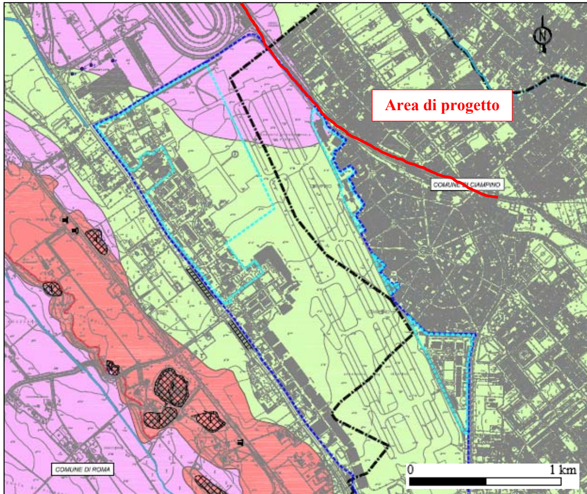
Figura 4-2 Carta geologica realizzata in scala 1:5.000 (Canuti et al.; 2015) e redatta da Aeroporti di Roma per l'aeroporto di G.B Pastine di Ciampino. In rosso è evidenziata la linea oggetto di quadruplicamento della linea ferroviaria al quale si riferisce il presente elaborato.
