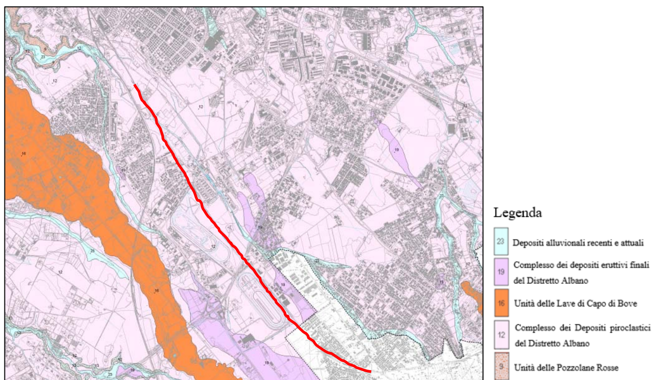
Figura 4-1 Stralcio non in scala del foglio VI della carta geolitologica realizzata in scala 1:20.000 per il PRG del Comune di Roma (Succhiarelli et al., 2008)
