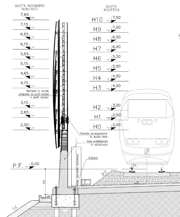
Figura 3 - Sezione trasversale barriera antirumore verticale
