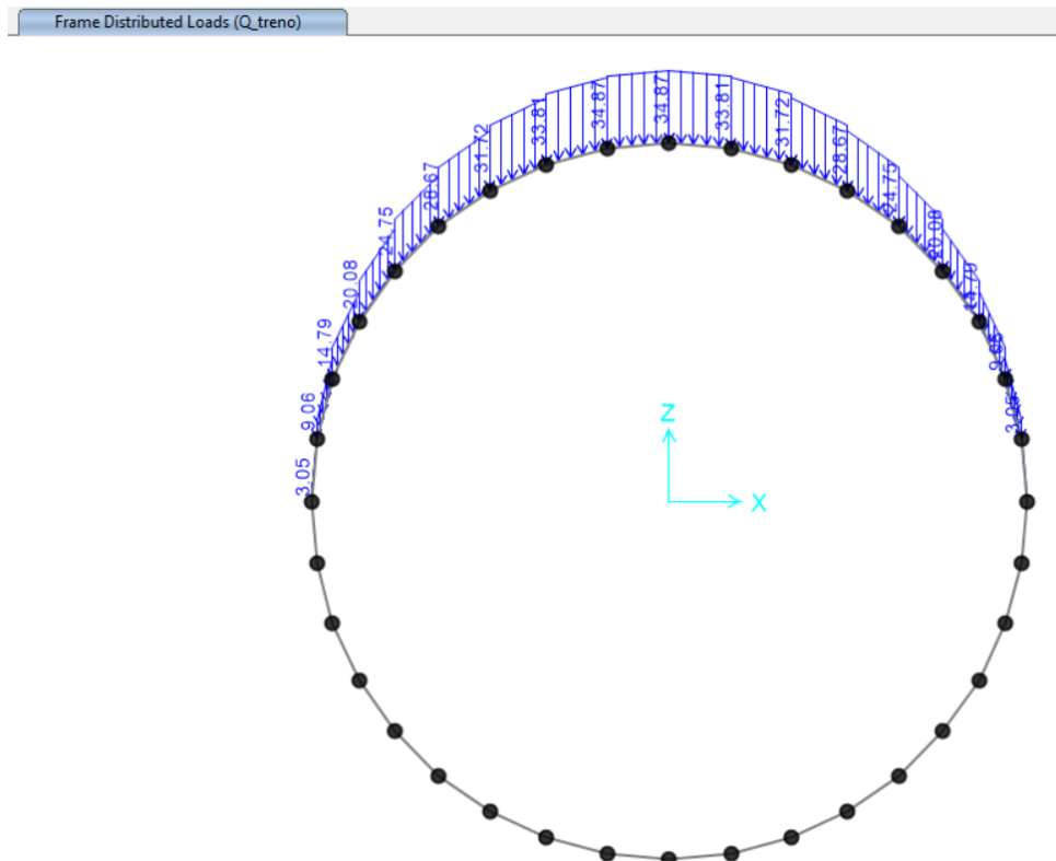
Figura - 16 Qtrn1- Carico del treno
