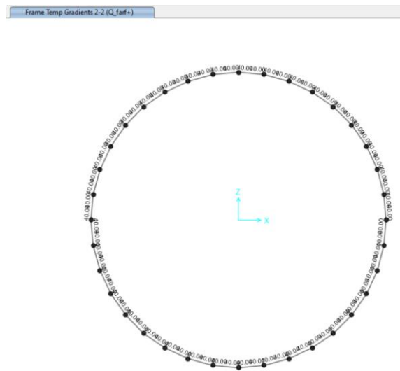
Figura - 19 Q_Temp_Farfalla+
