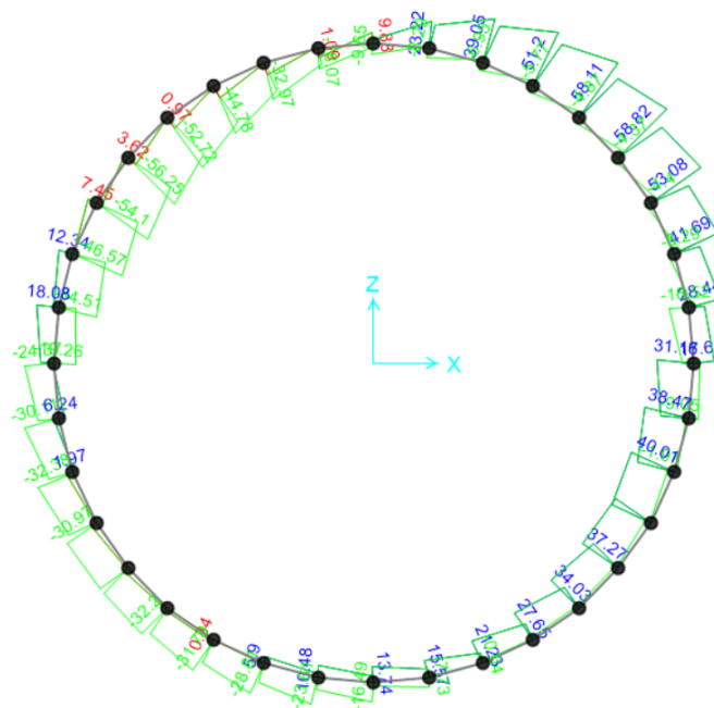
Figura - 29 SOLETTA SLE – V2 max./min.
