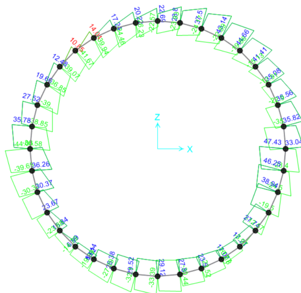
Figura - 35 SOLETTA SLV -V2 max./min.
