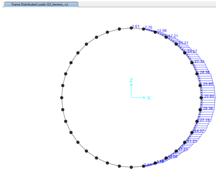
Figura - 7 G3 Spinta_H_X-
