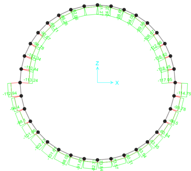
Figura - 33 SOLETTA SLV – AXIAL max./min.
