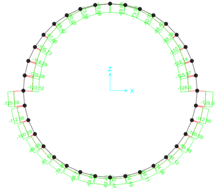
Figura - 27 SOLETTA SLE - AXIAL max./min.
