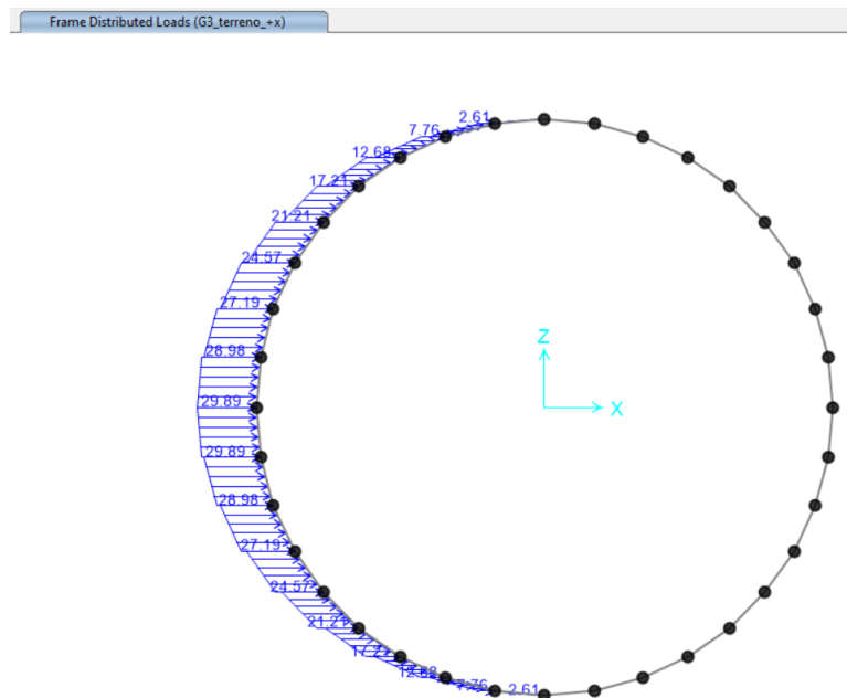
Figura - 6 G3 Spinta_H_X+
