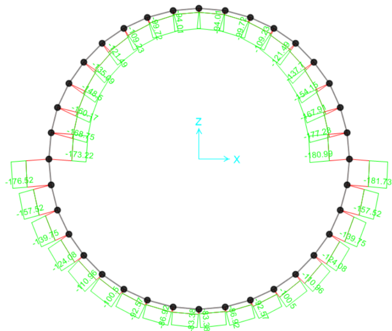
Figura - 30 SOLETTA SLU – AXIAL max./min.
