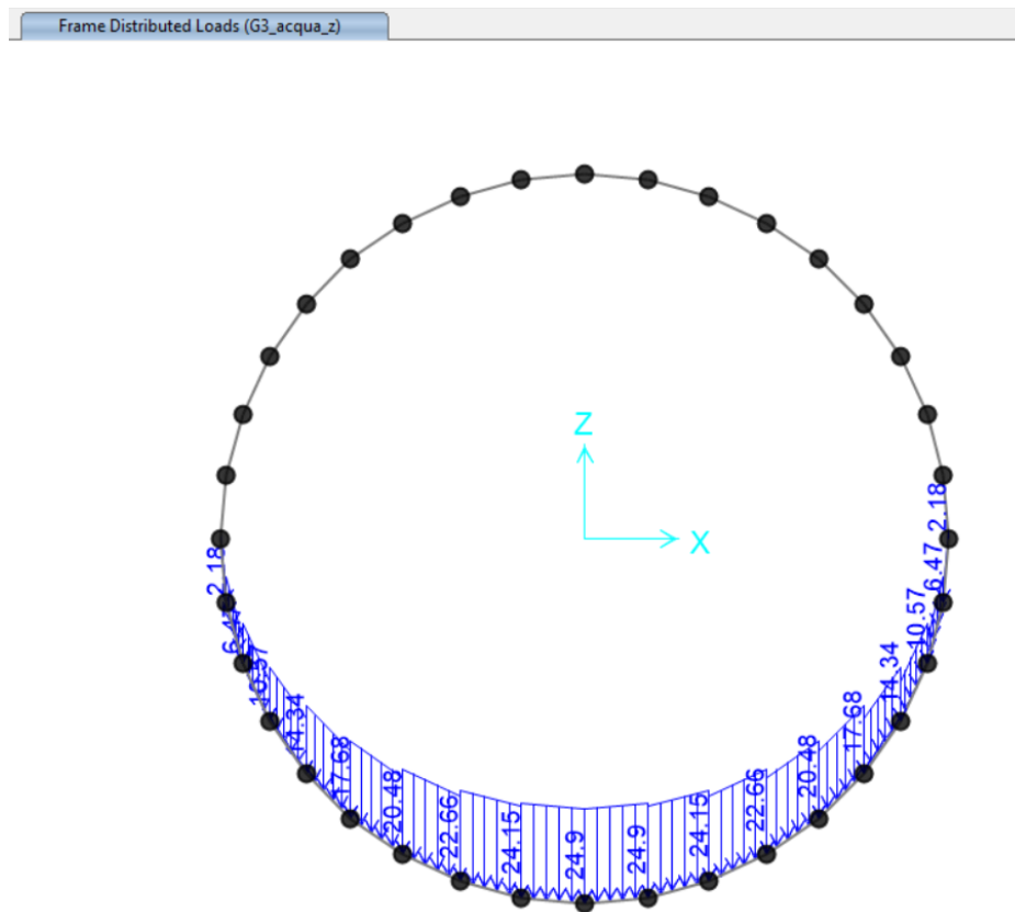
Figura - 11 G3 Acqua_V
