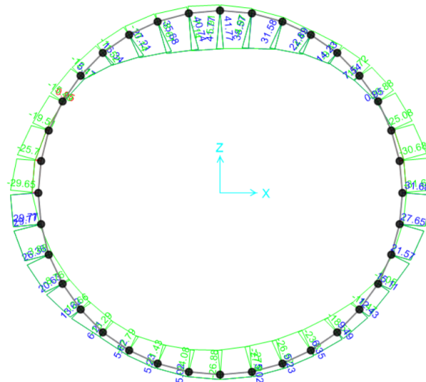
Figura - 28 SOLETTA SLE – M3 max./min.
