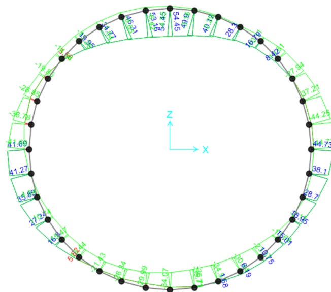
Figura - 31 SOLETTA SLU – M3 max./min.
