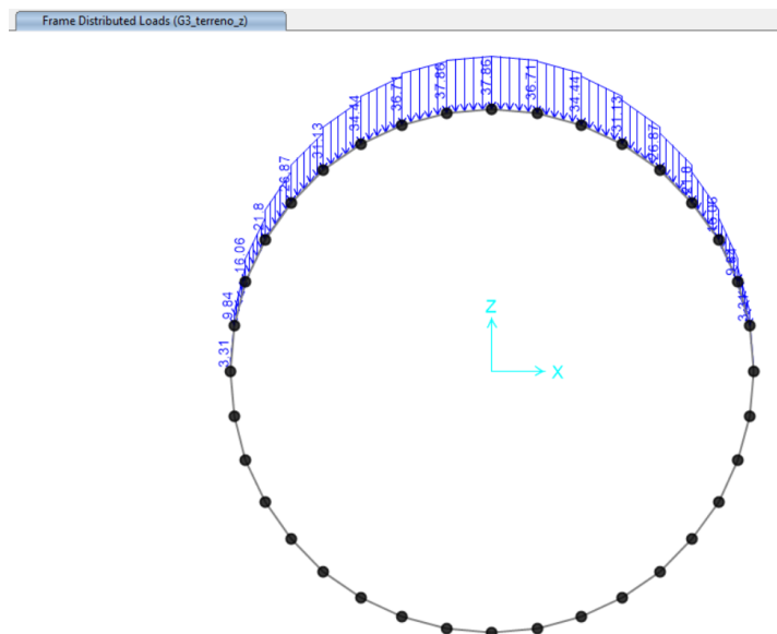
Figura - 8 G3 Verticale del Terreno
