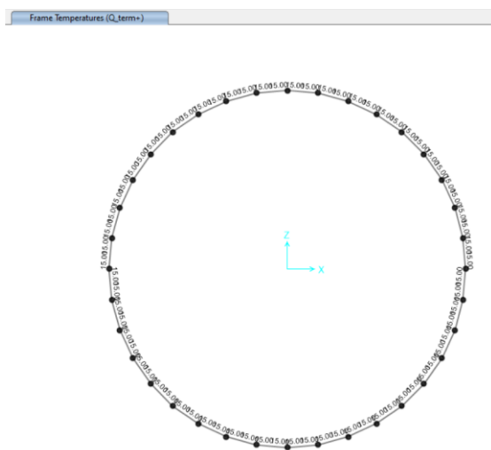
Figura - 17 Q_Temp_Uni+
