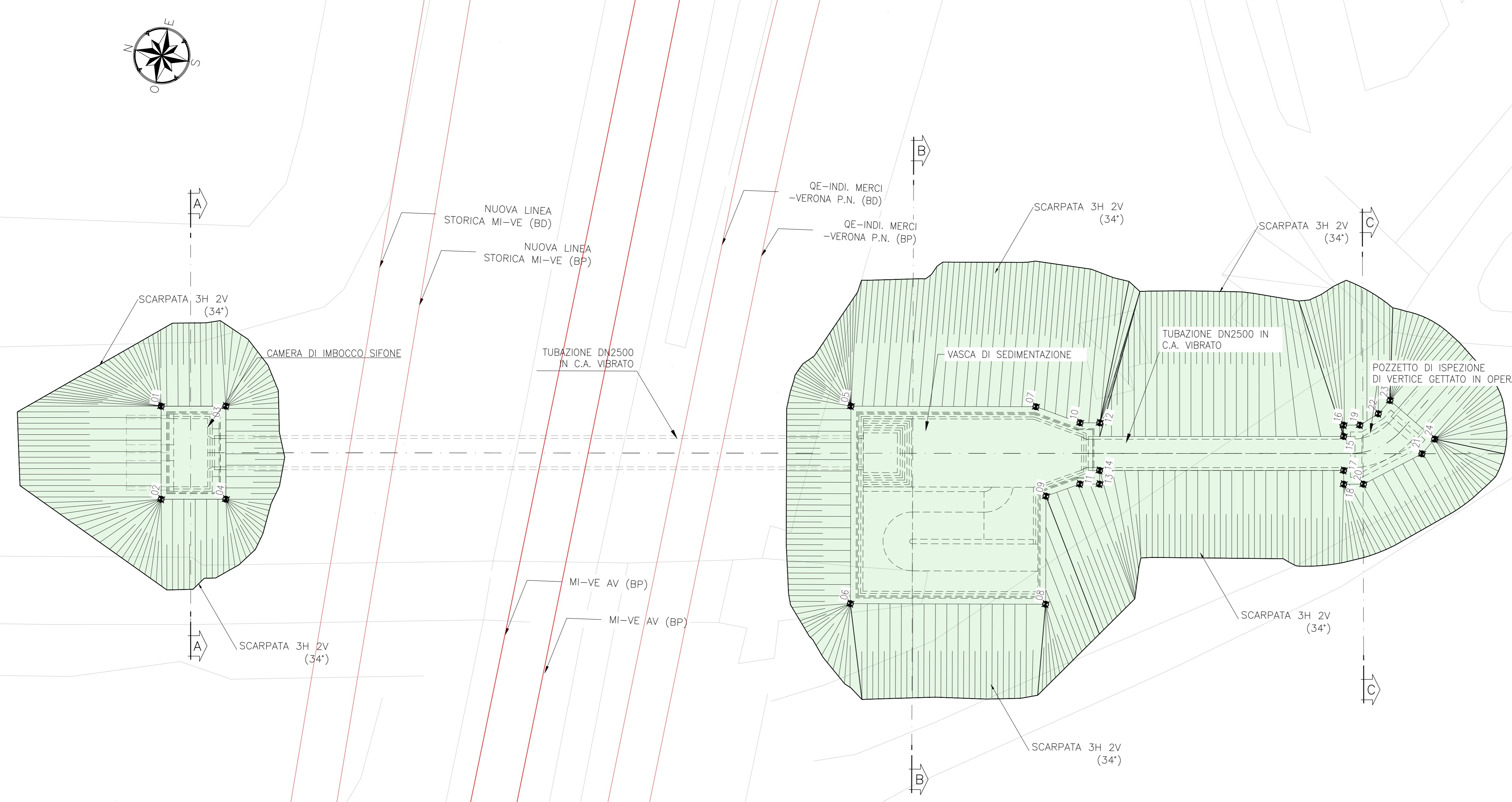
PLANIMETRIA SCALA 1:200
