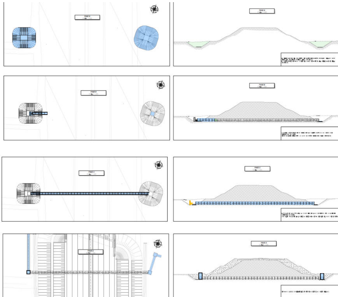
Figura 8 - Fasi progettuali
