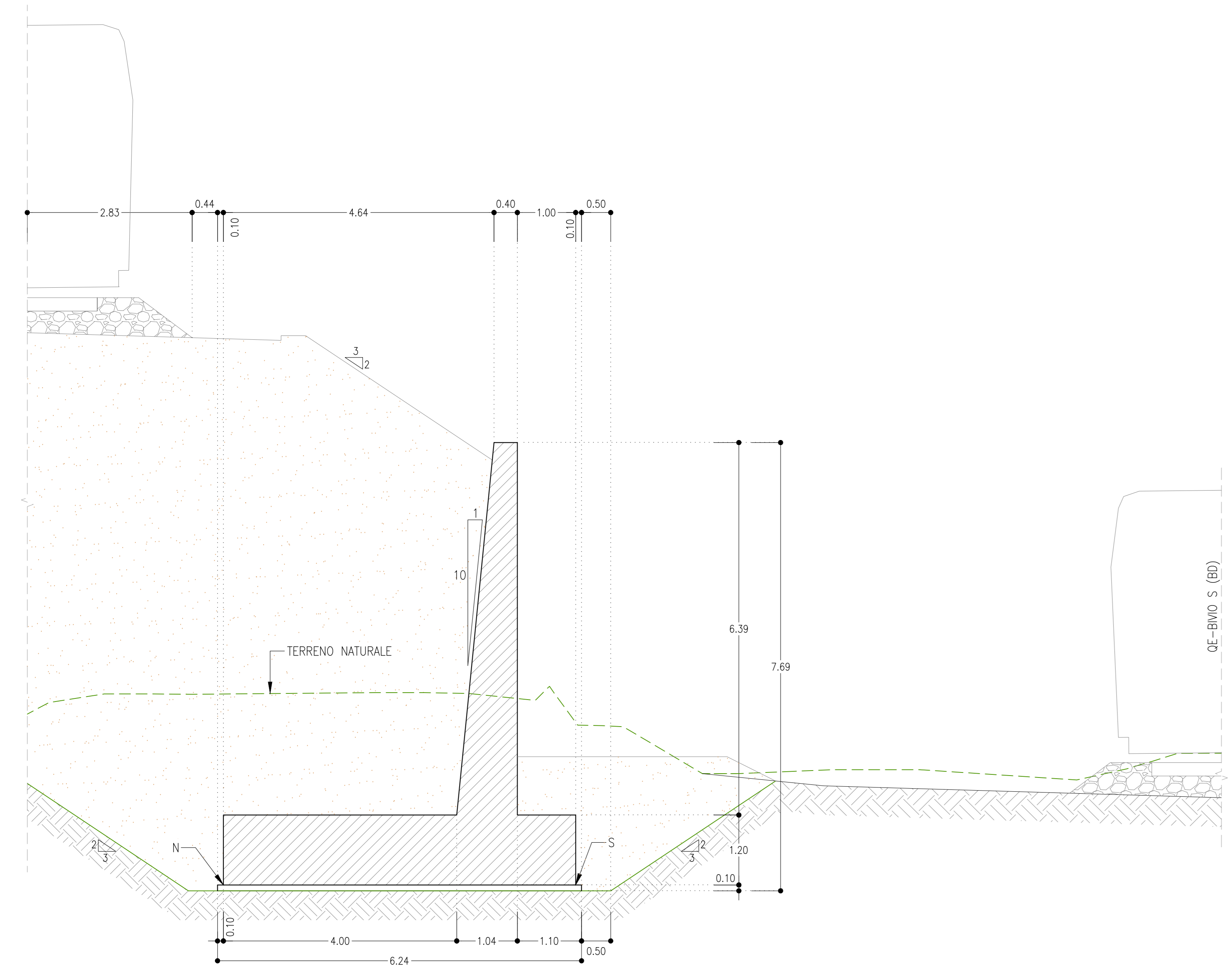
SEZIONE MURI - MU05 SCALA 1:50 SEZIONE TRASVERSALE
