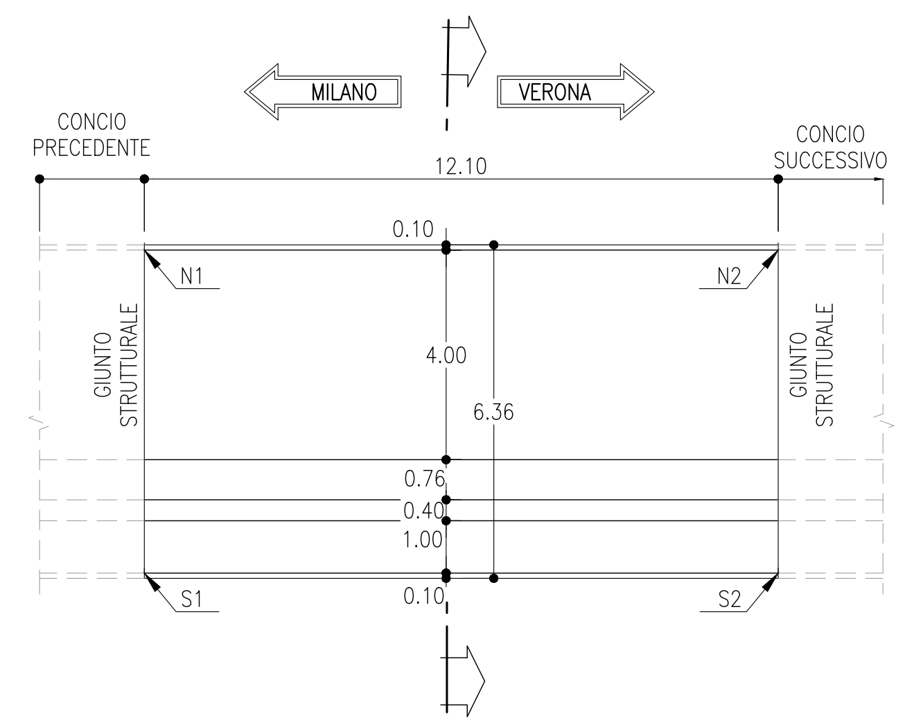
PIANTA TIPOLOGICA SCALA 1:100
