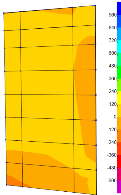
Diagramma momenti M22
