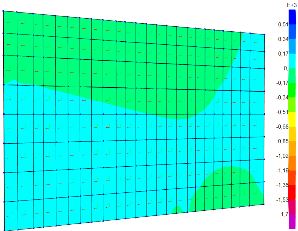
Diagramma momenti M11
