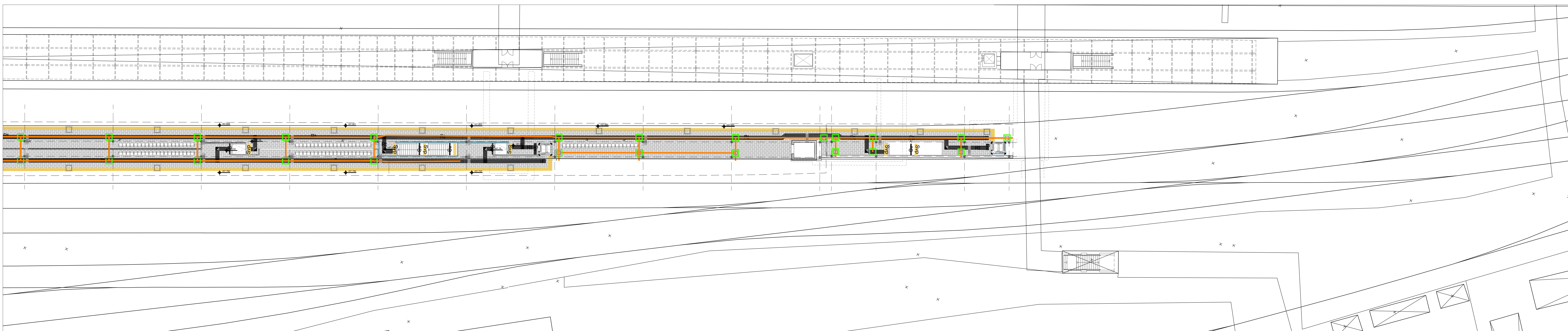
PLANIMETRIA QUADRO 2 - SCALA 1:200
