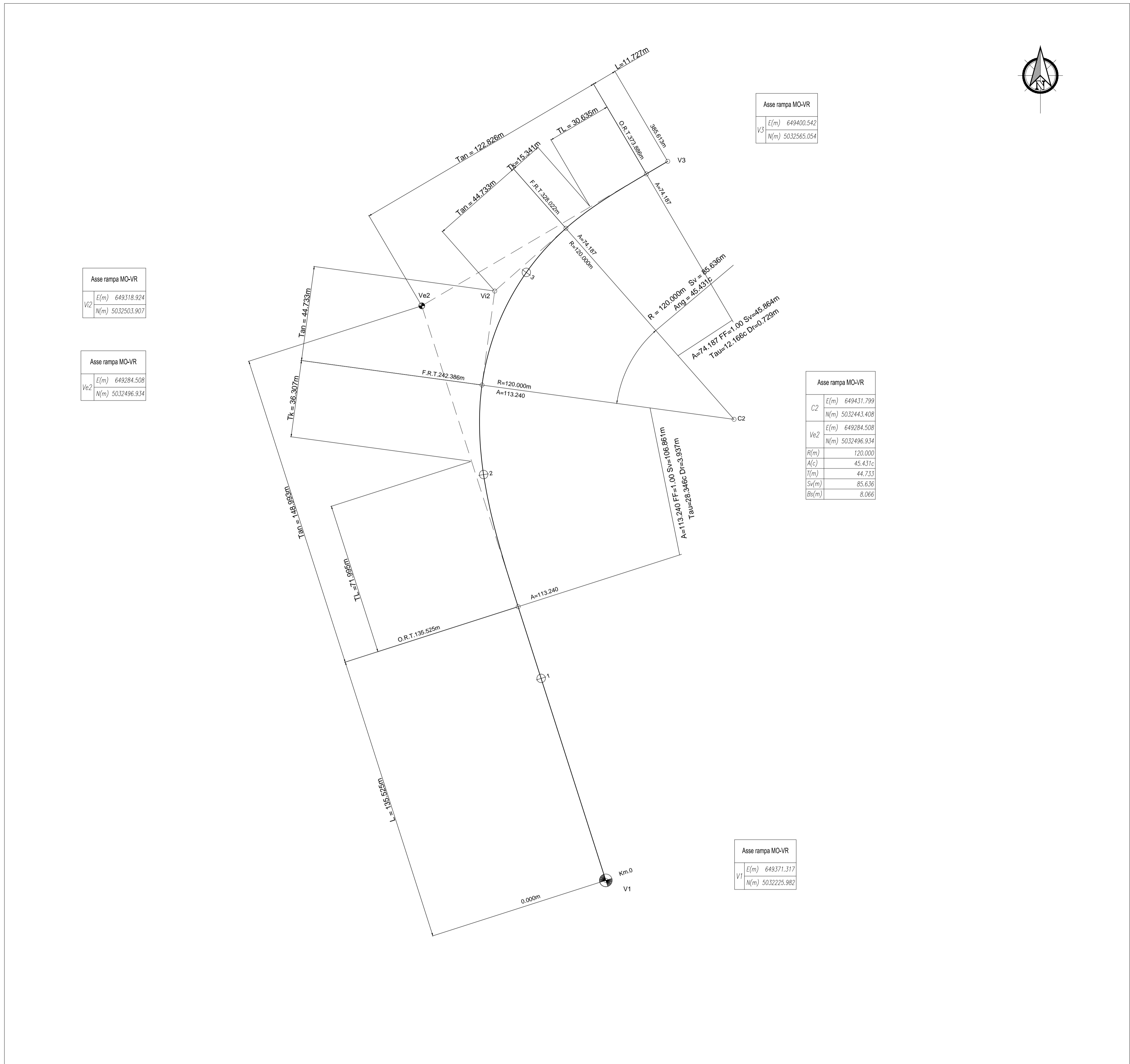
PLANIMETRIA DI TRACCIAMENTO - Asse Rampa MO-VR SCALA 1:1.000
