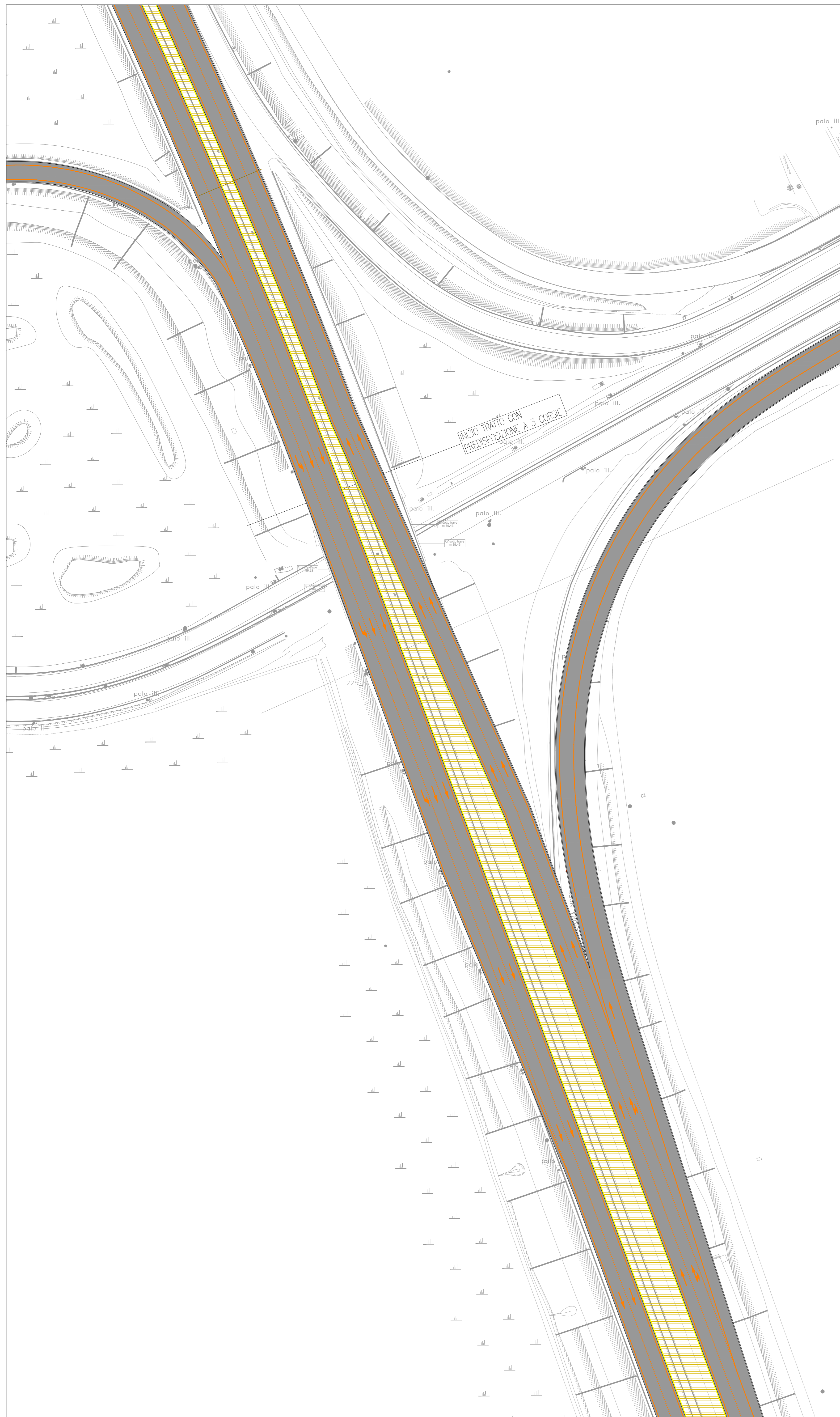
TRACCIAMENTO DEVIAZIONI - FASE 1b - QUADRO 1 SCALA 1:500
