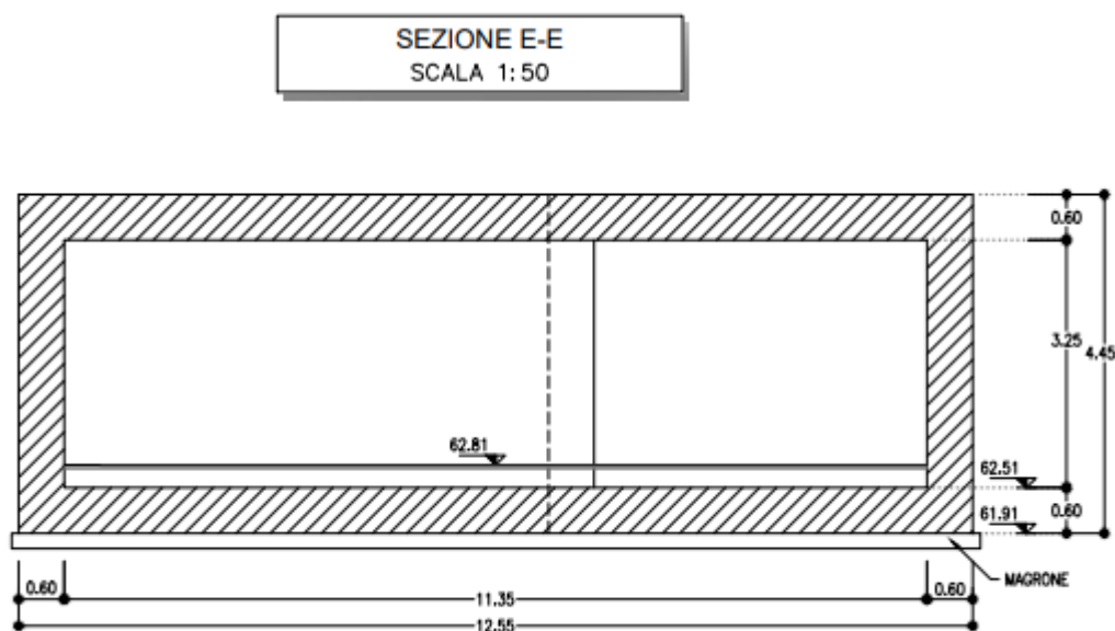
Figura 8 - Sezione trasversale E-E
