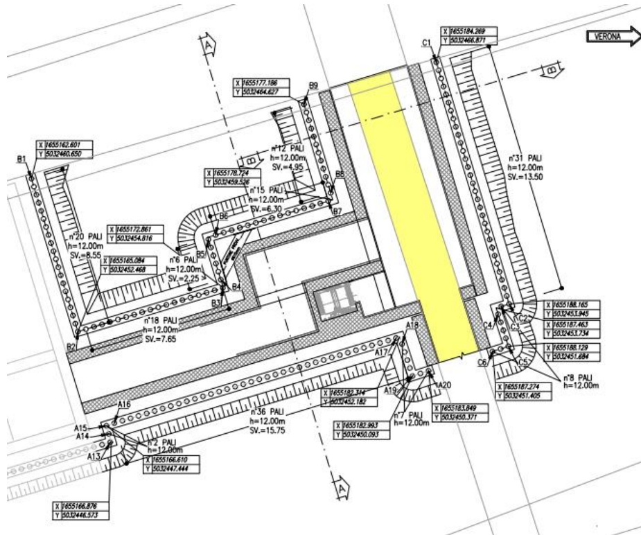
Figura 6 - Stralcio planimetrico della parte interrata
