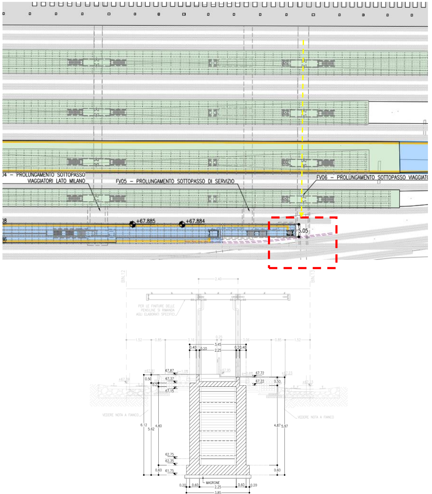
Figura 5 – FV06 Prolungamento sottopasso viaggiatori lato VENEZIA
