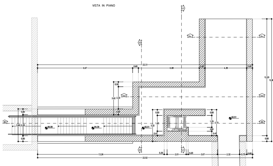
Figura 9 - Carpenteria opere in c.a.
