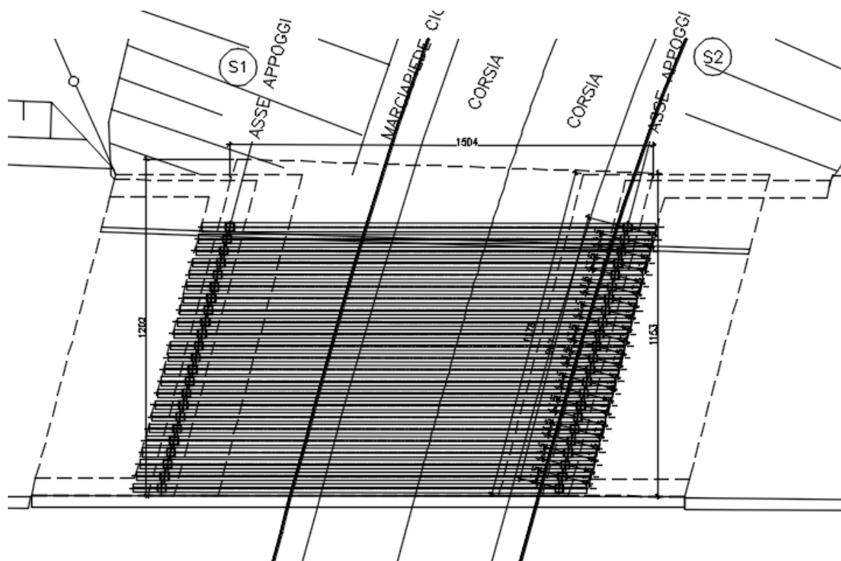
Figura 1-2 Pianta impalcato
