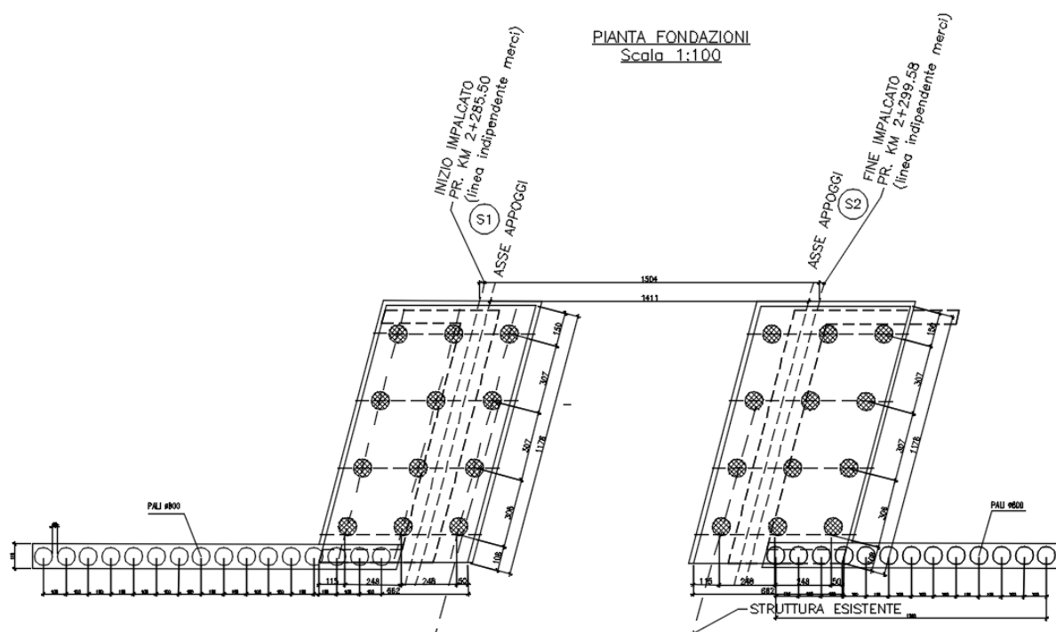
Figura 1.5 Spalla - Pianta delle fondazioni
