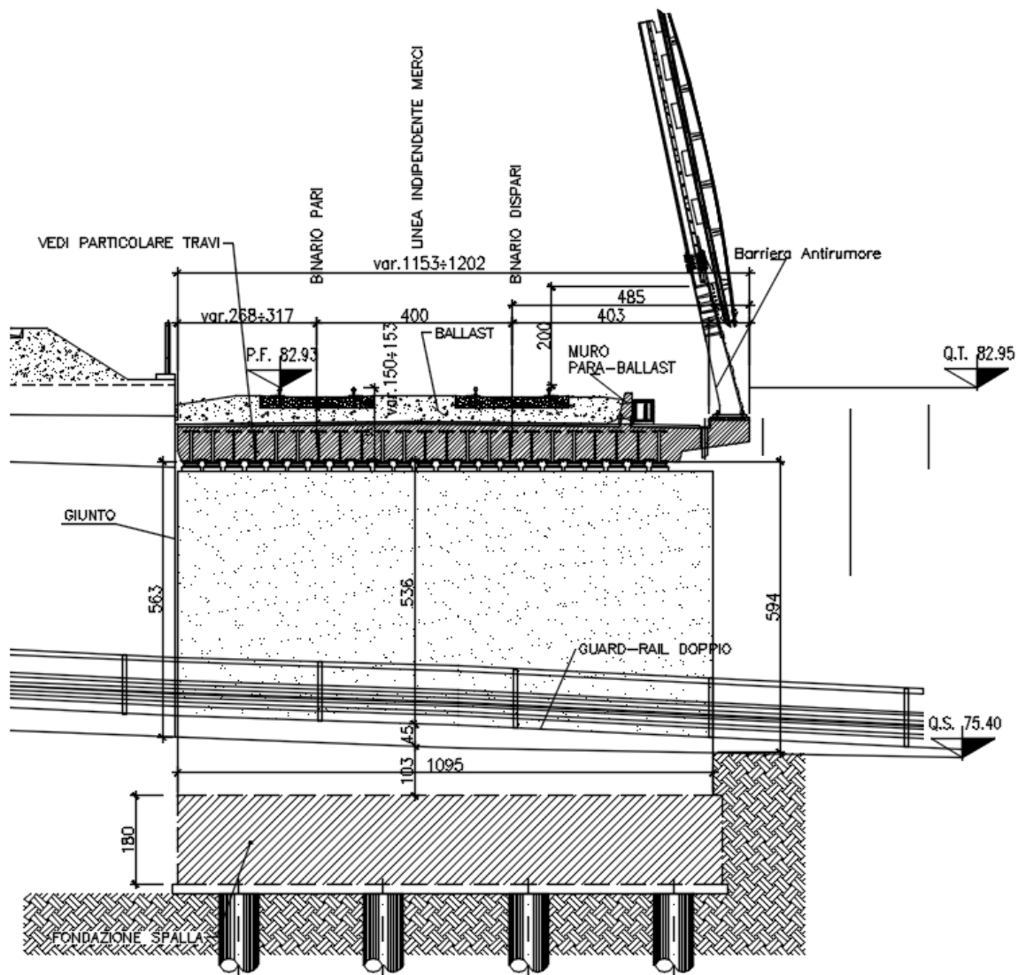
Figura 1-4 Sezione trasversale
