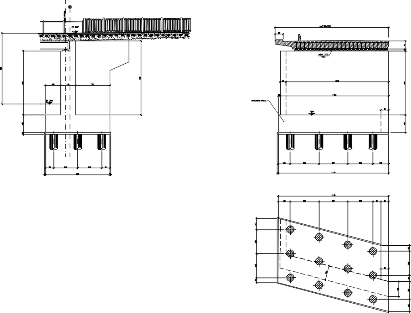
Figura 1.6 Spalla - Viste spalla
