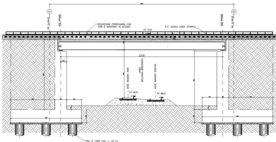
Figura 1.6 Spalla - Viste spalla
