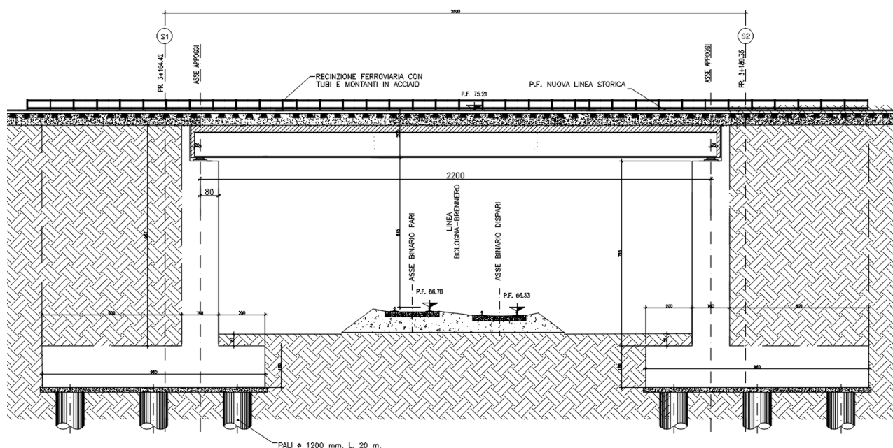
Figura 1-3 Sezione longitudinale
