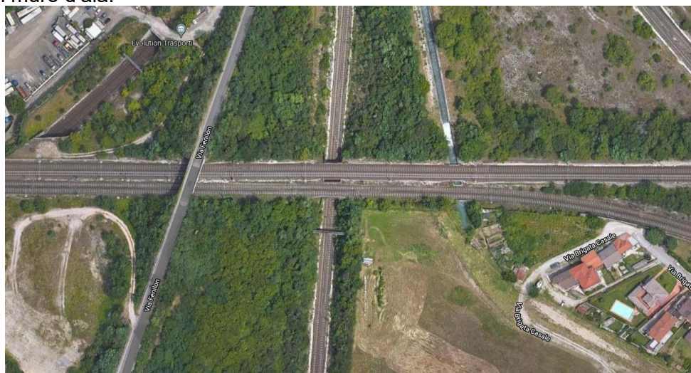
Figura 1.1 Vista planimetrica stato di fatto
