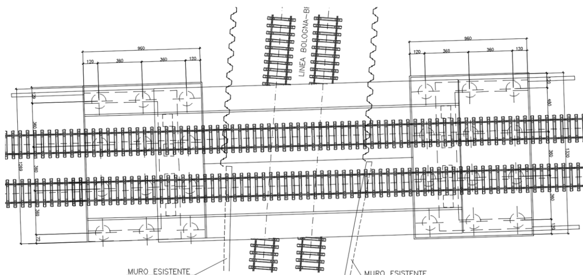
Figura 1.5 Spalla - Pianta delle fondazioni
