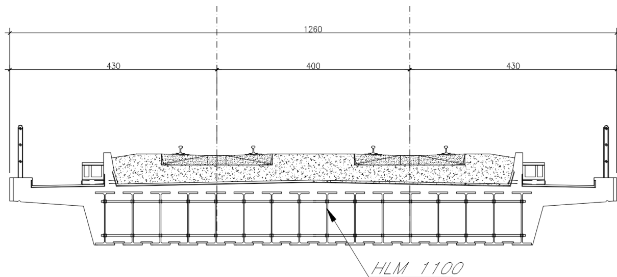
Figura 1-4 Sezione trasversale
