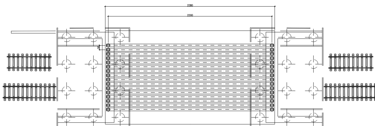
Figura 1-2 Pianta impalcato
