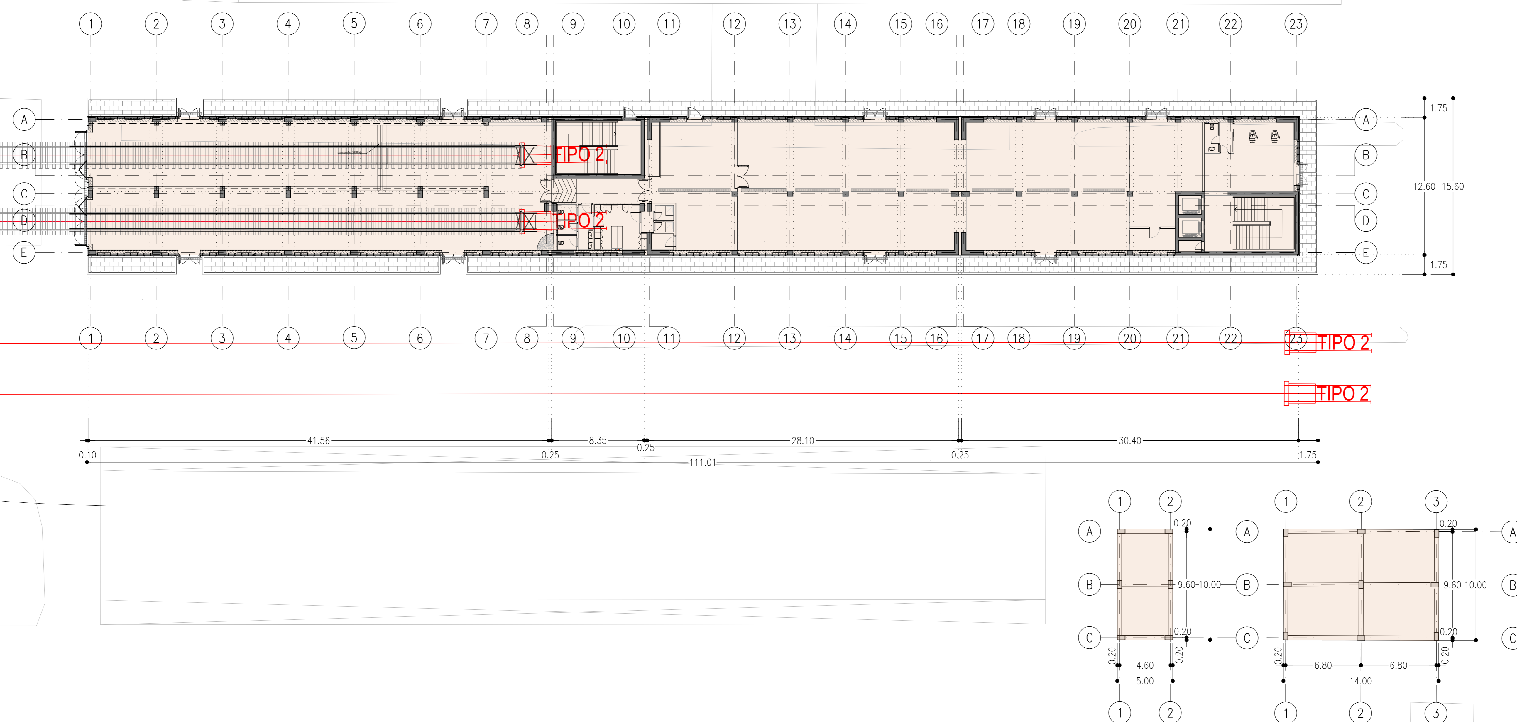
PLANIMETRIA SCALA 1: 200
