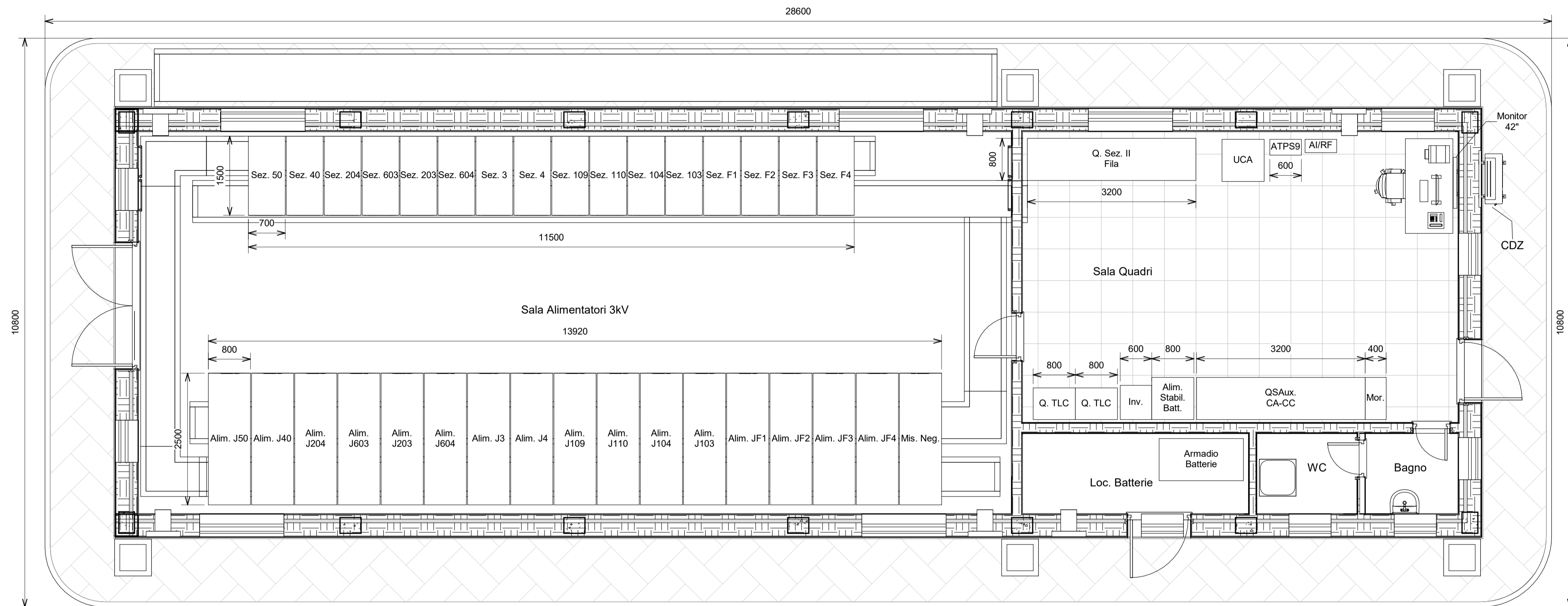
1 Disposizione apparecchiature (Layout) 1 : 50
