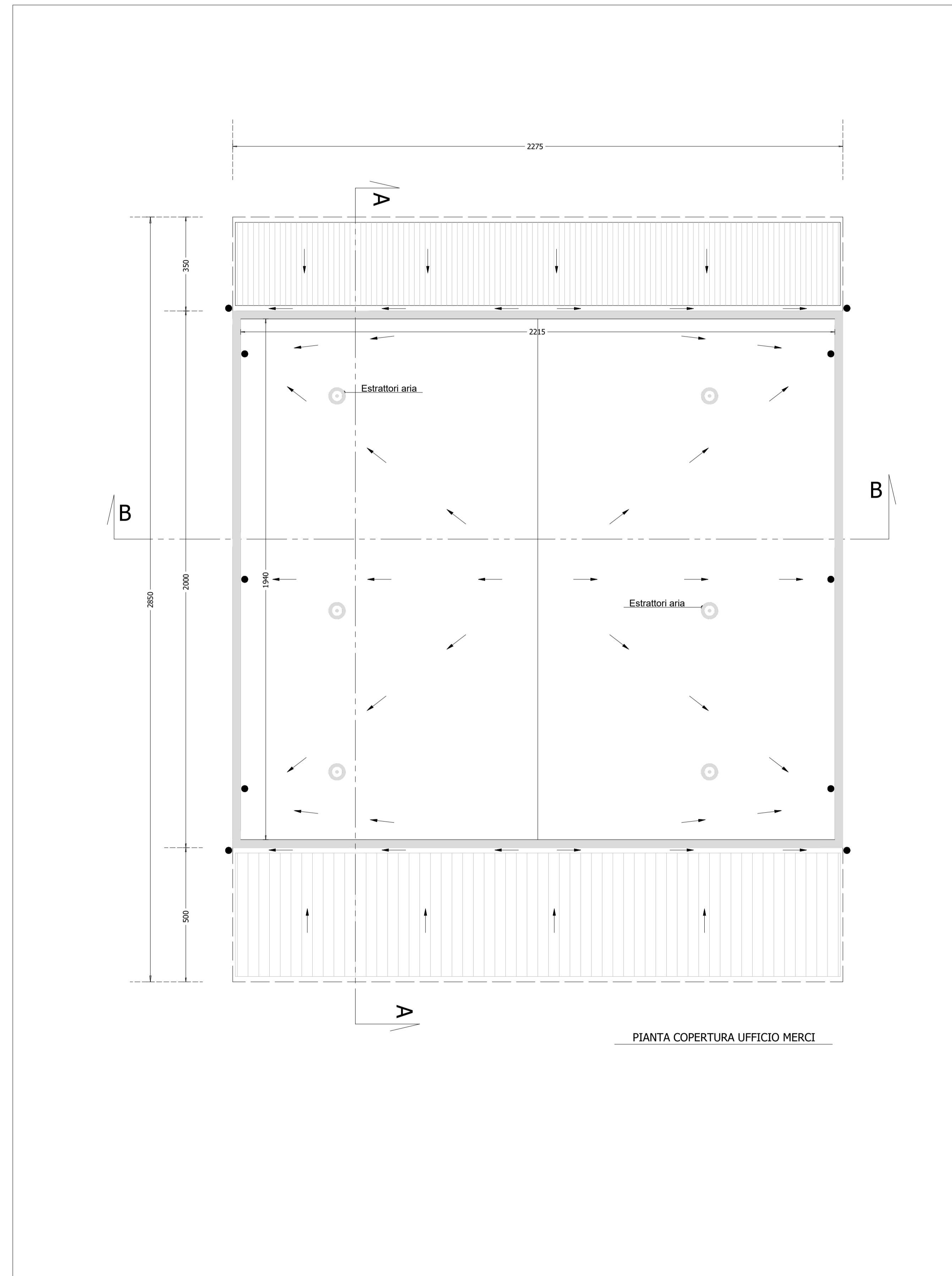
PIANTA COPERTURA
