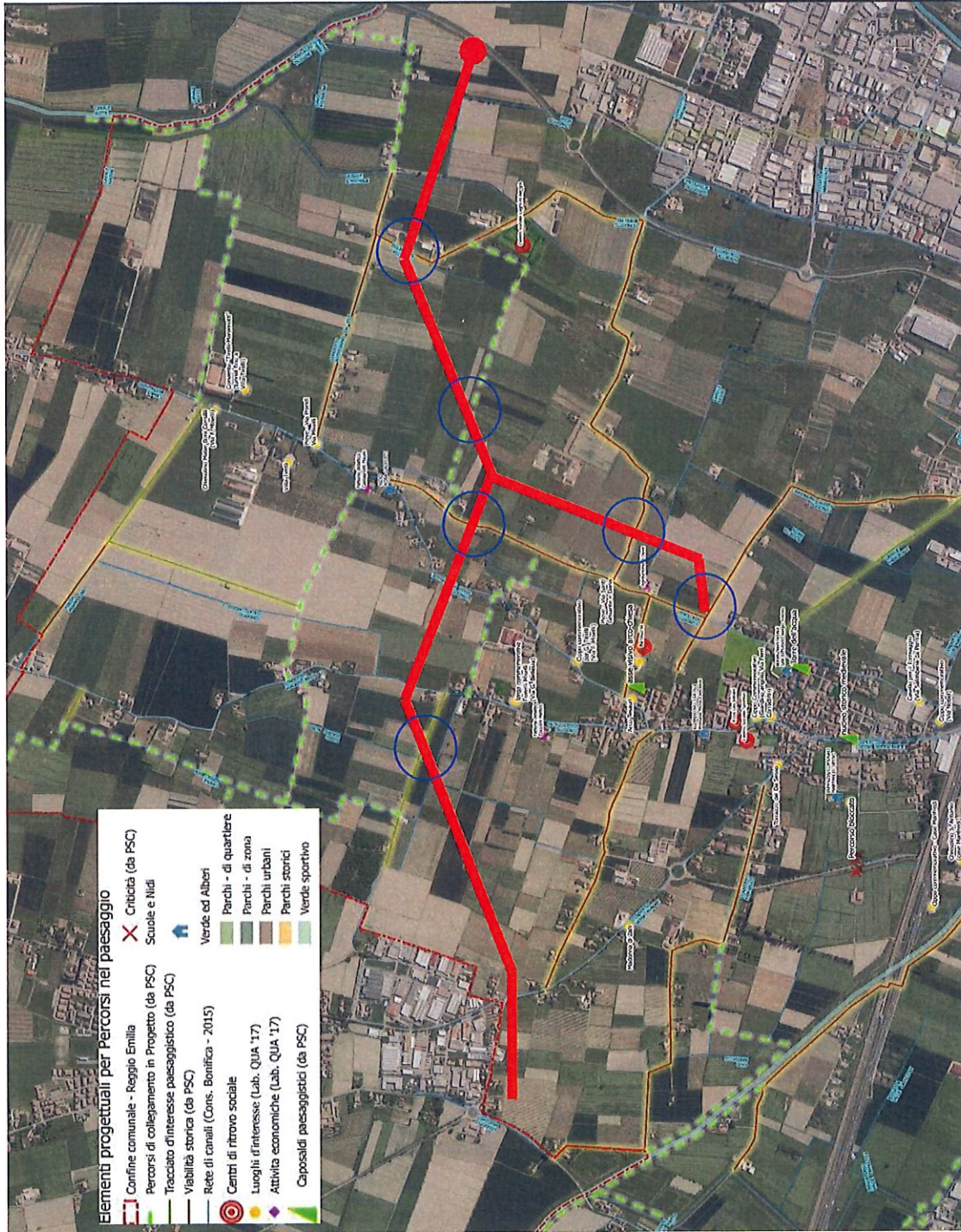
Figura 15 – Percorsi di storia nel Paesaggio ed interferenze (cerchi blu) della nuova linea aerea (in rosso)
