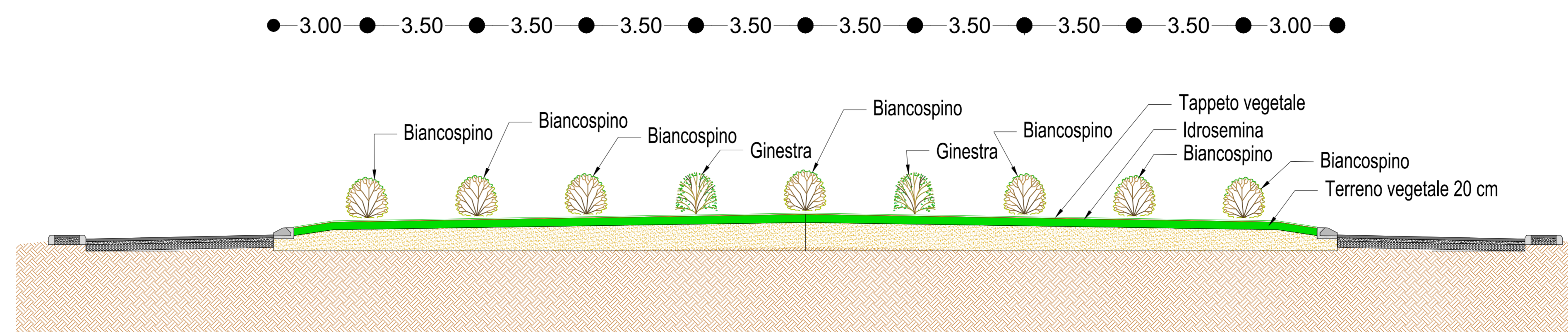
SEZIONE TIPO A ROTATORIA SUD
