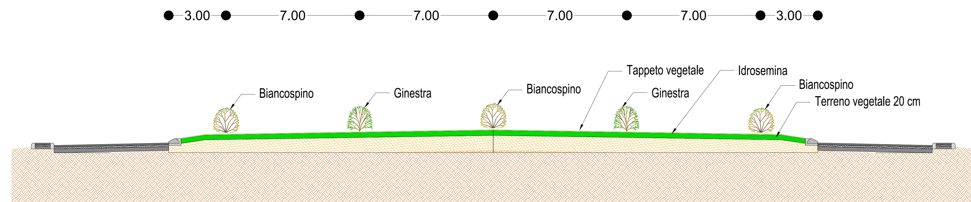
SEZIONE TIPO B ROTATORIA SUD
