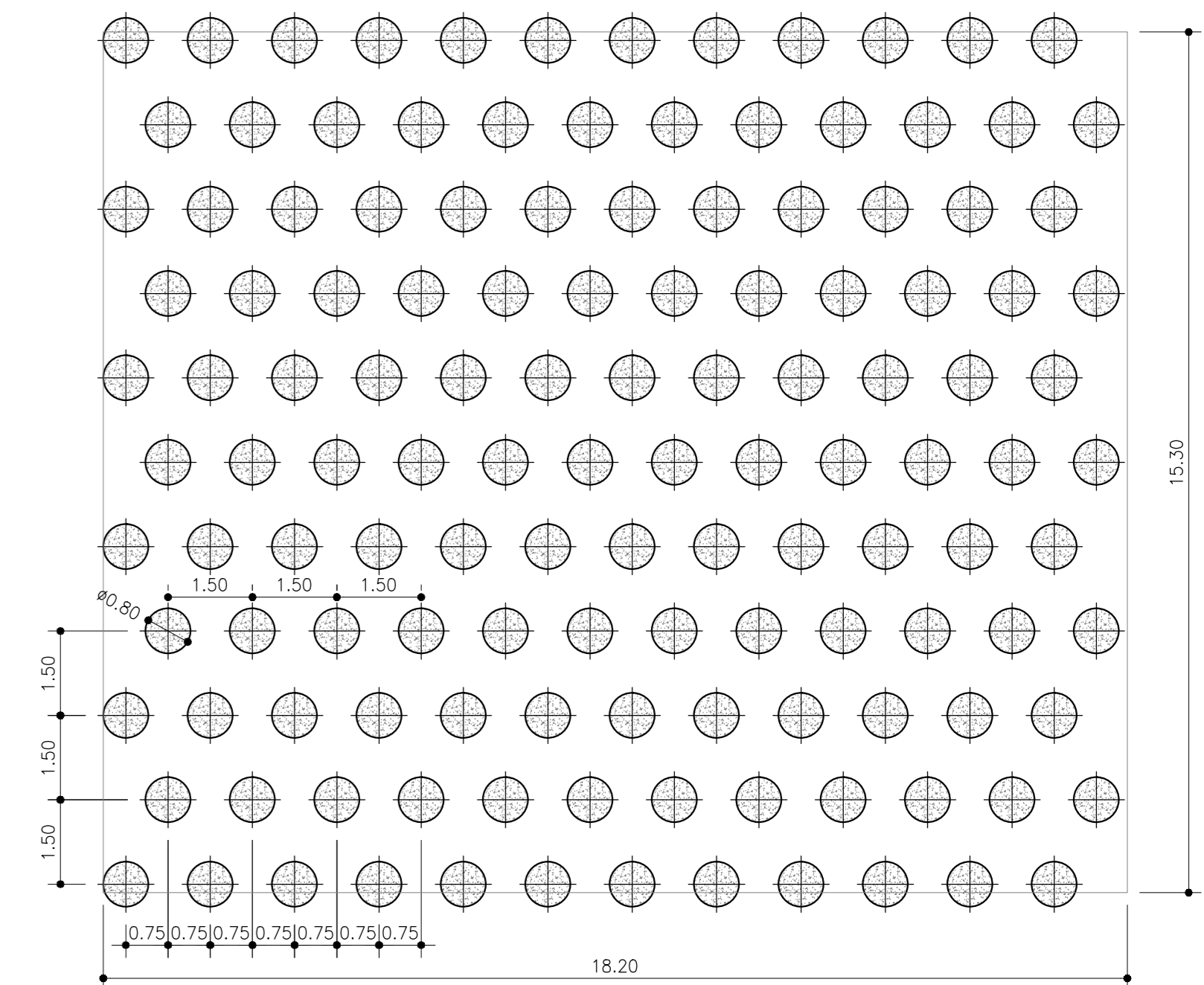
DISPOSIZIONE COLONNE JET GROUTING SCALA 1:100
