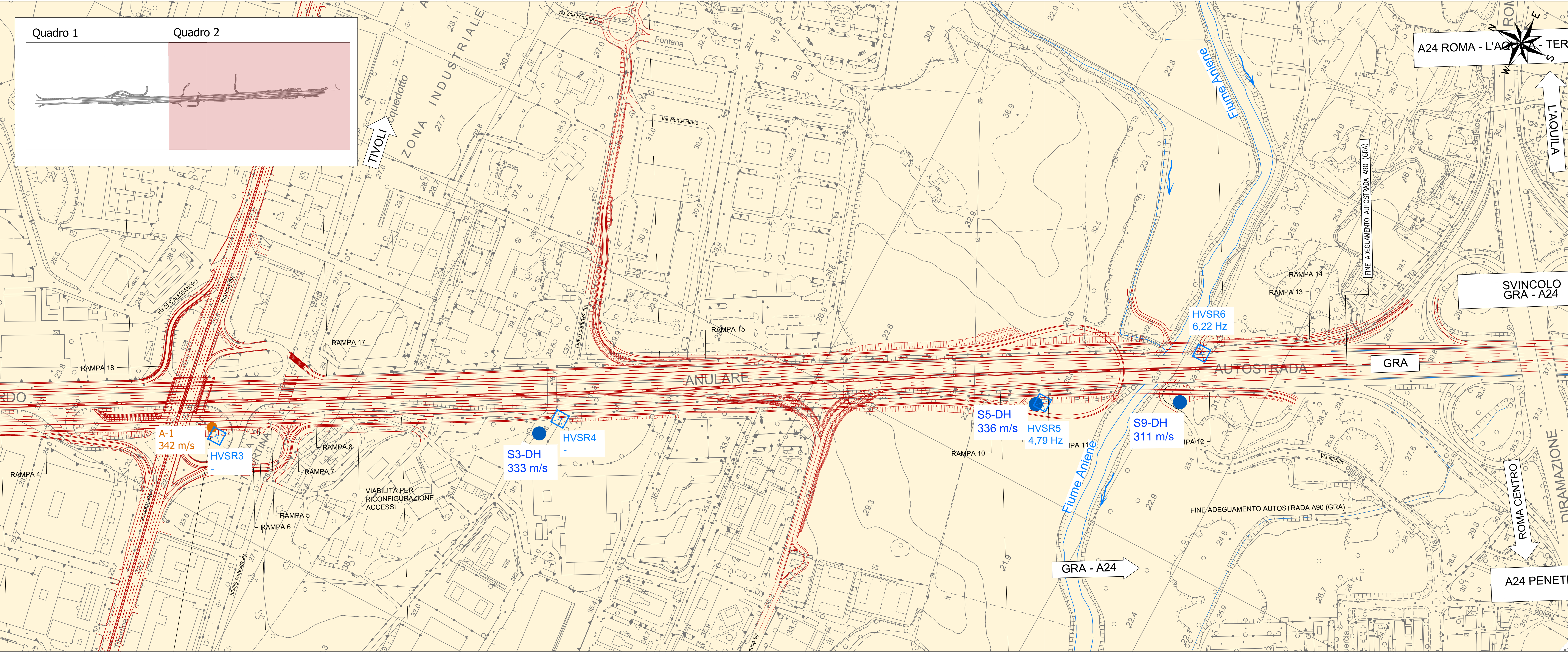
Carta sismica - Scala 1:2000 - Quadro 2
