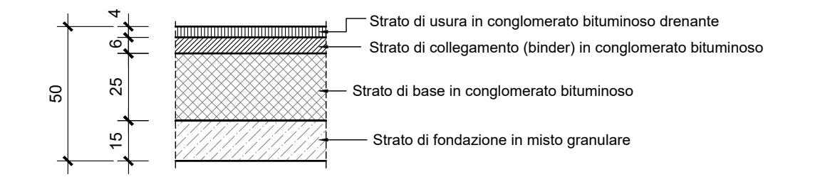
PARTICOLARE DELLA PAVIMENTAZIONE VIABILITÀ COMPLANARI E RAMPE Scala 1:20
