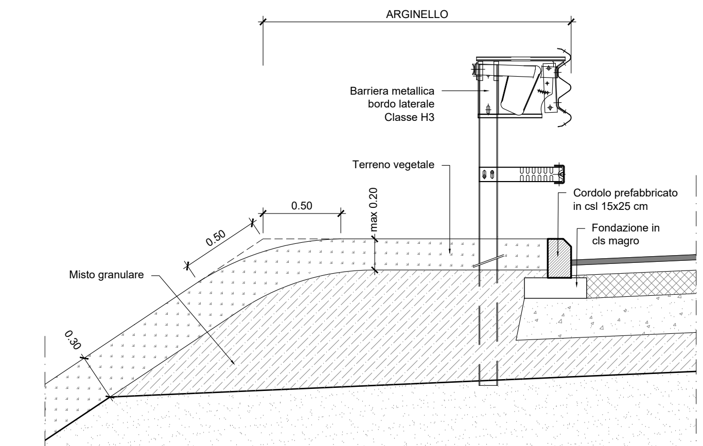
DETTAGLIO ARGINELLO SCALA 1:25
