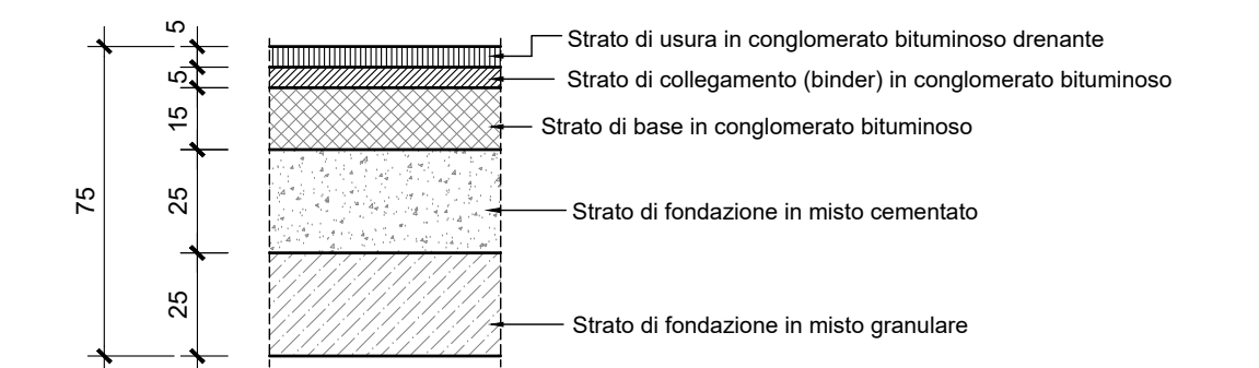
PARTICOLARE DELLA PAVIMENTAZIONE G.R.A. Scala 1:20
