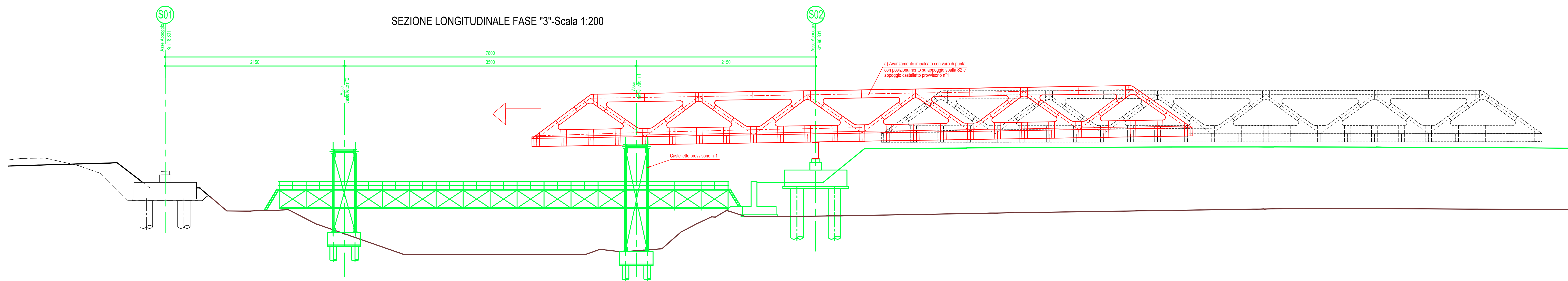
SEZIONE LONGITUDINALE FASE "3"-Scala 1:200
