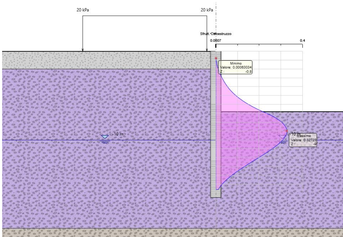
Figura 24 - Verifica tensioni di esercizio nel calcestruzzo
