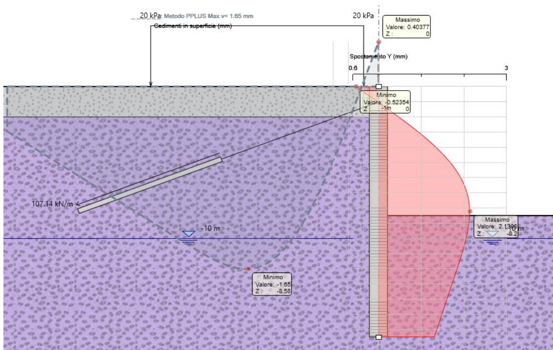
Figura 28 - Involucro spostamenti allo SLE. |umax|=2.14 mm
