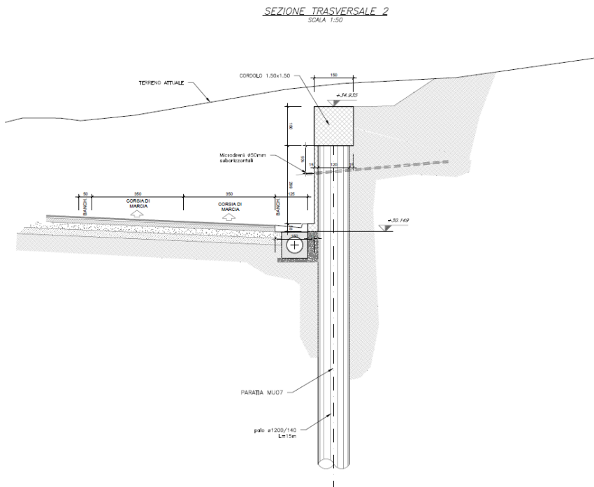
Figura 5: Sezione di progetto "Tipologico n.2"
