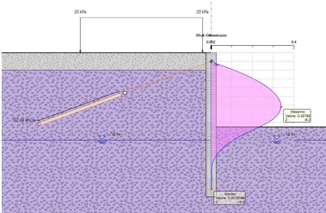
Figura 32 - Verifica tensioni di esercizio nel calcestruzzo
