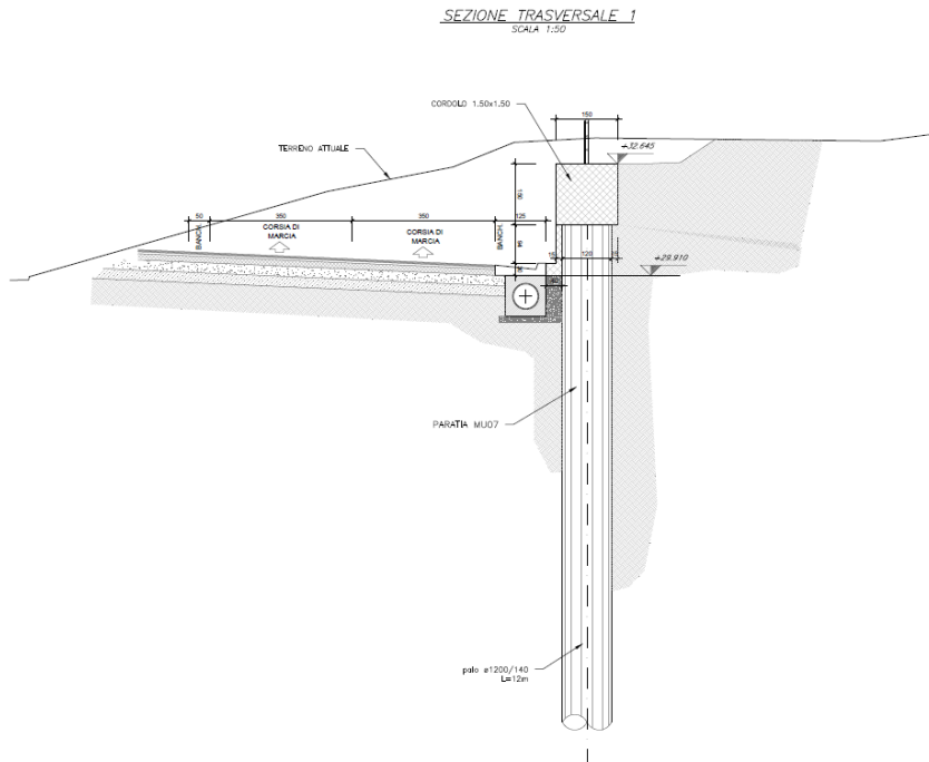
Figura 4: Sezione di progetto "Tipologico n.1"
