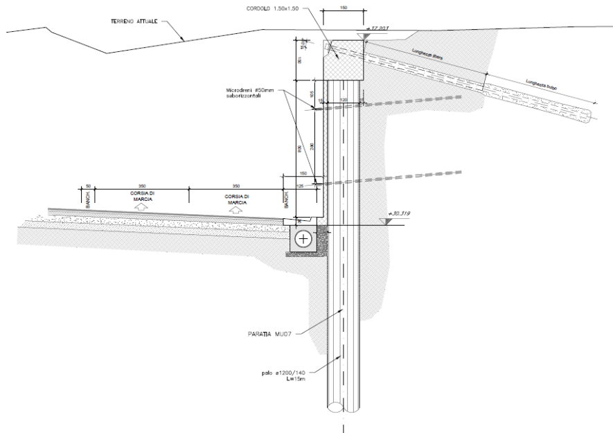
Figura 6: Sezione di progetto “Tipologico n.3”
