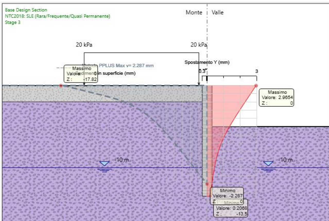
Figura 12 - Involuppo spostamenti allo SLE. |umax|=2.96 mm
