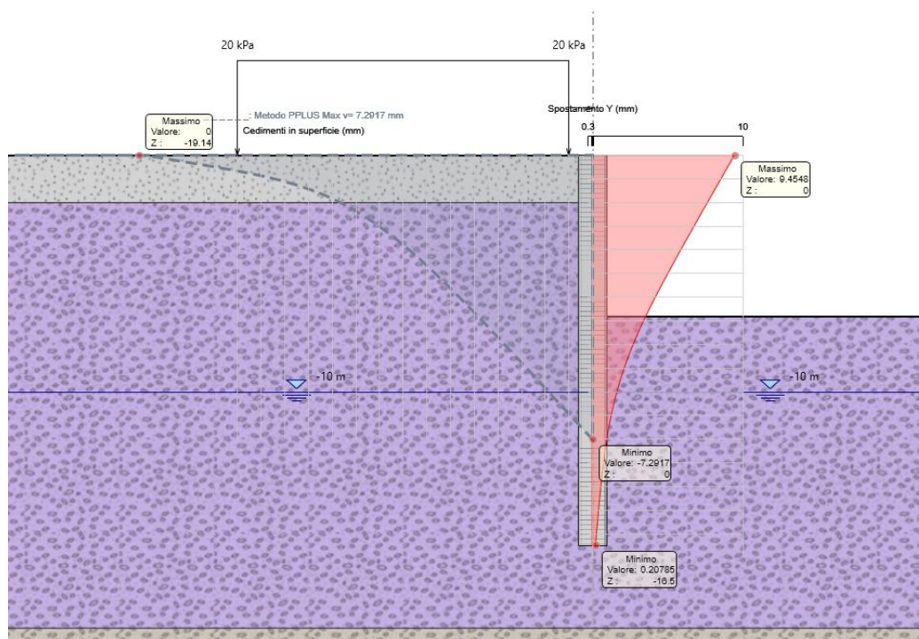
Figura 20 - Involucro spostamenti allo SLE. |umax|=9.46 mm
