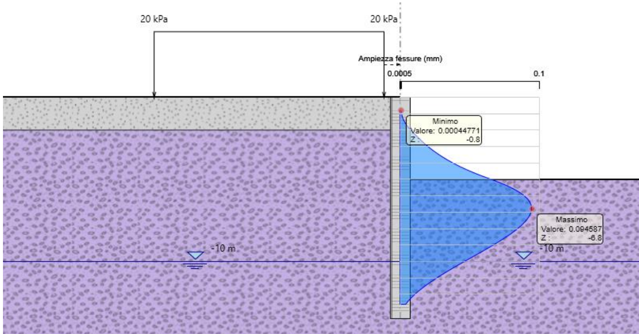
Figura 18 - Verifica a fessurazione SLE
