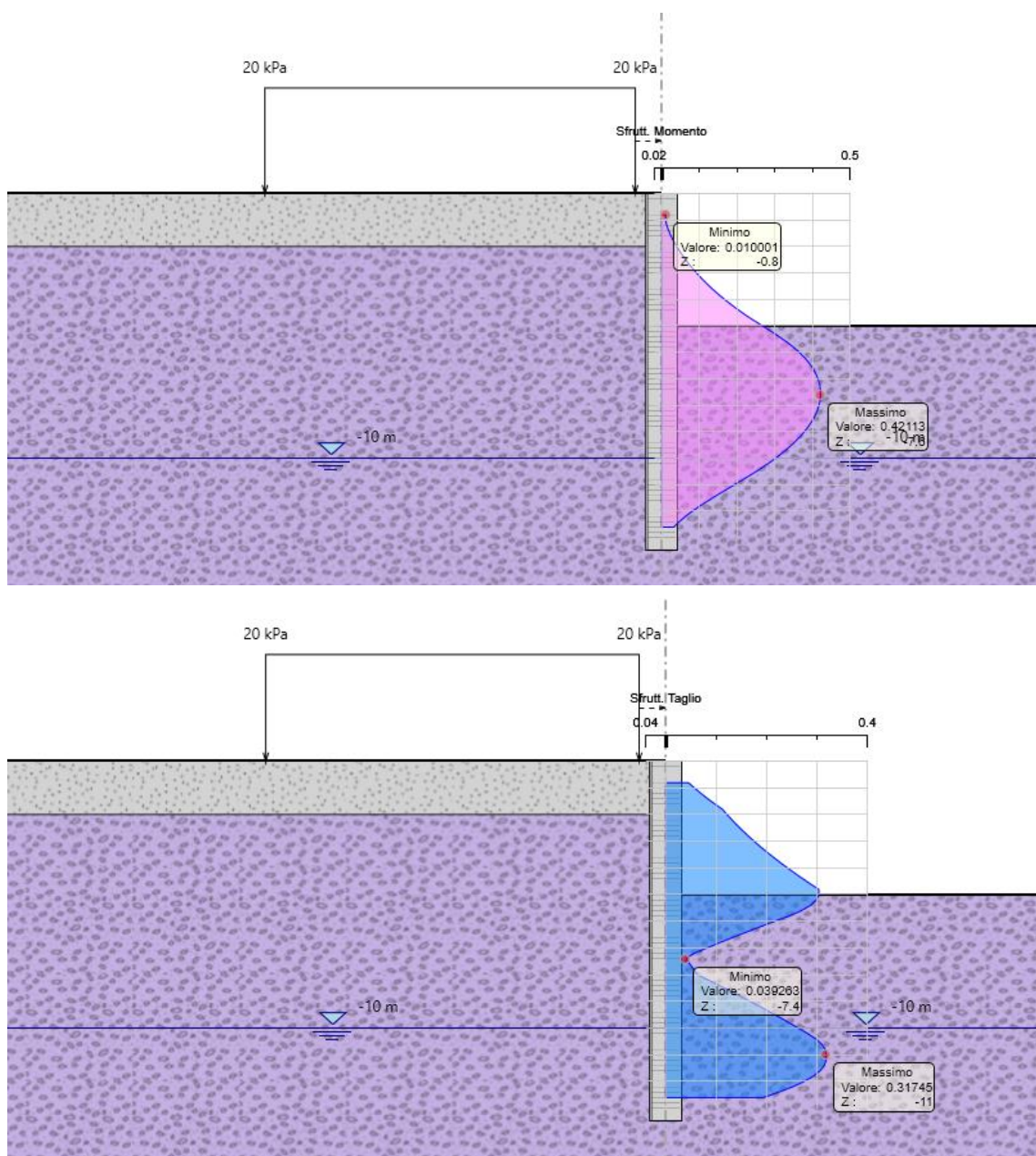
Figura 15 - Verifica strutturale palo SLU
