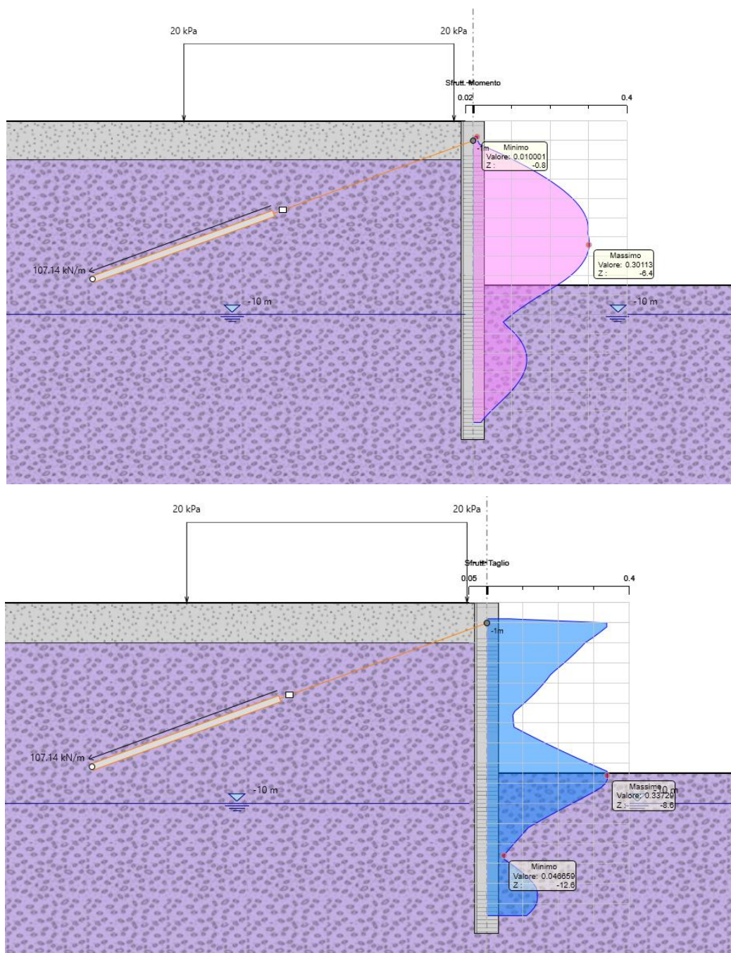
Figura 31 - Verifica strutturale palo SLV
