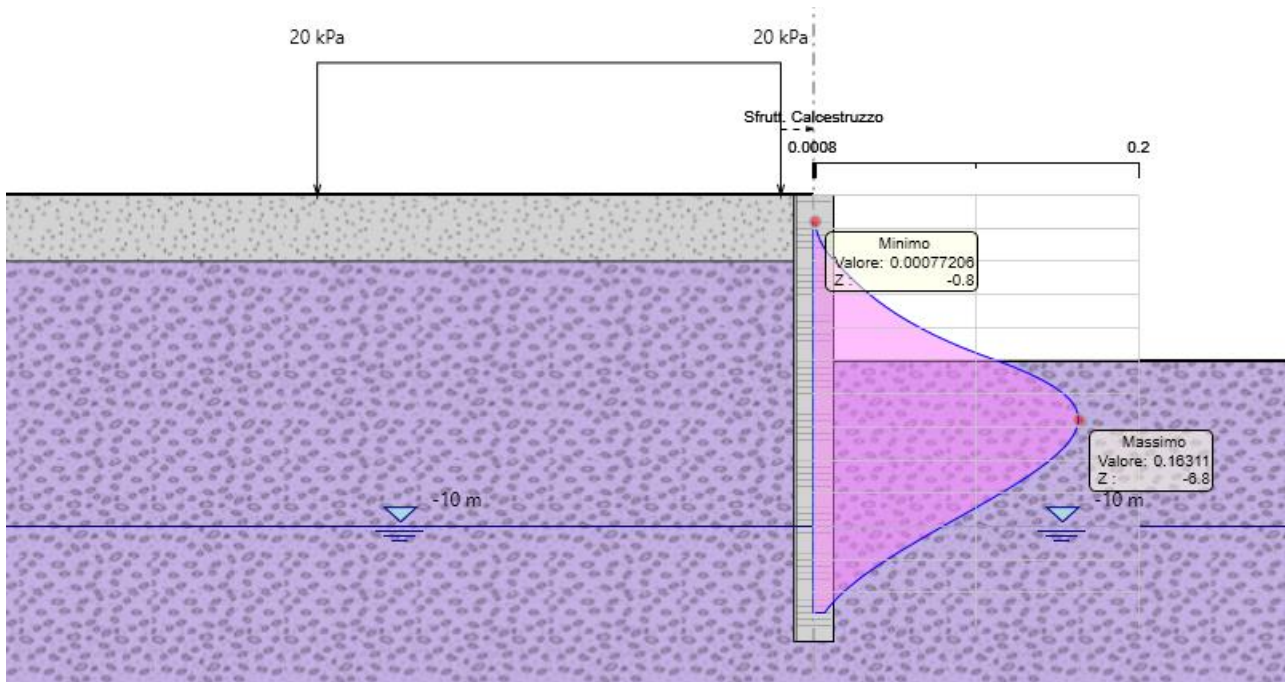
Figura 16 - Verifica tensioni di esercizio nel calcestruzzo
