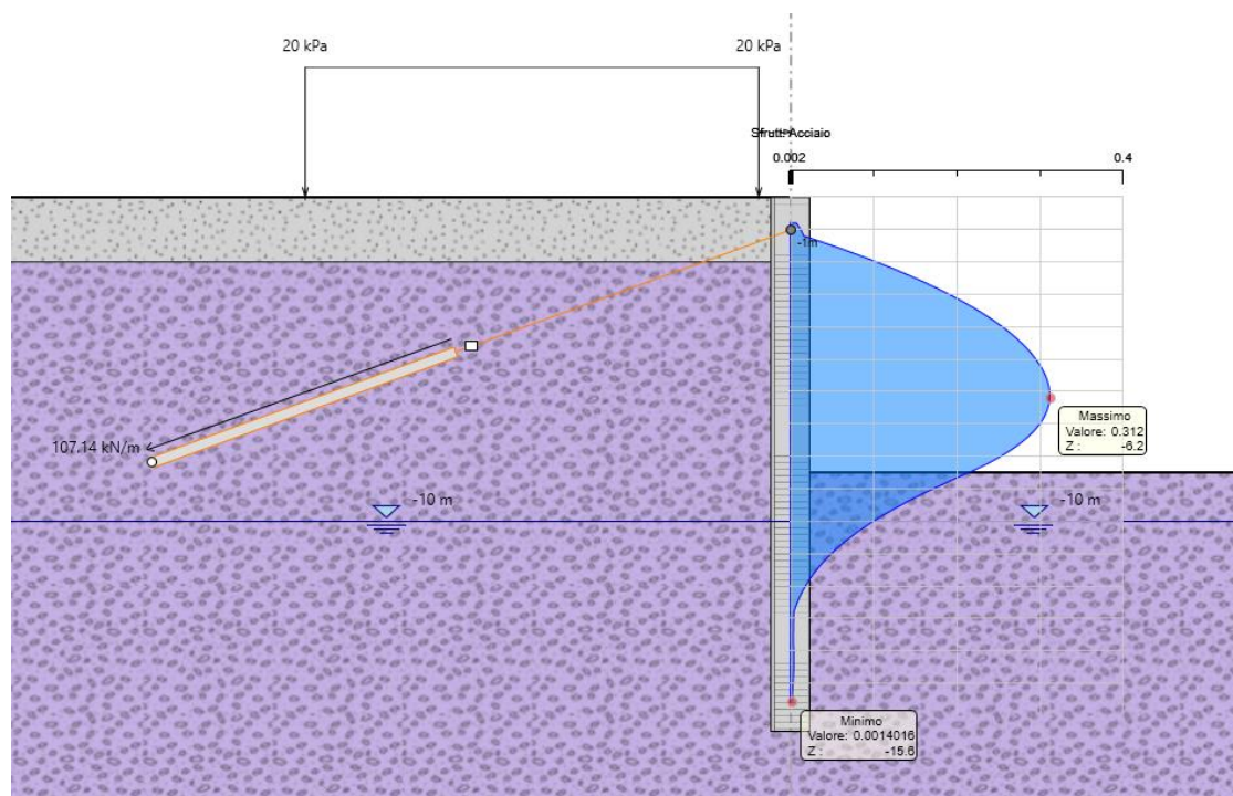
Figura 33 - Verifica tensioni di esercizio nell'acciaio
