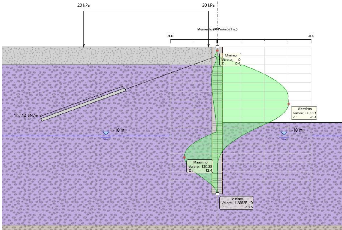
Figura 29 - Involuppo momento flettente
