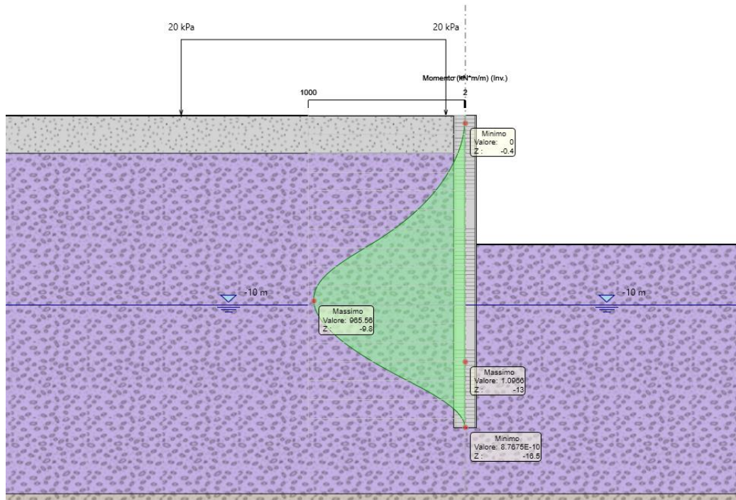
Figura 21 - Inviluppo momento flettente
