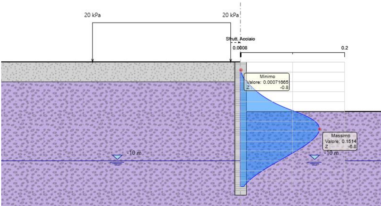
Figura 17 - Verifica tensioni di esercizio nell'acciaio
