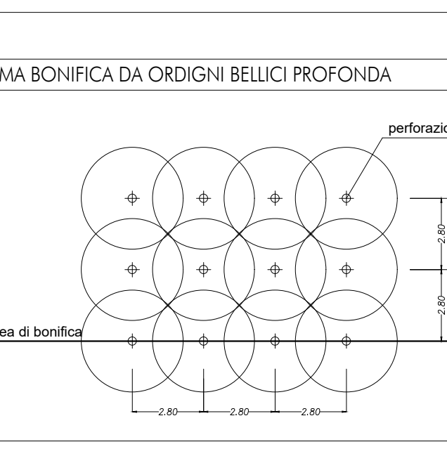
SCHEMA TIPOLOGICO BONIFICA PROFONDA
