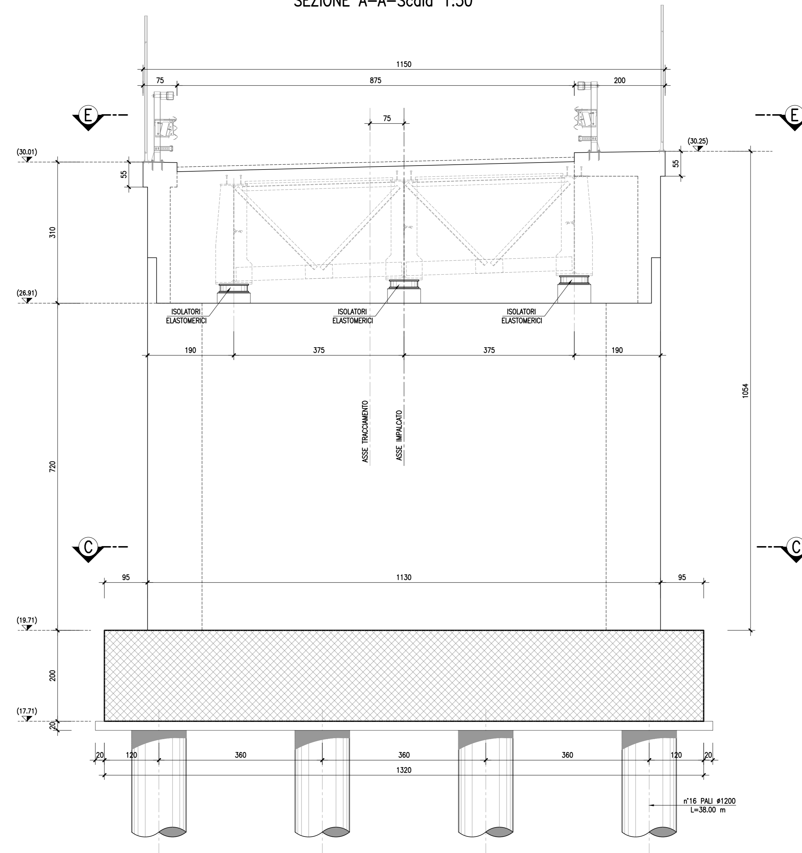
SEZIONE A-A-Scala 1:50
