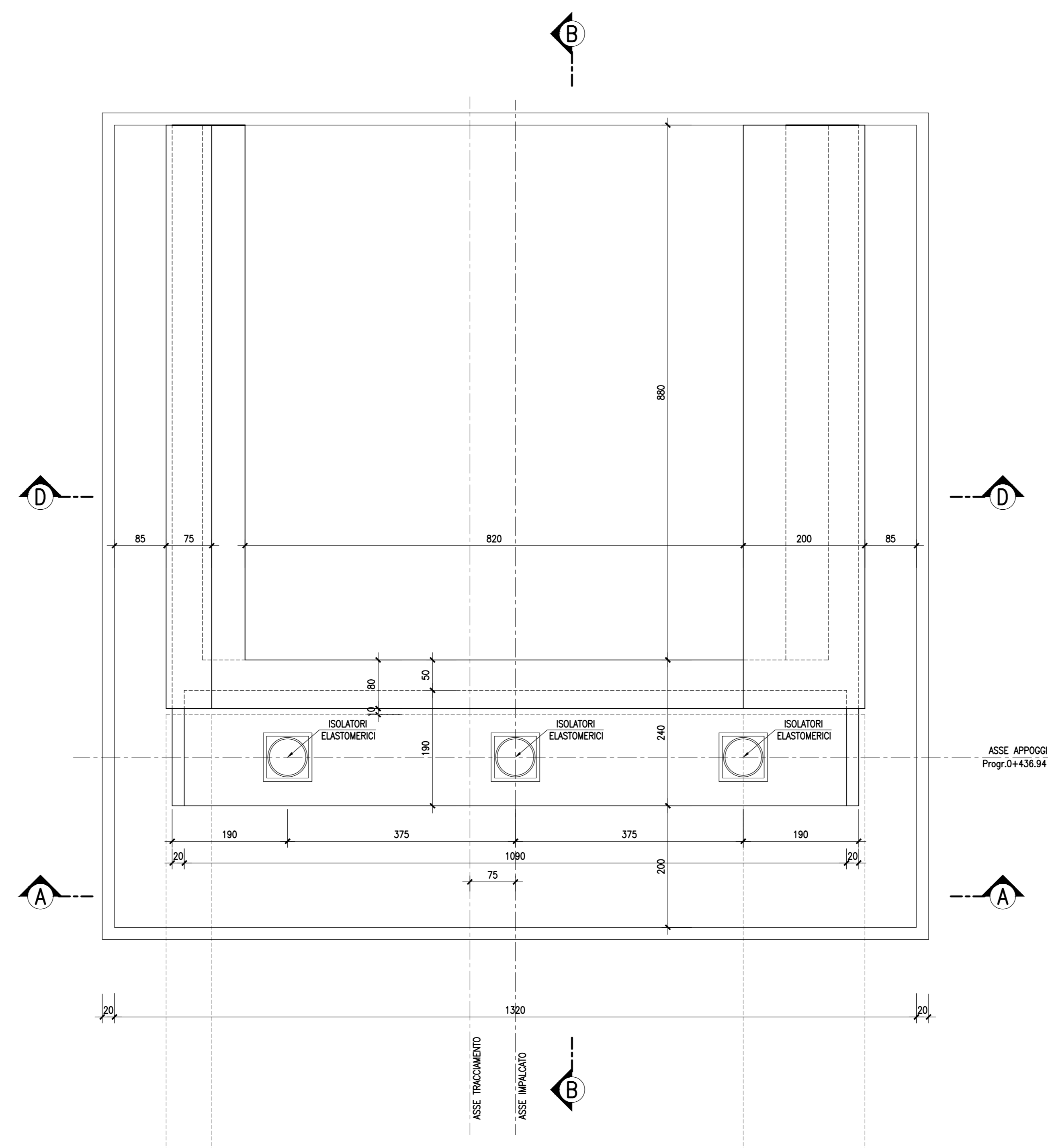
SEZIONE E-E-Scala 1:50
