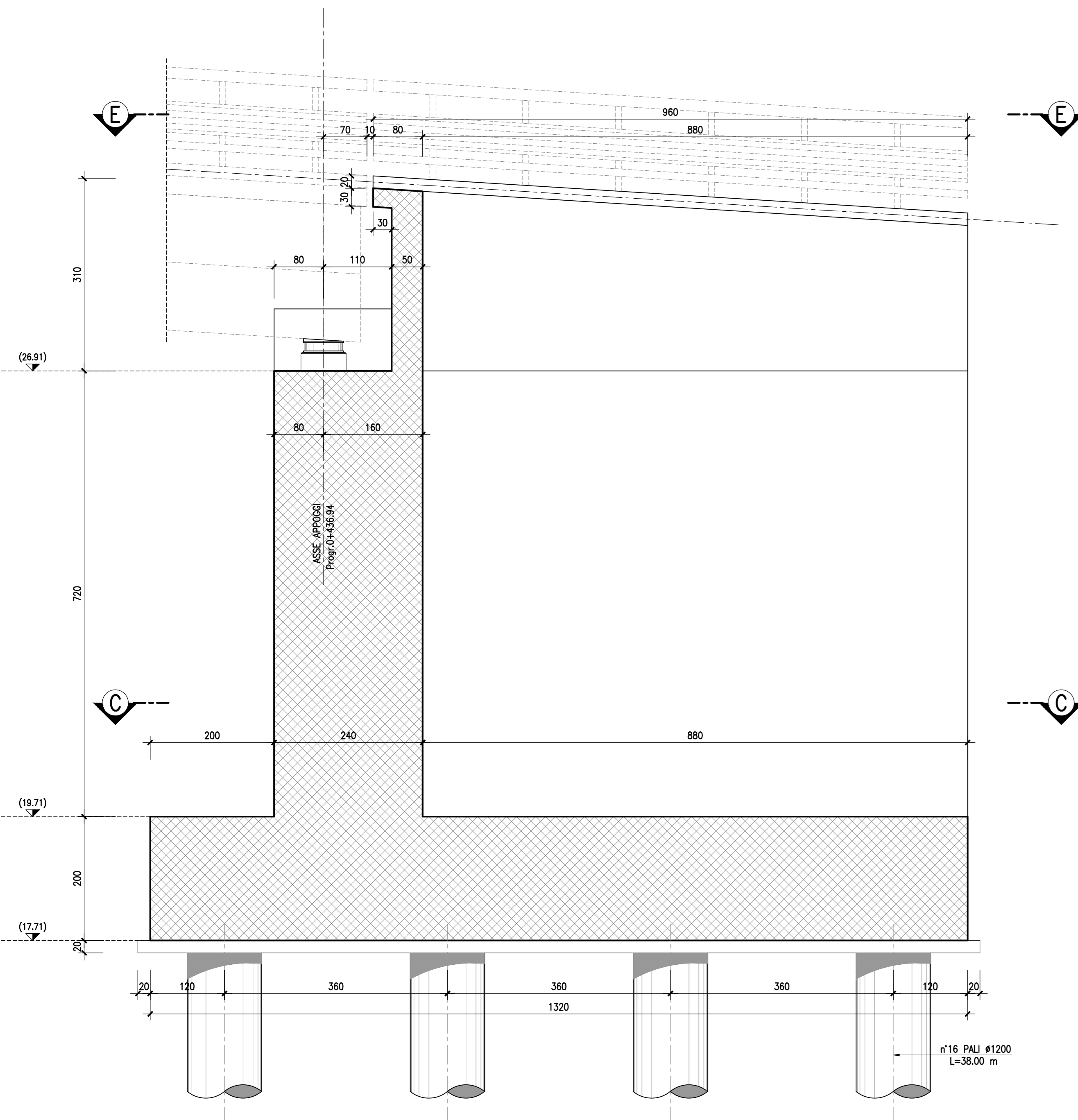
SEZIONE B-B-Scala 1:50
