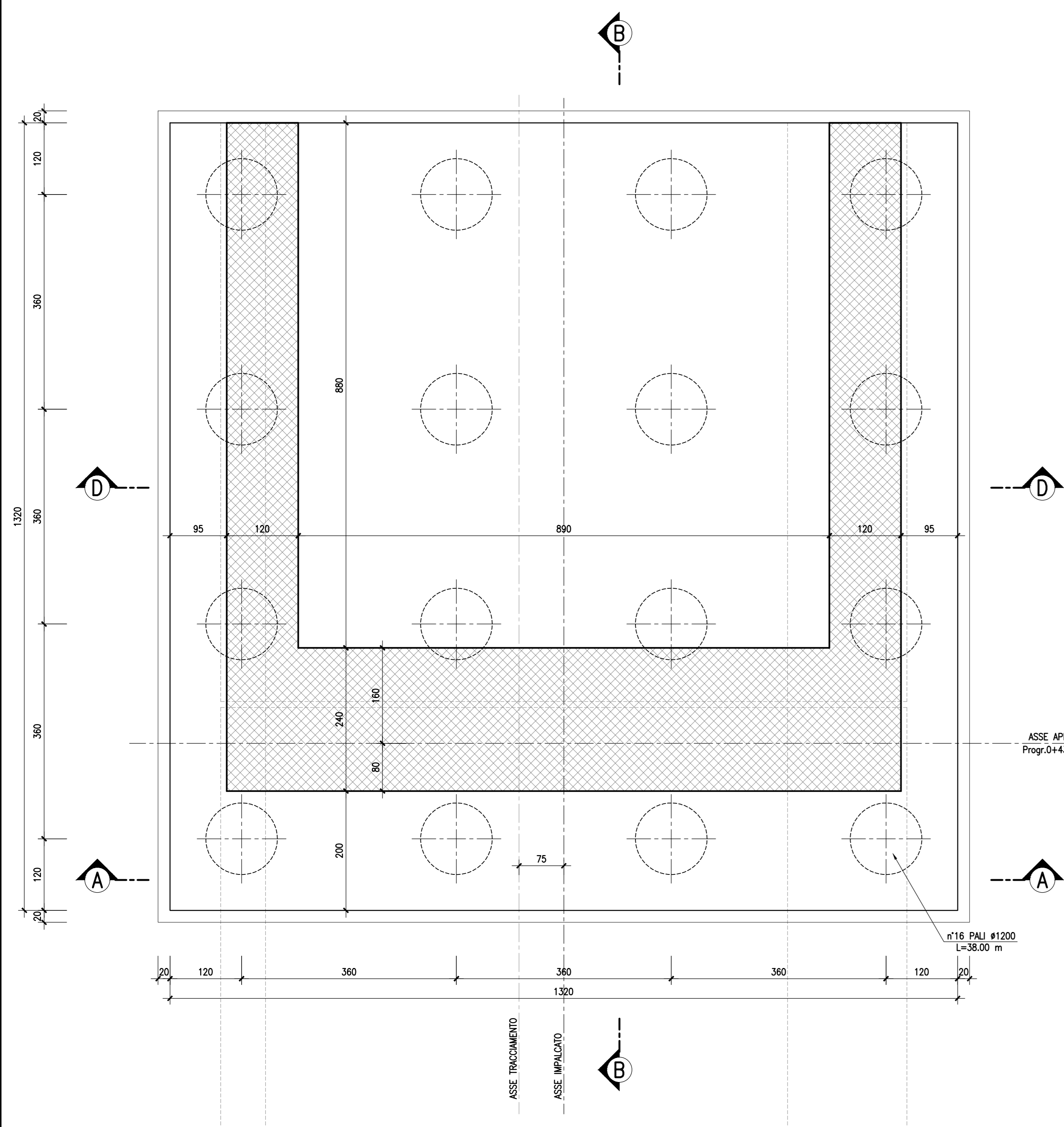
SEZIONE C-C-Scala 1:50
