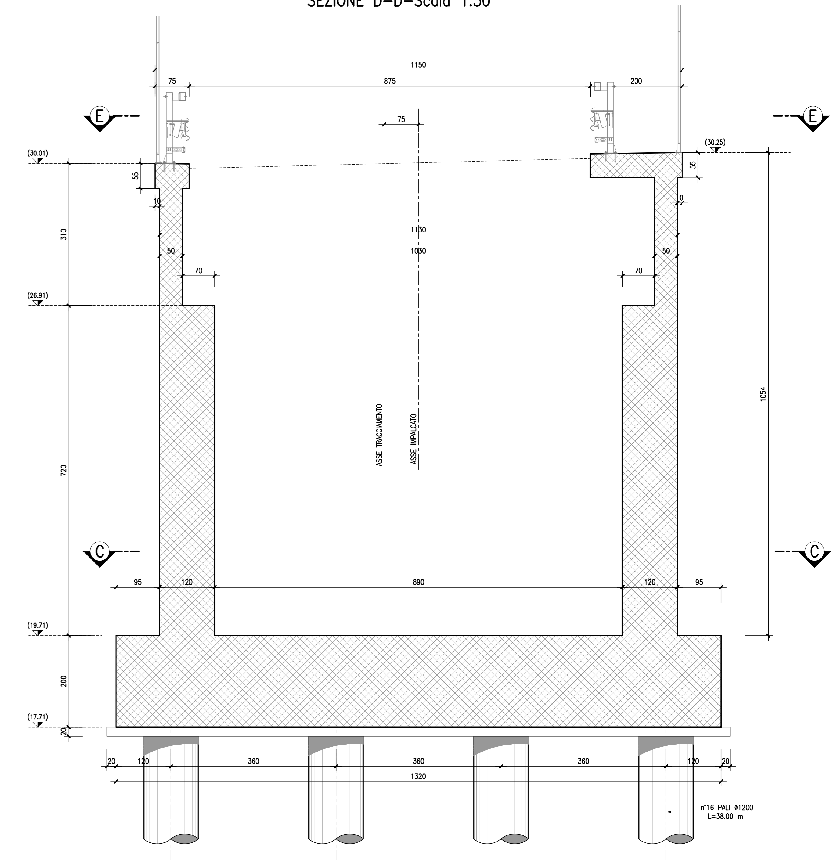
SEZIONE D-D-Scala 1:50
