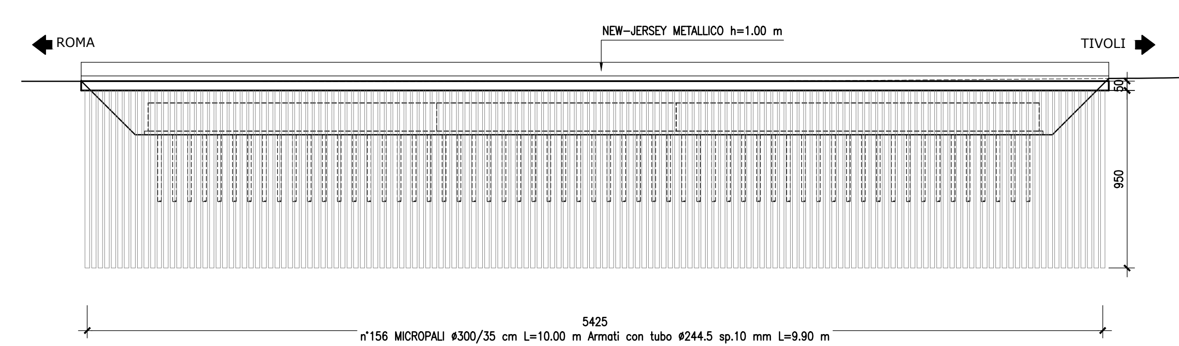
SEZIONE LONGITUDINALE PARATIE PROVISORIE SU VIA TIBURTINA-Scala 1:200
