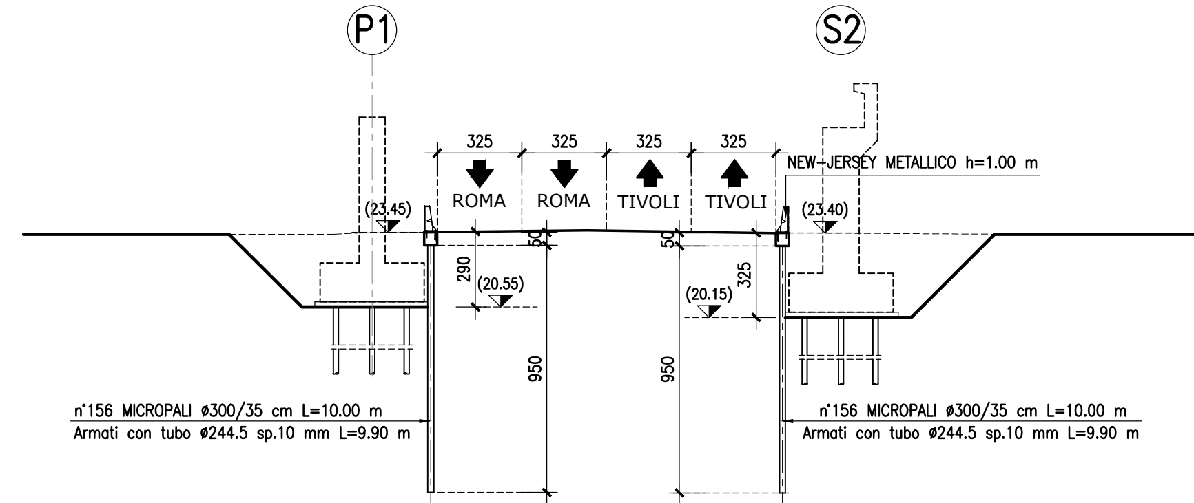
SEZIONE TRASVERSALE PARATIE PROVISORIE SU VIA TIBURTINA-Scala 1:200
