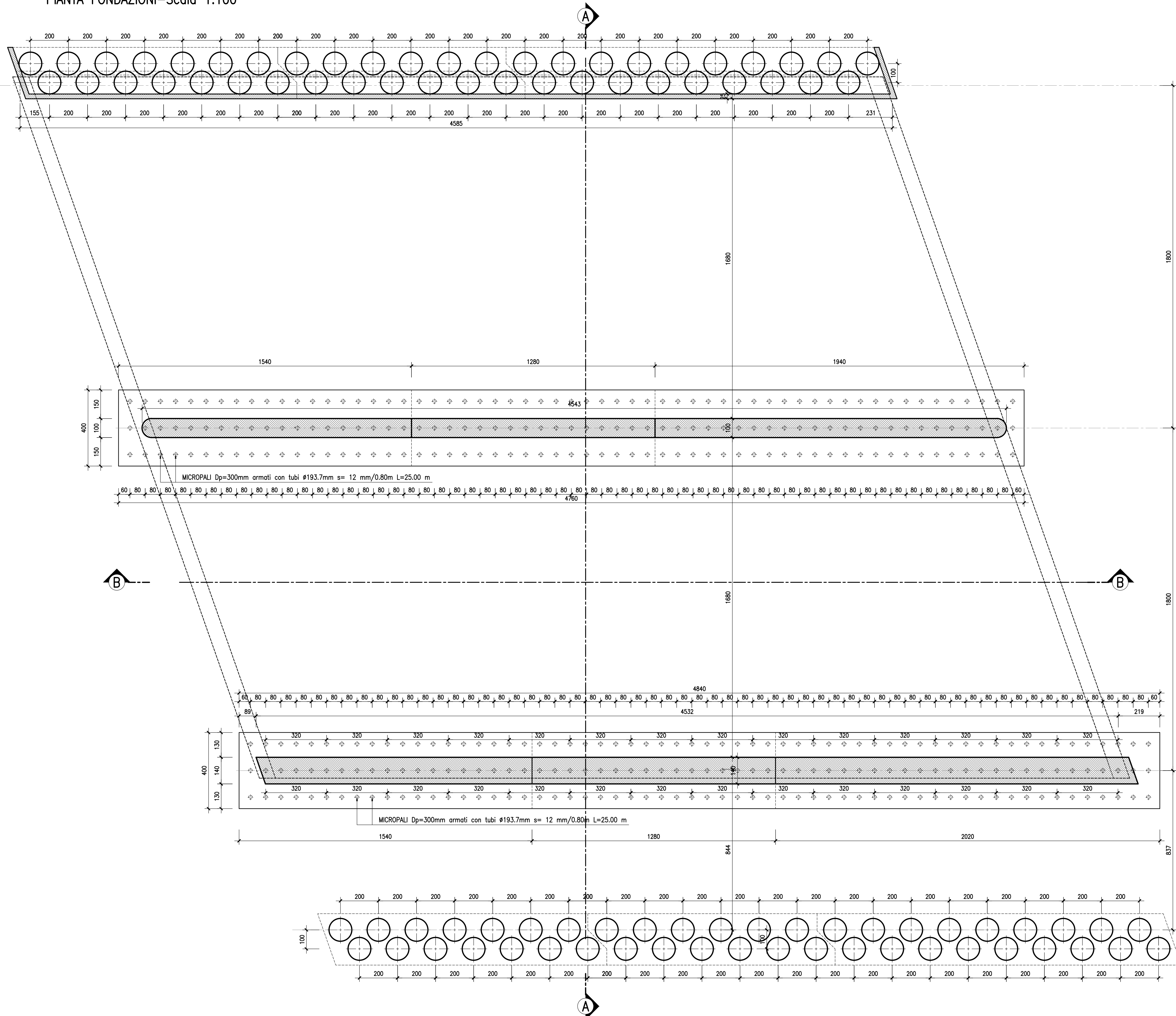
PIANTA FONDAZIONI-Scala 1:100
