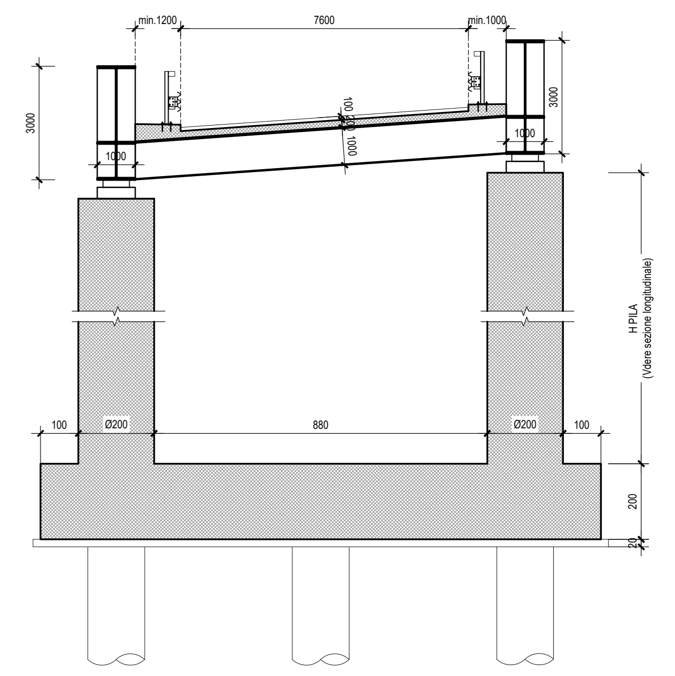
SEZIONE TRASVERSALE TIPO-Scala 1:100
