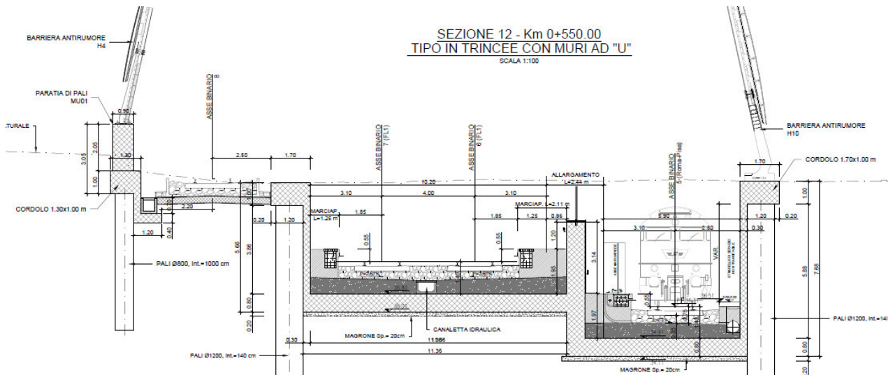
TR05: Sezione trincea con più binari
