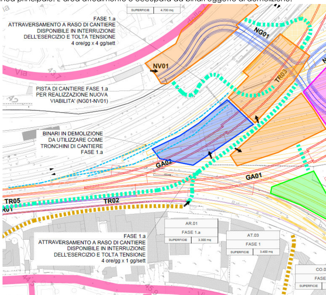
Vista planimetrica dell'area AR.01 (Fase 1)
