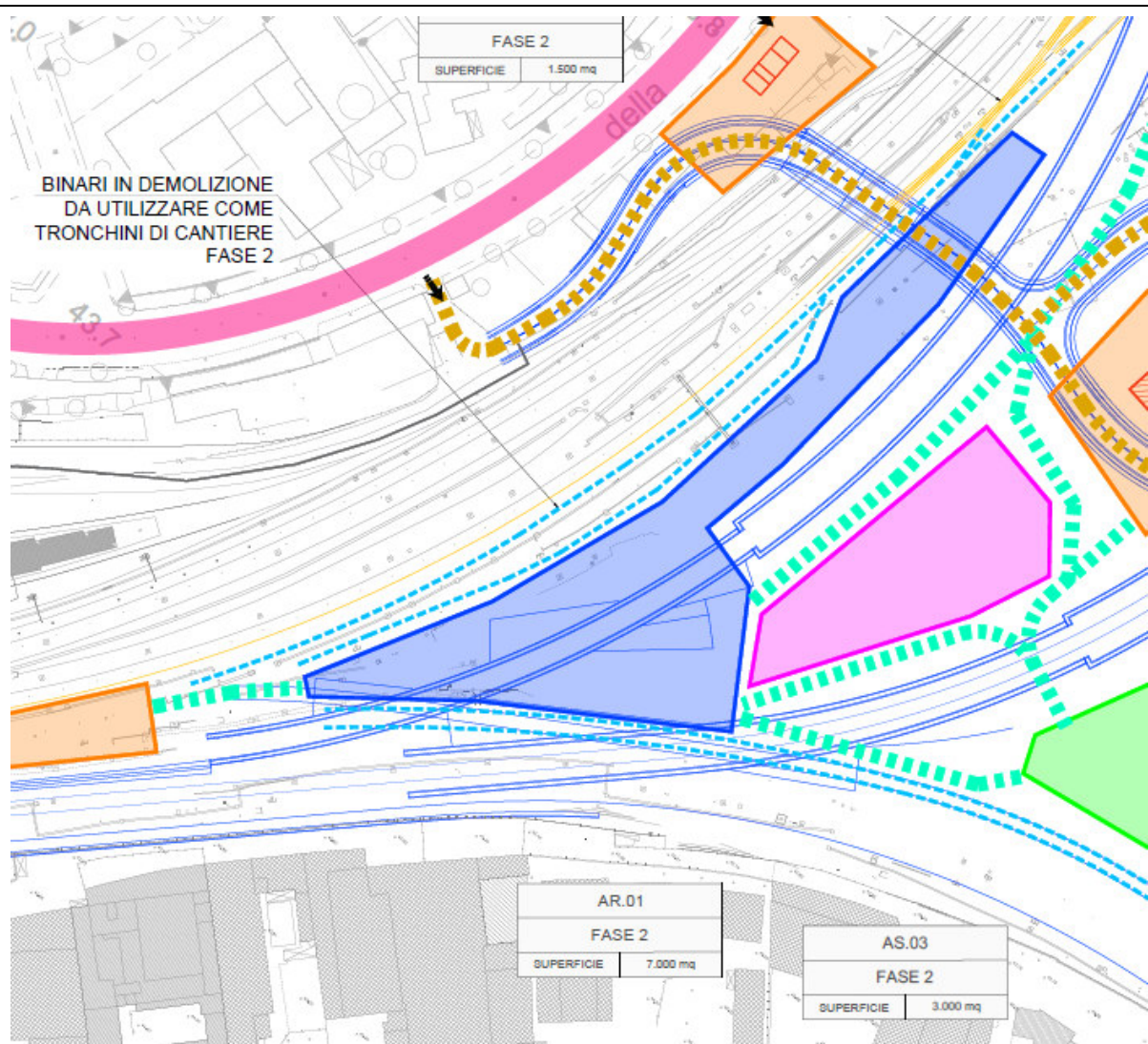
Vista planimetrica dell'area AR.01 (Fase 2)
