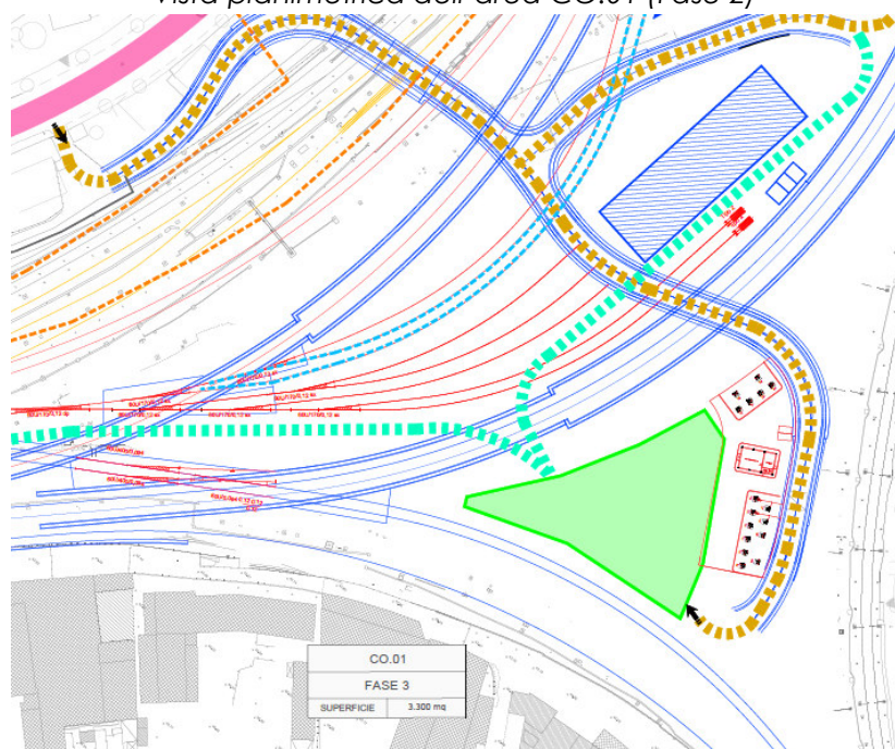
Vista planimetrica dell'area CO.01 (Fase 3) – realizzazione Cabina TE
