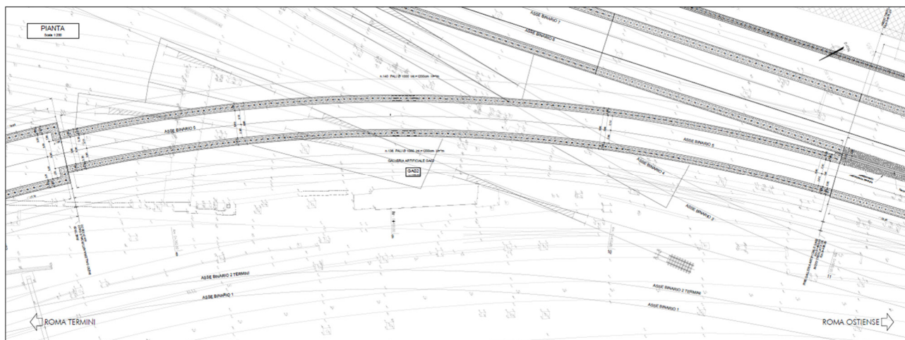
Pianta della galleria artificiale GA02
