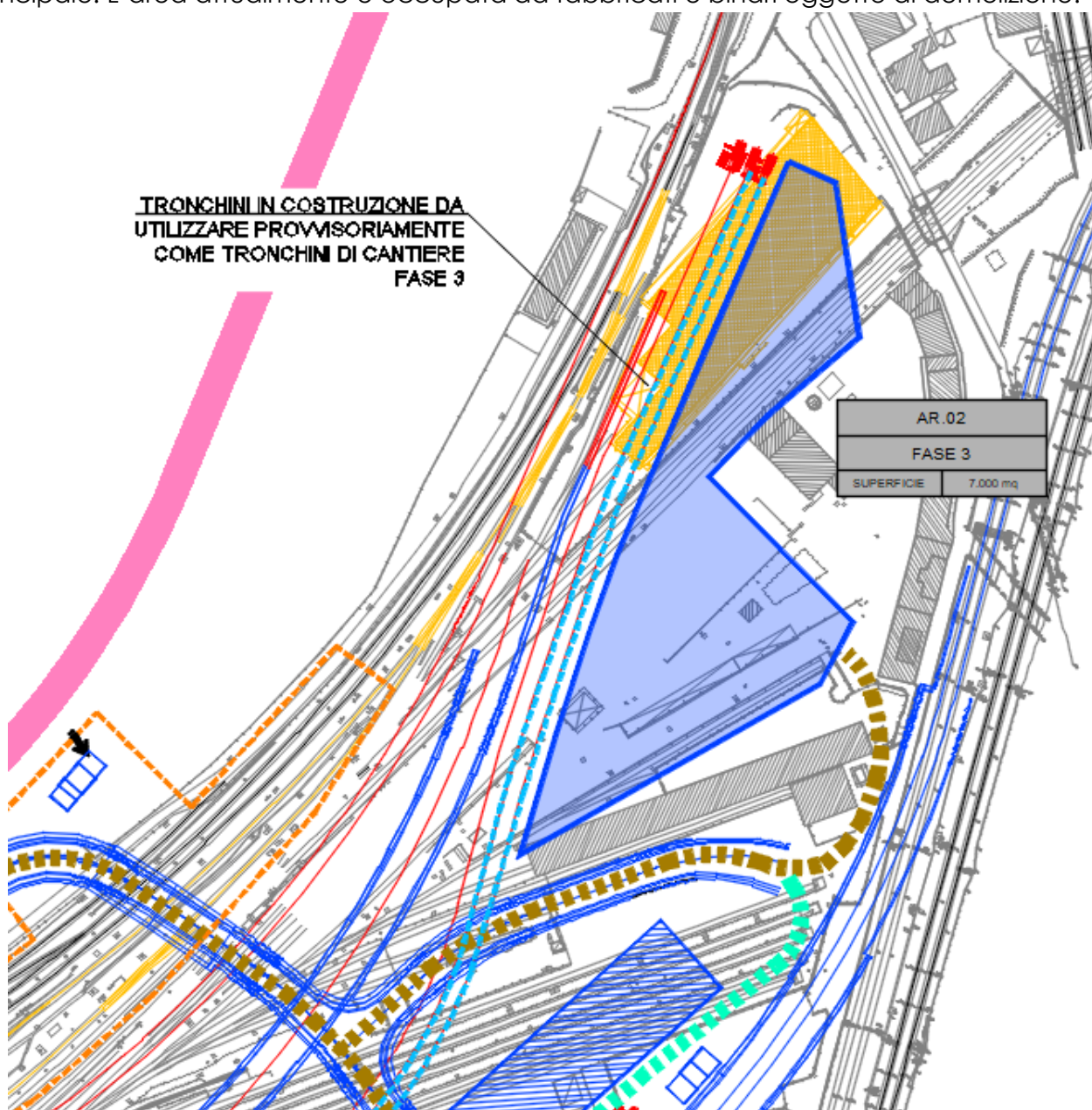
Vista planimetrica dell'area AR.02 (Fase 3)
