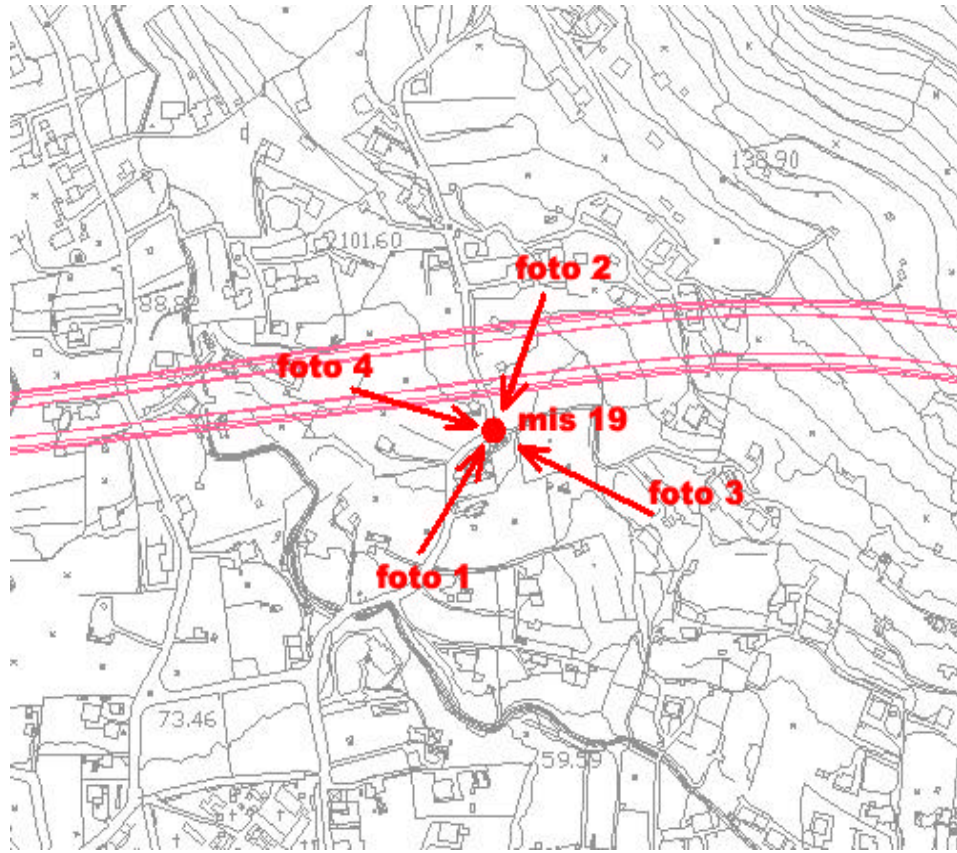
Stralcio planimetrico
