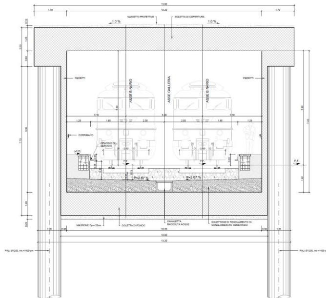
Sezioni GA01
