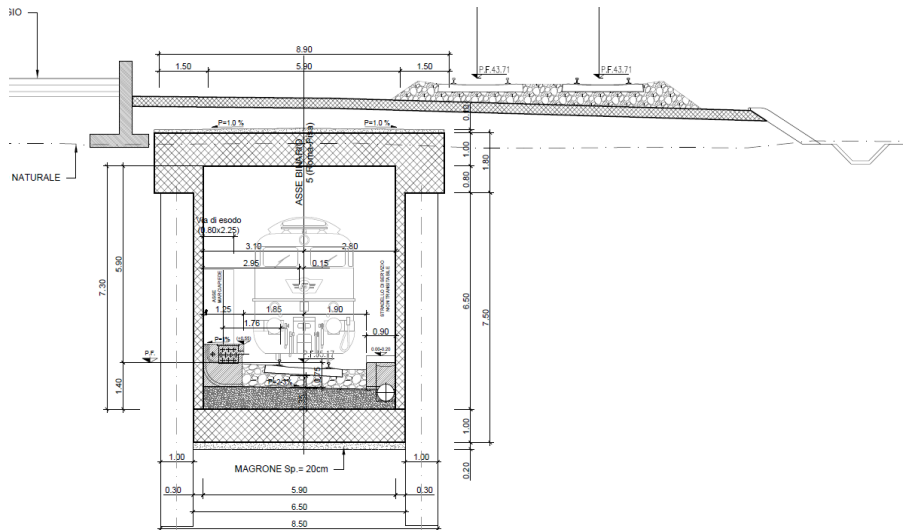
Sezioni GA02
