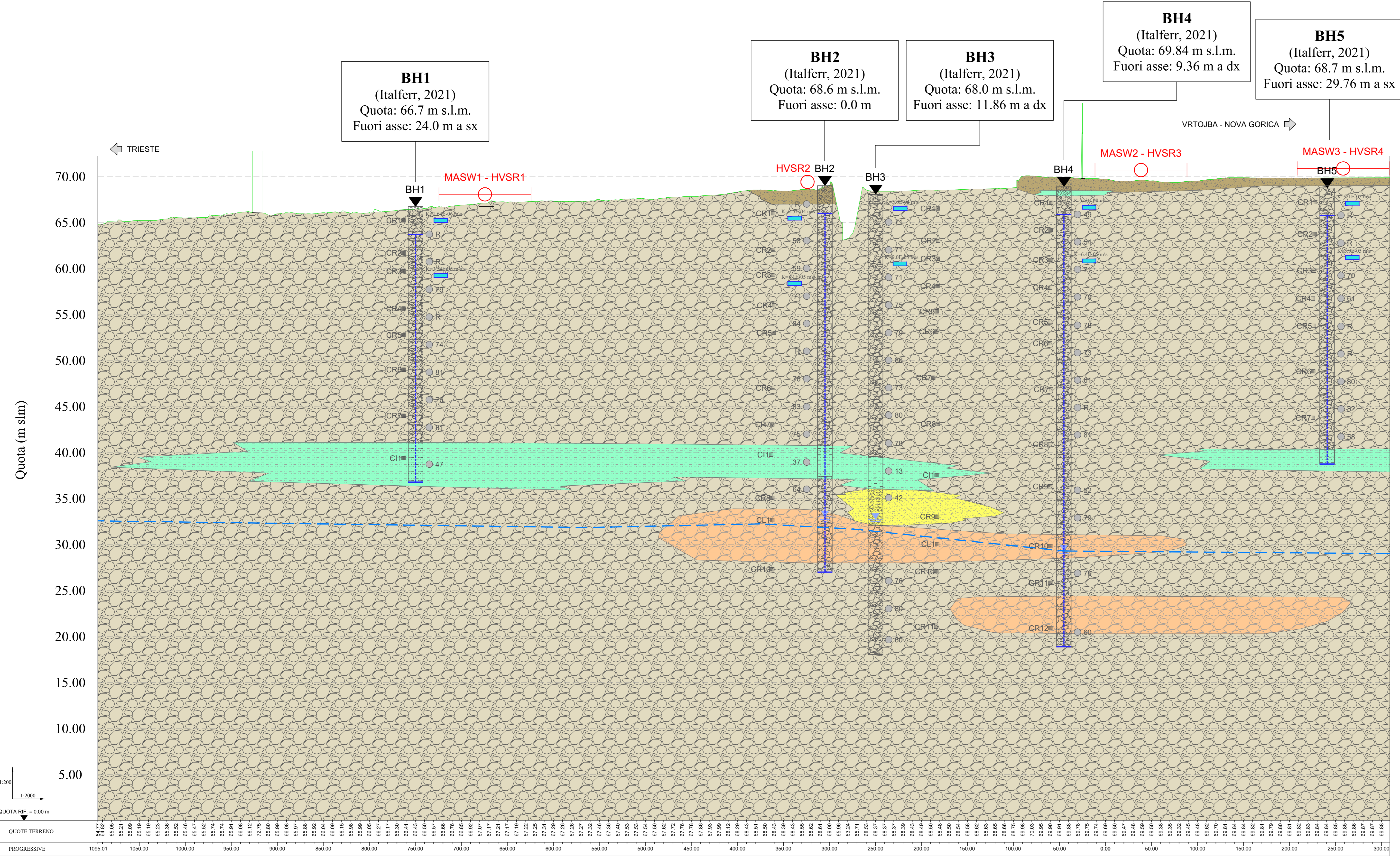
PROFILO GEOLOGICO SCALA 1:2000
