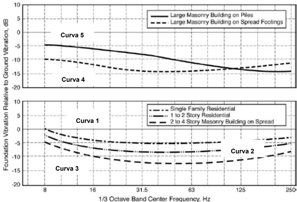
Figura 5-10 Fattori correttivi dovuti alla tipologia di fondazione
