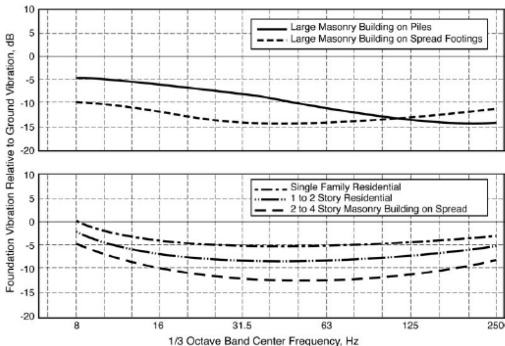
Figura 5-7 Risposta delle fondazioni per diverse tipologie di edifici (Fonte: FTA, USA)
