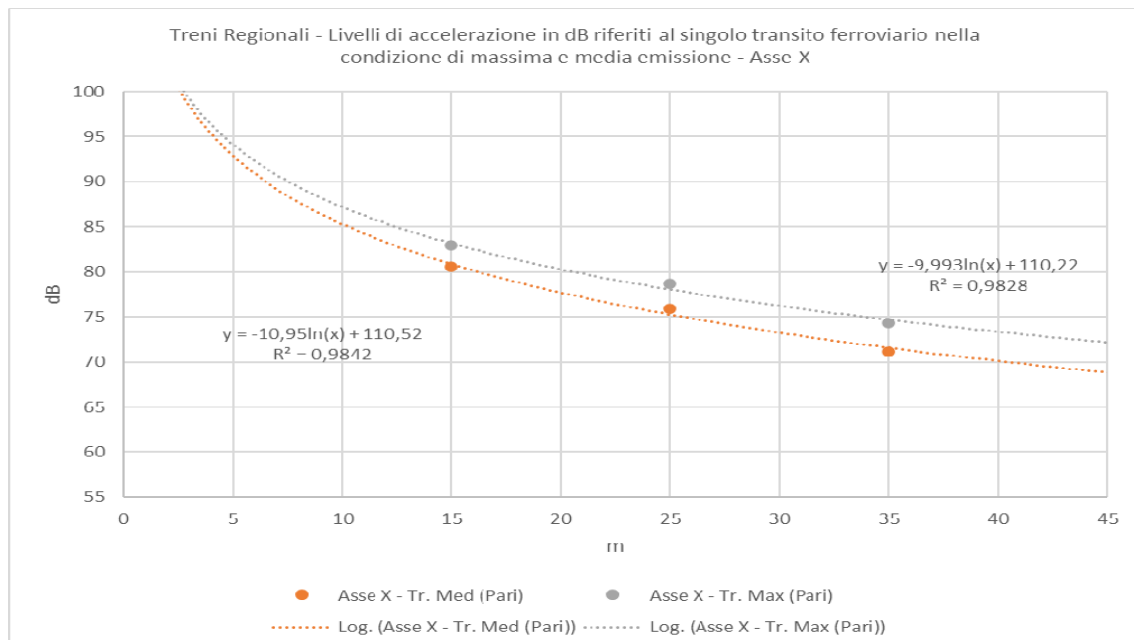
Figura 5-4 Individuazione della legge di propagazione delle vibrazioni nel terreno sulla base dei dati sperimentali lungo l'asse X per un singolo transito ferroviario di treno regionale nella condizione di massima e media emissione.
