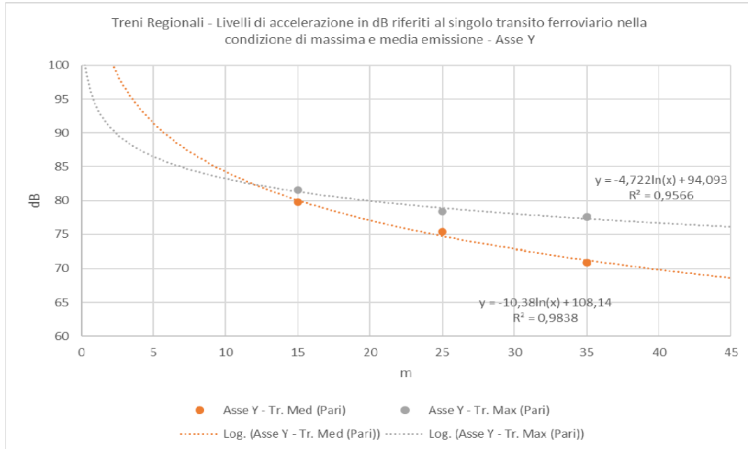
Figura 5-5 Individuazione della legge di propagazione delle vibrazioni nel terreno sulla base dei dati sperimentali lungo l'asse Y per un singolo transito ferroviario di treno regionale nella condizione di massima e media emissione.
