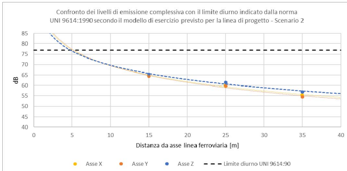
Figura 6-4 Confronto dei livelli di emissione complessiva all'interno degli edifici con i limiti UNI 9614:1990 in funzione della distanza dal binario secondo il modello di esercizio previsto – Periodo diurno, Scenario 2.
