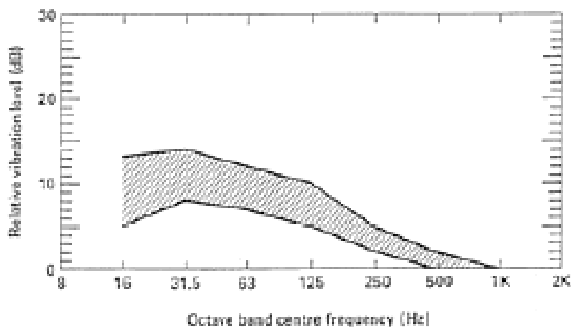
Figura 5-9 Amplificazione prodotta dai solai
