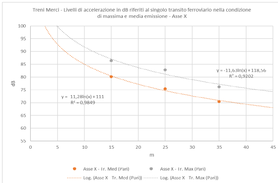
Figura 5-1 Individuazione della legge di propagazione delle vibrazioni nel terreno sulla base dei dati sperimentali lungo l'asse X per un singolo transito ferroviario di treno merci nella condizione di massima e media emissione.
