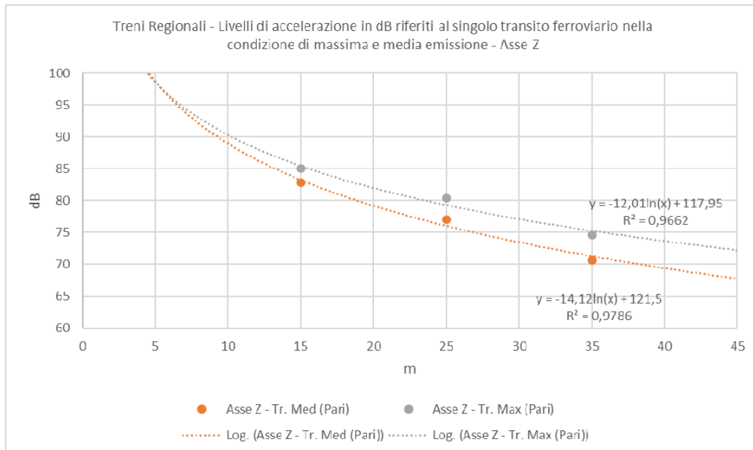
Figura 5-6 Individuazione della legge di propagazione delle vibrazioni nel terreno sulla base dei dati sperimentali lungo l'asse Z per un singolo transito ferroviario di treno regionale nella condizione di massima e media emissione.
