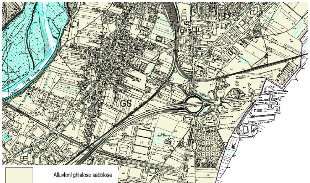
Figura 3-2 Stralcio non in scala della Carta Geologica del Comune di Gorizia realizzata in scala 1:10.000.
