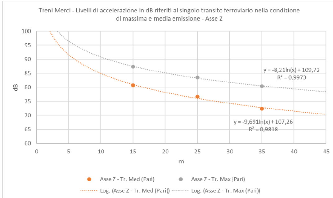
Figura 5-3 Individuazione della legge di propagazione delle vibrazioni nel terreno sulla base dei dati sperimentali lungo l'asse Z per un singolo transito ferroviario di treno merci nella condizione di massima e media emissione.
