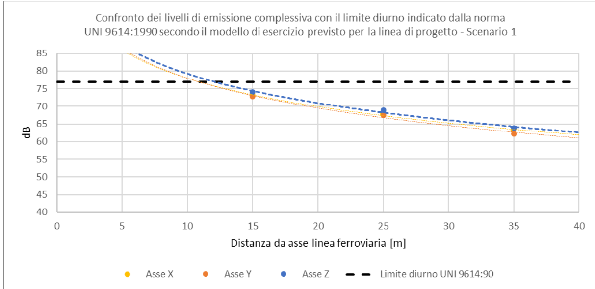
Figura 6-2 Confronto dei livelli di emissione complessiva all'interno degli edifici con i limiti UNI 9614:1990 in funzione della distanza dal binario secondo il modello di esercizio previsto – Periodo diurno, Scenario 1.
