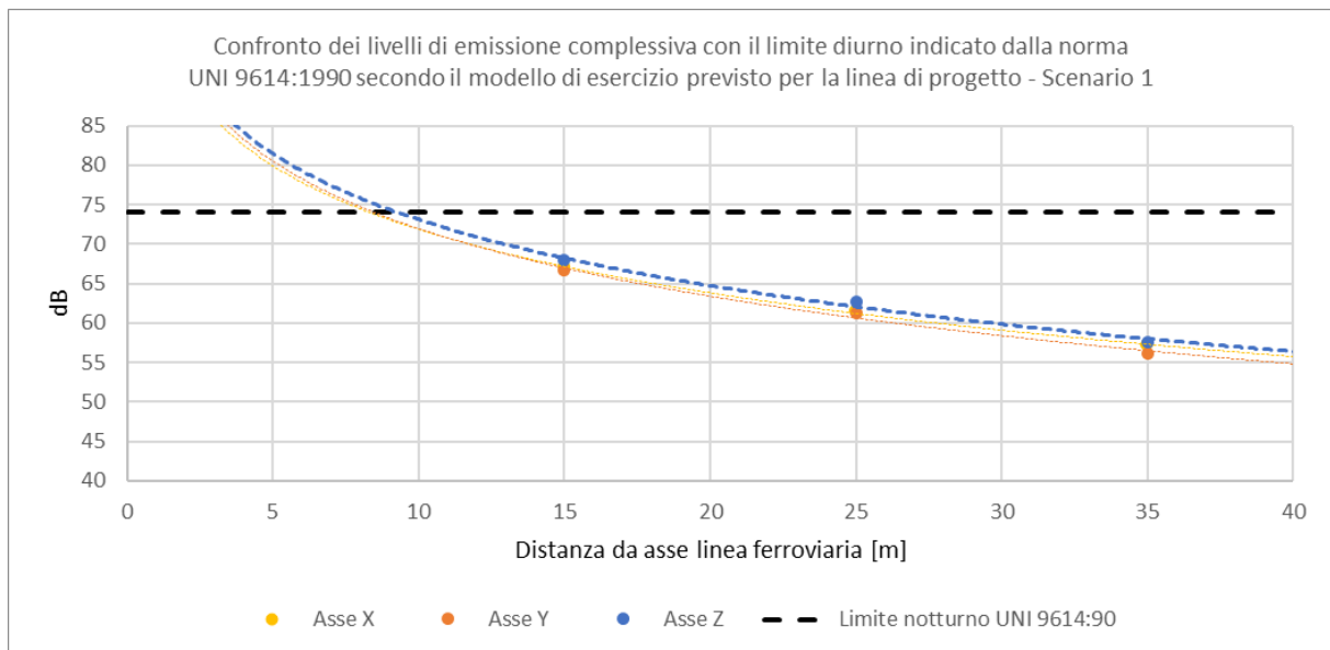
Figura 6-3 Confronto dei livelli di emissione complessiva all'interno degli edifici con i limiti UNI 9614:1990 in funzione della distanza dal binario secondo il modello di esercizio previsto – Periodo notturno, Scenario 1.
