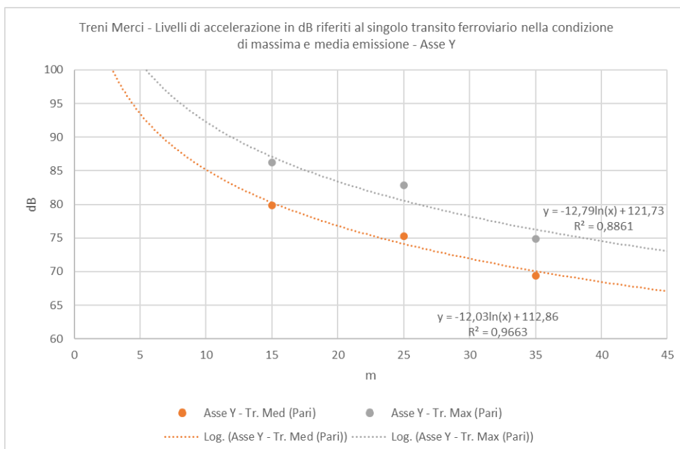
Figura 5-2 Individuazione della legge di propagazione delle vibrazioni nel terreno sulla base dei dati sperimentali lungo l'asse Y per un singolo transito ferroviario di treno merci nella condizione di massima e media emissione.
