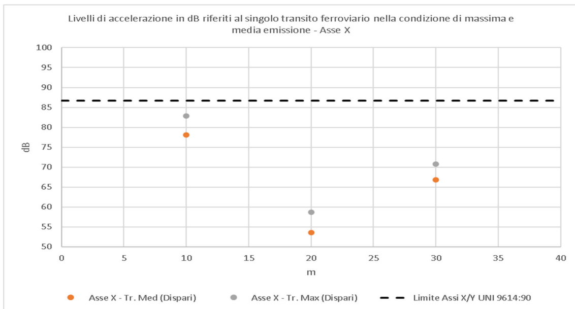
Figura 1-10 Livelli di accelerazione lungo l'asse X rappresentativi delle condizioni di massima e media emissione di un singolo transito ferroviario sul binario dispari a 10, 20 e 30 m dall'asse del binario e confronto con il livello limite per gli assi X e Y della UNI 9614:1990 per i singoli transiti ferroviari (appendice A4)
