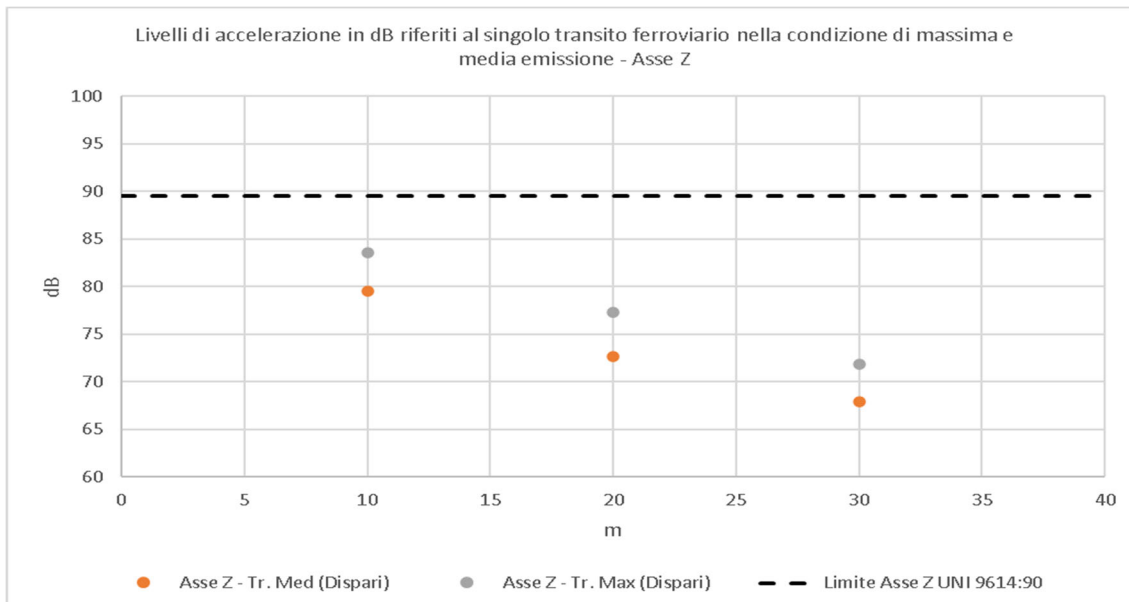
Figura 1-12 Livelli di accelerazione lungo l'asse Z rappresentativi delle condizioni di massima e media emissione di un singolo transito ferroviario sul binario dispari a 10, 20 e 30 m dall'asse del binario e confronto con il livello limite per l'asse Z della UNI 9614:1990 per i singoli transiti ferroviari (appendice A4)
