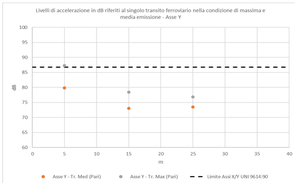
Figura 1-8 Livelli di accelerazione lungo l'asse Y rappresentativi delle condizioni di massima e media emissione di un singolo transito ferroviario sul binario pari a 5, 15 e 25 m dall'asse del binario e confronto con il livello limite per gli assi X e Y della UNI 9614:1990 per i singoli transiti ferroviari (appendice A4)
