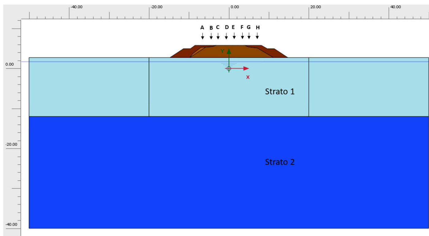
Figura 8.4: Schema rappresentativo sezione
