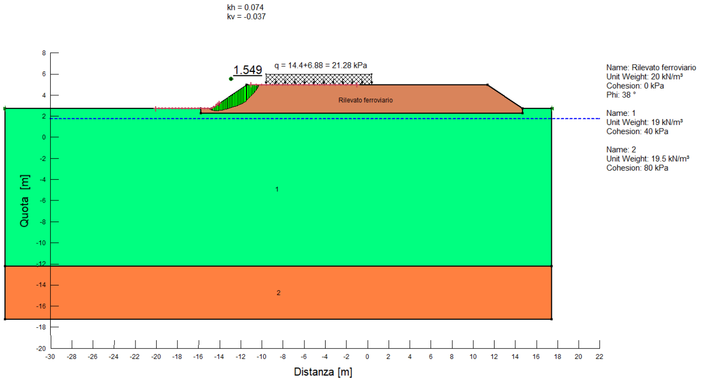
Figura 8.3: Analisi di stabilità globale in campo sismico. Condizioni non drenate
