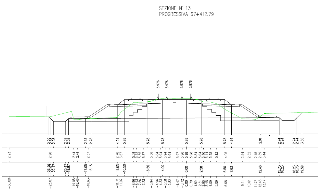
Figura 7.1: - Stralcio di sezione del rilevato del PM in corrispondenza della maggiore altezza
