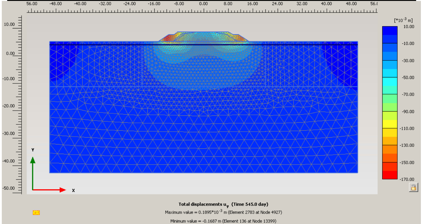
Figura 8.6: Spostamenti verticali termine costruzione
