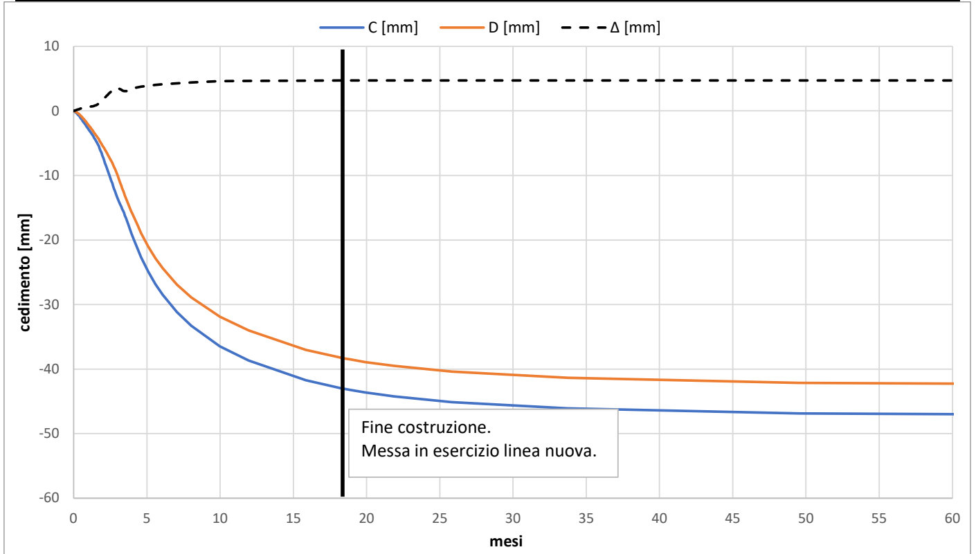
Figura 8.11: Andamento cedimenti nel tempo sulle rotaie dei binari della linea esistente (lato C-D)
