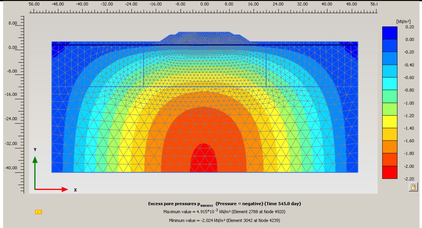
Figura 8.8: Sovrappressioni interstiziali \Delta u termine costruzione
