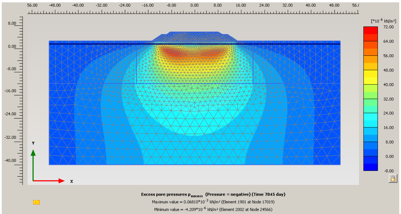
Figura 8.8: Sovrappressioni interstiziali \Delta u termine costruzione
