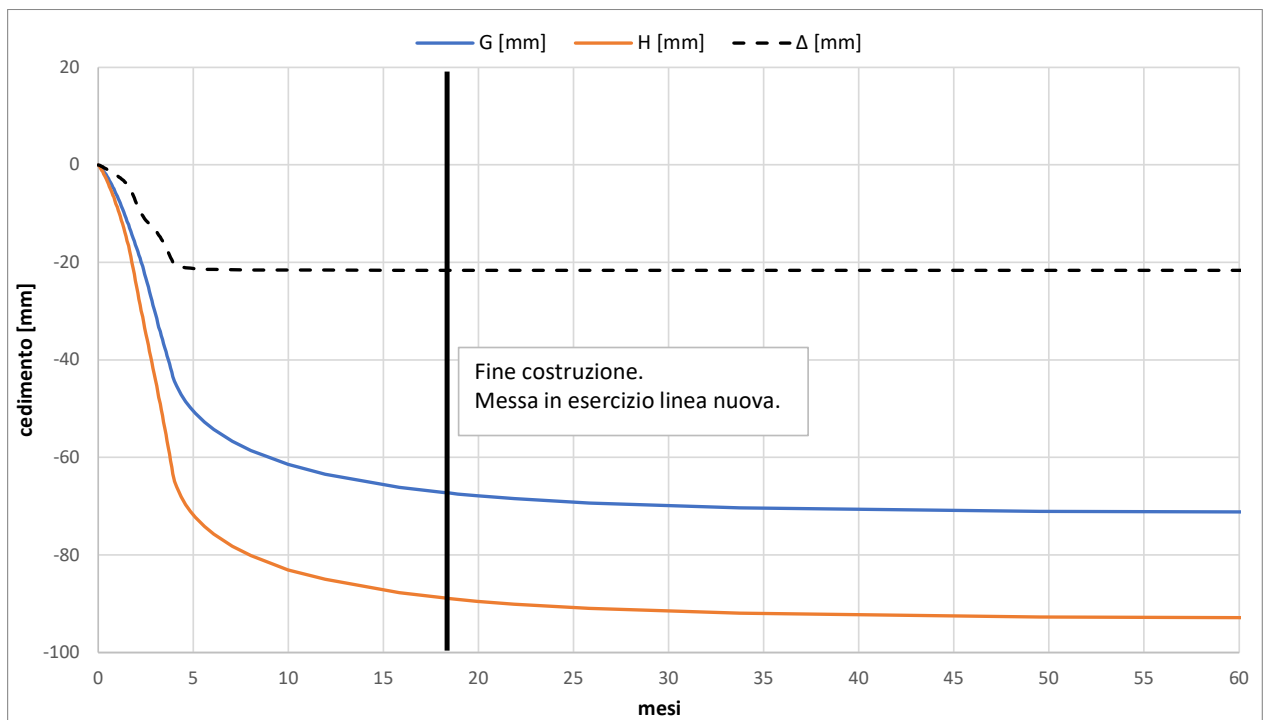
Figura 8.10: Andamento cedimenti nel tempo sulle rotaie dei binari della nuova linea
