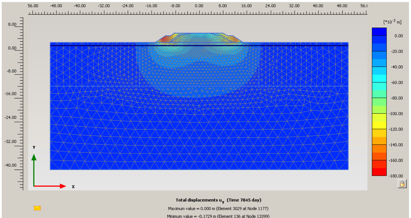
Figura 8.7: Spostamenti verticali lungo termine
