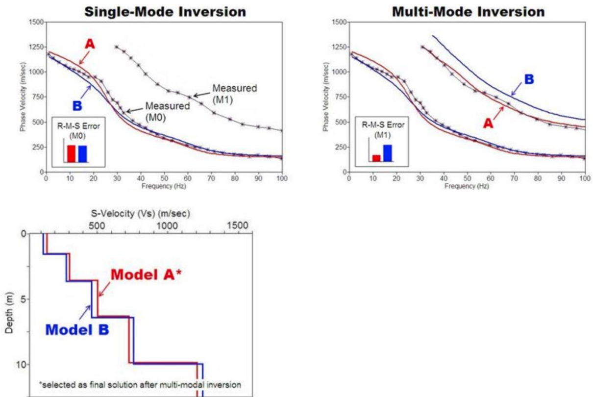
Figura 4.4 – Inversione dei dati (Curva di dispersione con picking – Log V_s )
