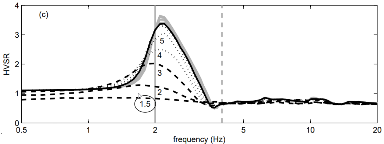
Figura 3.3 - Variazione del rapporto HVSR-Frequenza al variare dell'impedenza sismica (1.5-2.0-3.0-4.0-5.0)
