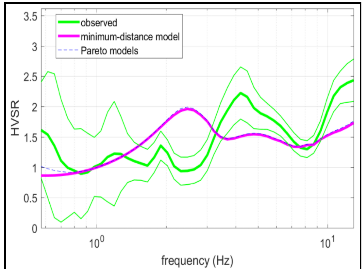
HVSR - CURVE H/V
