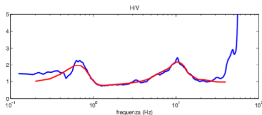
Figura 3.7 - In sinistra è riportato uno spettro H/V (curva di dispersione) in blu e la relativa curva di ellitticità elaborata prodotta dai log in V_s riportati sul grafico a destra. In questa figura indicati i successivi modelli iterativi in verde ed il log V_s finale in rosso.
