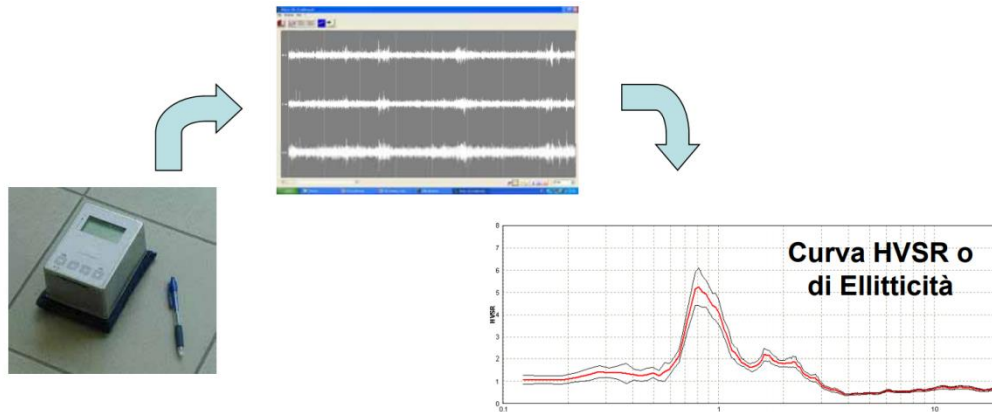
Figura 3.4 - Flow per la determinazione della curva di ellitticità
