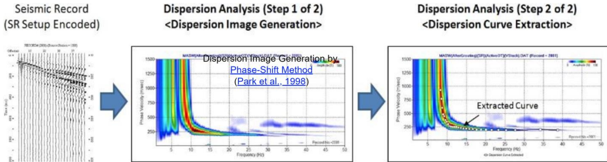
Figura 3.3 – Analisi MASW (sismogramma – Spectral analysis e curva di dispersione – Picking).
