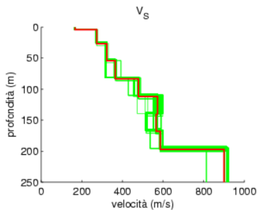
Figura 3.7 - In sinistra è riportato uno spettro H/V (curva di dispersione) in blu e la relativa curva di ellitticità elaborata prodotta dai log in V_s riportati sul grafico a destra. In questa figura indicati i successivi modelli iterativi in verde ed il log V_s finale in rosso.
