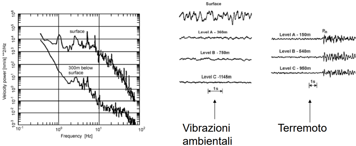
Figura 3.1 – Esempio di ampiezze di segnali acquisiti a profondità differenti.
