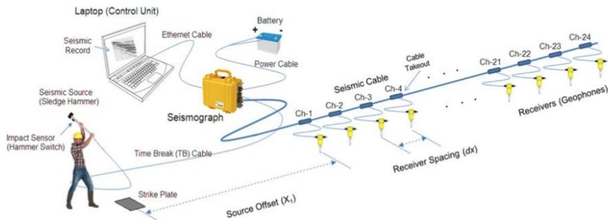
Figura 3.1 - Configurazione MASW
