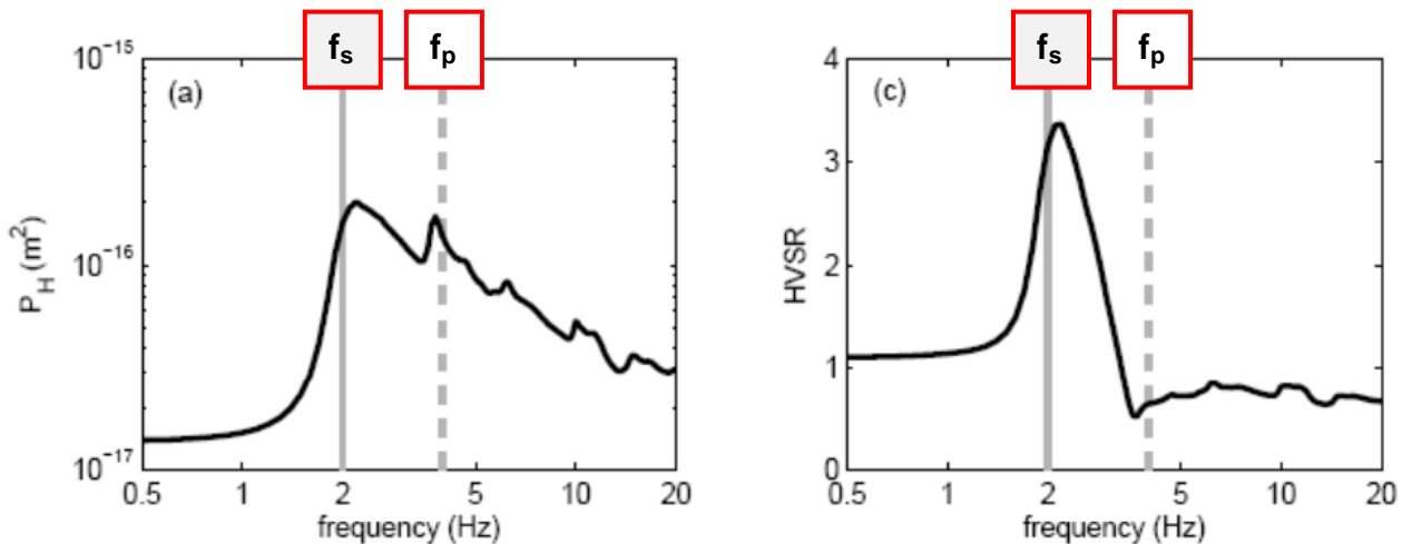
Figura 3.2 - Spettro di potenza (a sinistra) e HVSR (a destra) relativi alle onde di taglio e compressione
