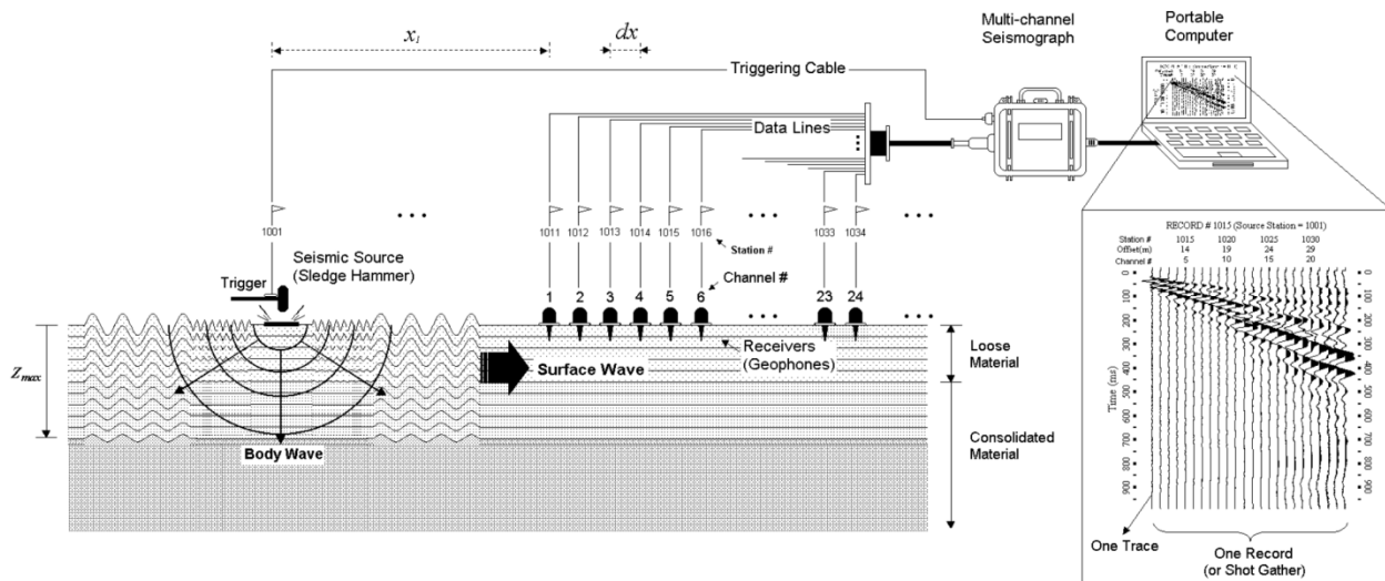
Figura 3.2. Tipica configurazione di campo per prova MASW
