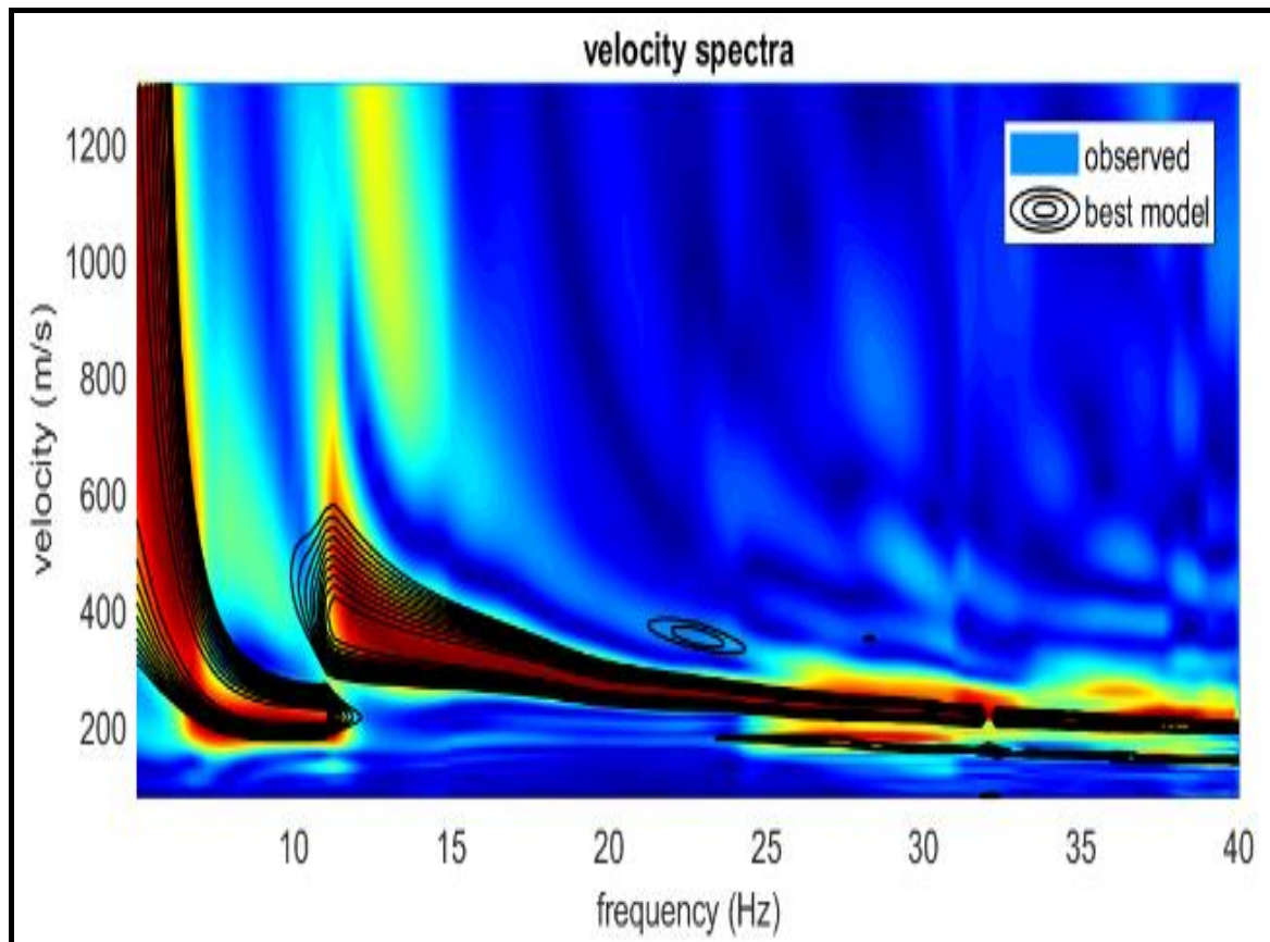
MASW - SPETTRO DI VELOCITA'
