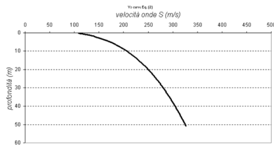
Figura 3.6 - Andamento delle V_s in profondità
