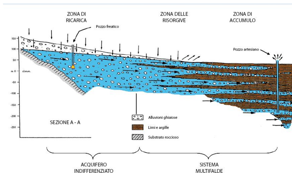
Figura 4-4: Schema idrogeologico e dell'interdigitazione dei sedimenti nella pianura veneto-friulana (da Dal Prà et al. 2000).
