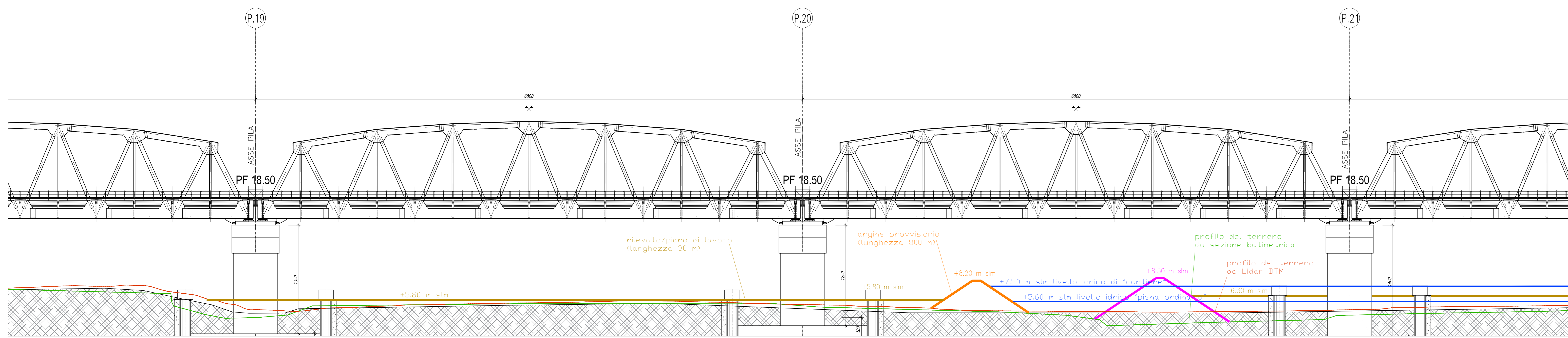
SEZIONE - FASE 2 Scala 1:200
